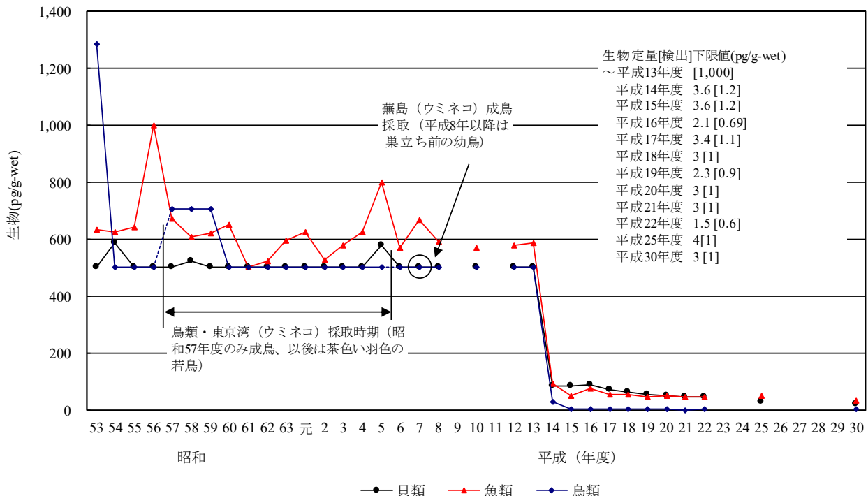
[6-5] o,p' -DDE
