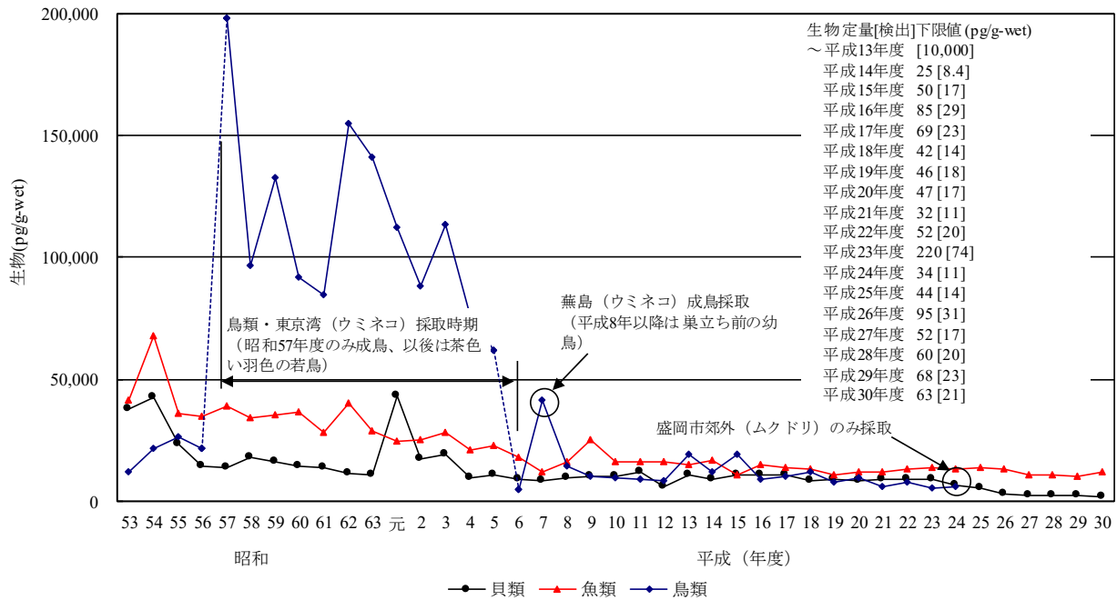
[1] PCB類
