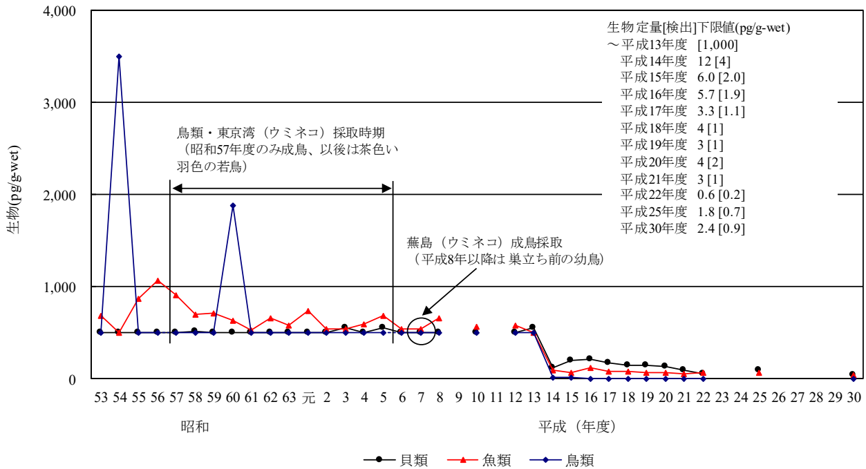
[6-6] o,p' -DDD
