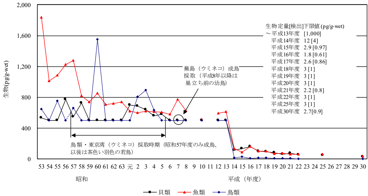
[6-4] o,p' -DDT
