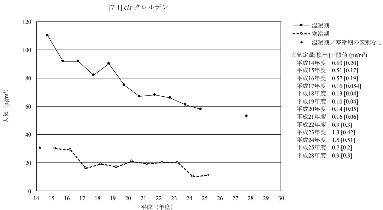
図 3-7-1-3 cis -クロルデンの生物の経年変化 (幾何平均値)
