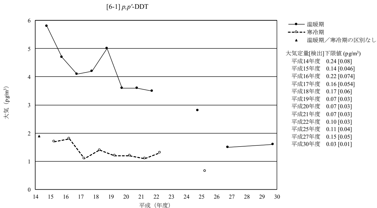
図 3-6-1-2 p,p' -DDT の大気の経年変化 (幾何平均値)
