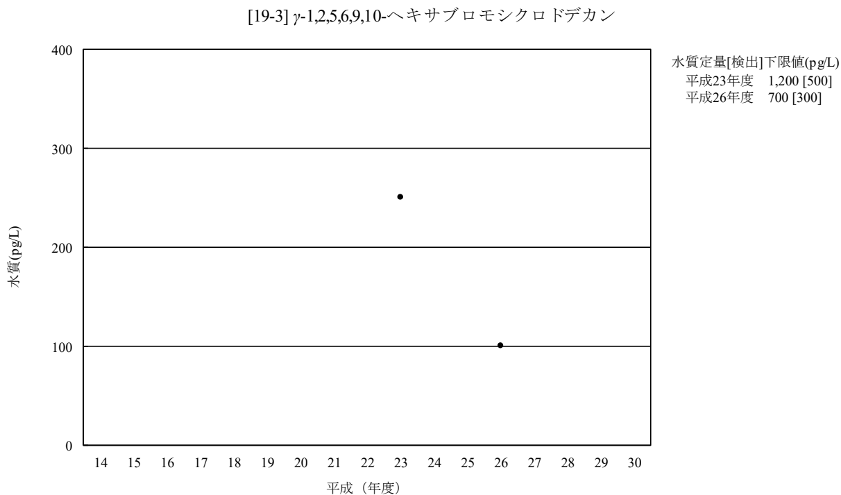
図 3-19-3-2 \gamma -1,2,5,6,9,10-ヘキサブロモシクロドデカンの水質の経年変化 (幾何平均値)
