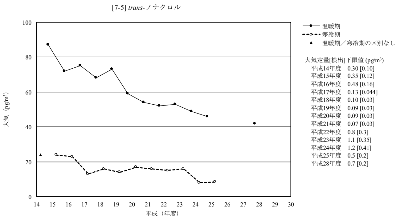
図 3-7-5-3 trans -ノナクロルの生物の経年変化(幾何平均値)
