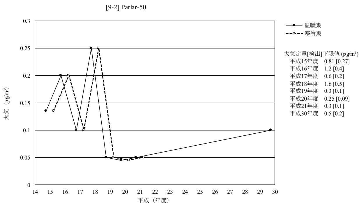
図 3-9-2-1 トキサフェン Parlar-50 の生物の経年変化 (幾何平均値)
