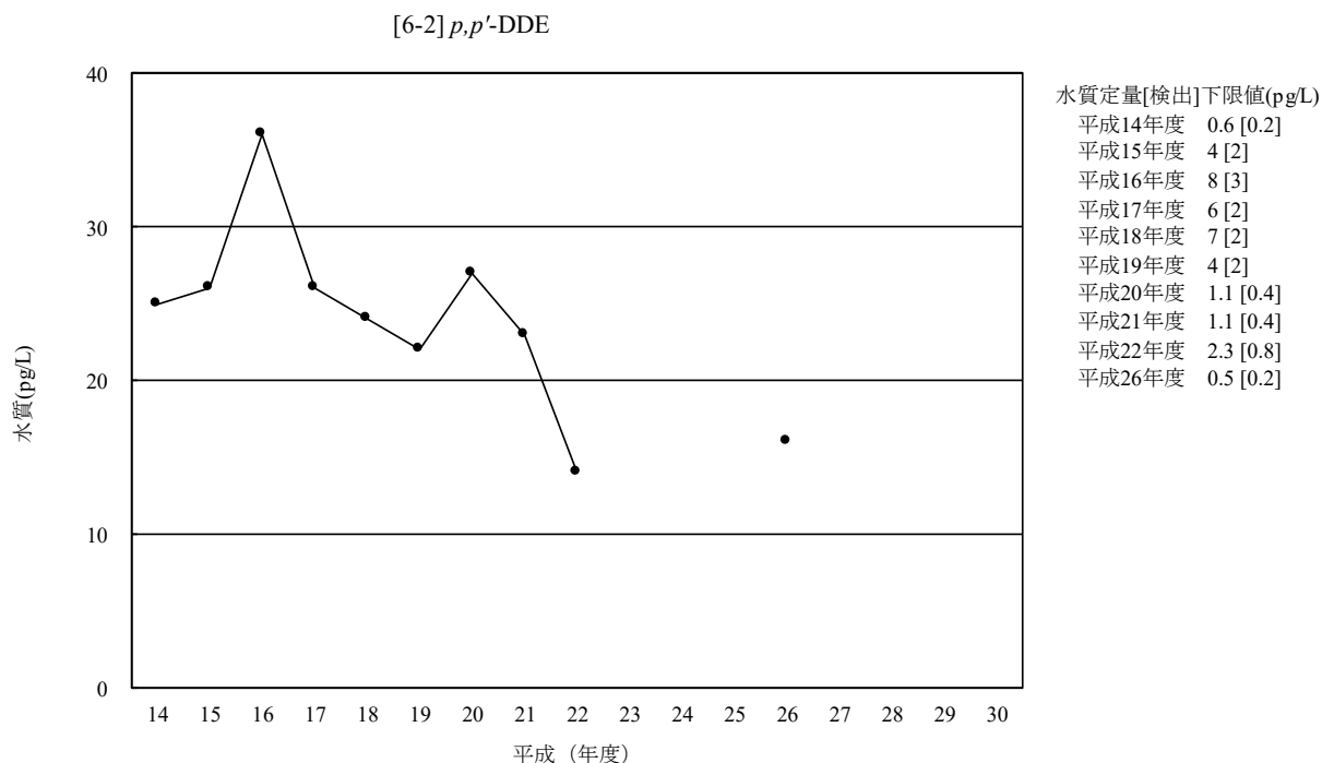
図 3-6-2-3 p,p' -DDE の水質の経年変化 (幾何平均値)
