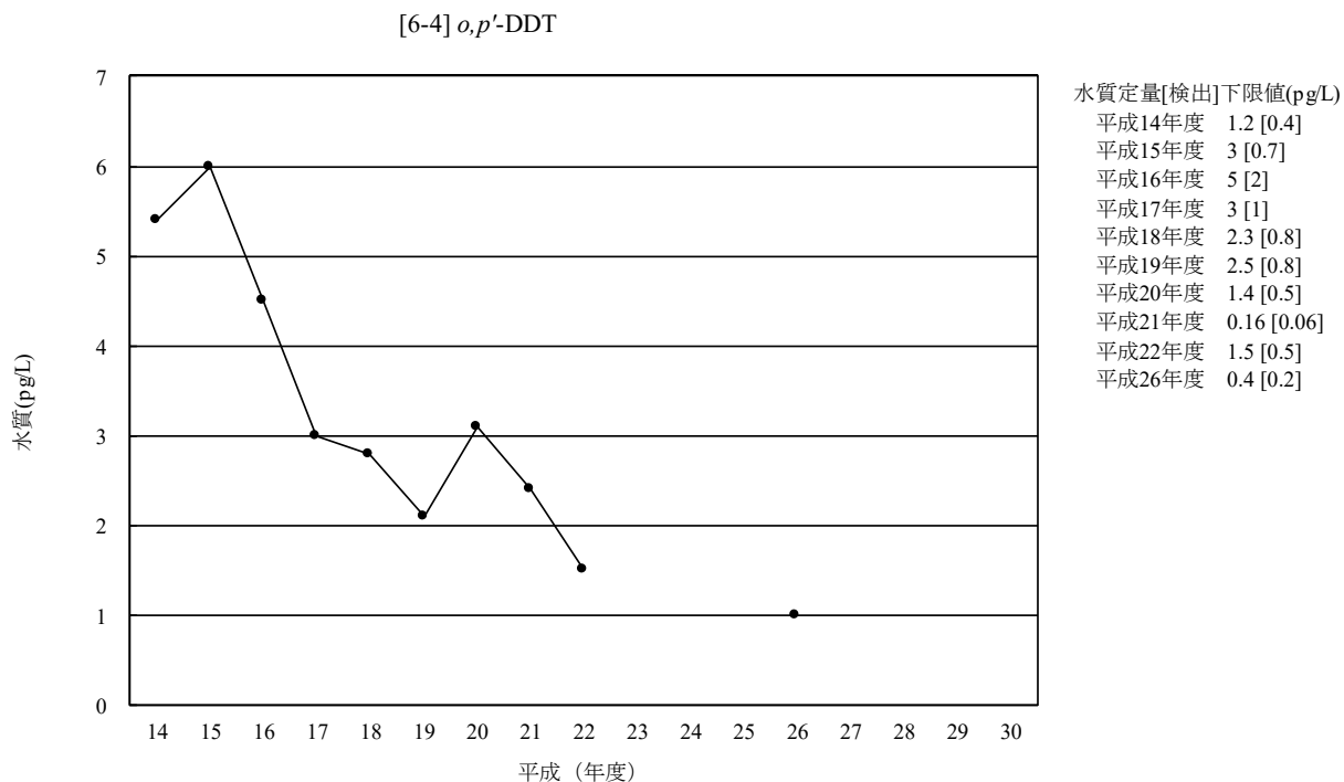
図 3-6-4-3 o,p' -DDT の水質の経年変化 (幾何平均値)
