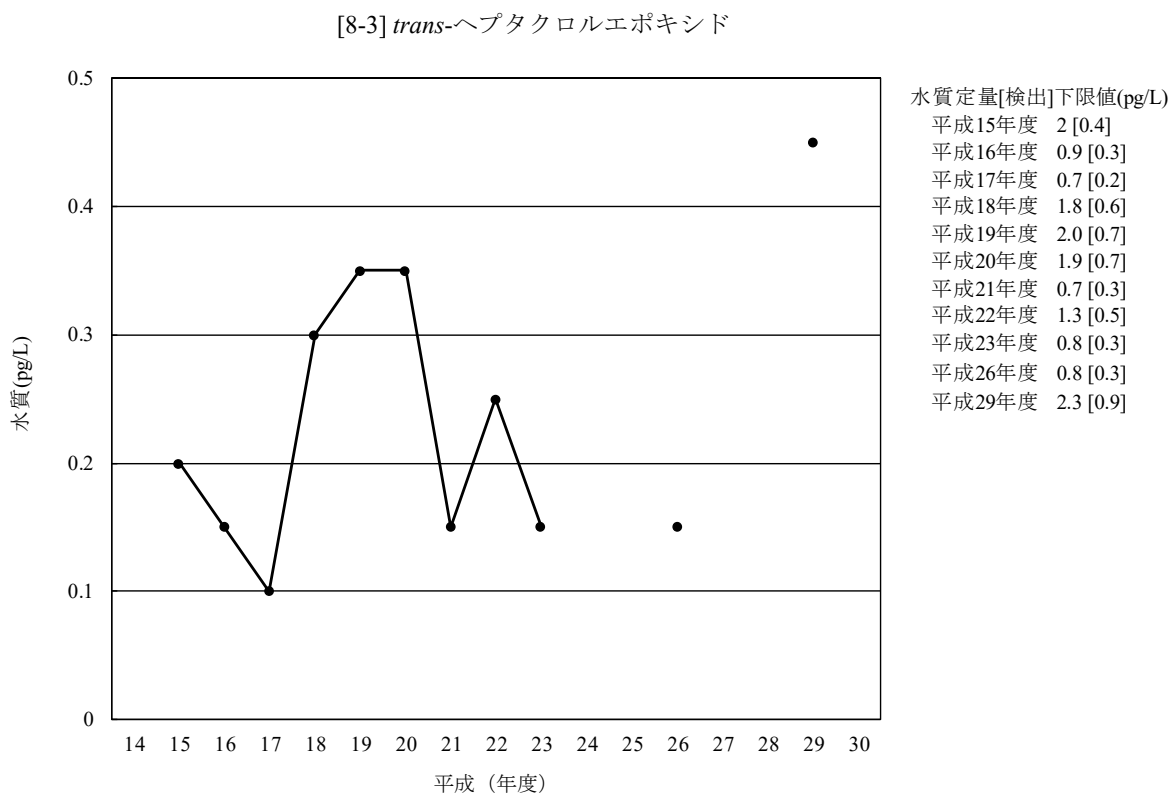
図 3-8-3-1 trans -ヘプタクロルエポキシドの水質の経年変化 (幾何平均値)
