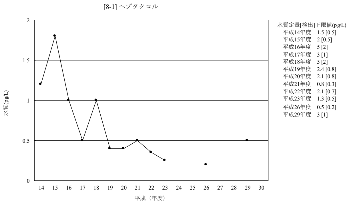
図 3-8-1-1 ヘプタクロルの水質の経年変化 (幾何平均値)
