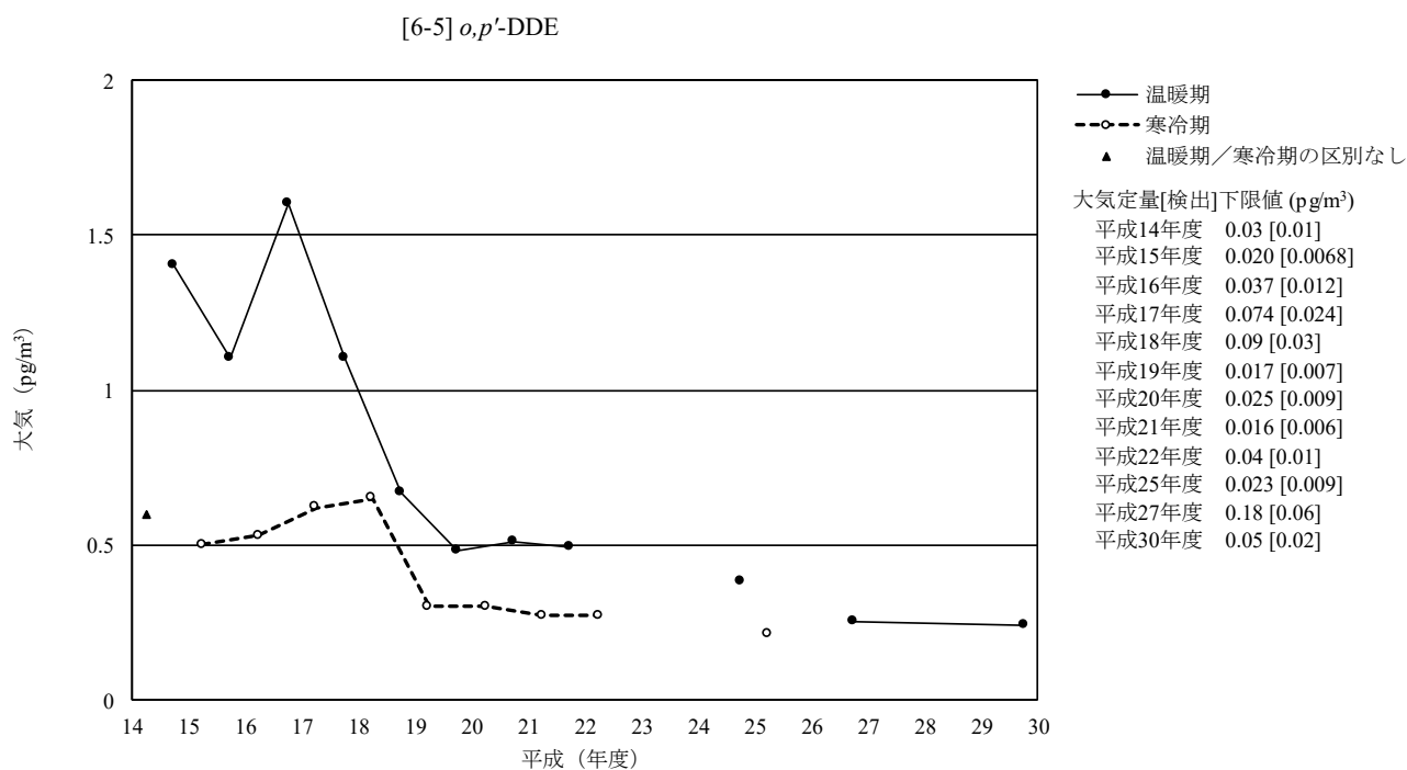
図 3-6-5-2 o,p' -DDE の大気の経年変化（幾何平均値）
