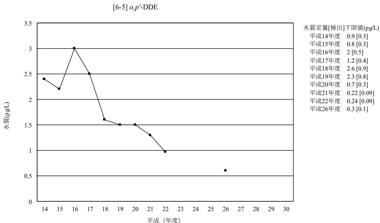
図 3-6-5-3 o,p' -DDE の水質の経年変化 (幾何平均値)
