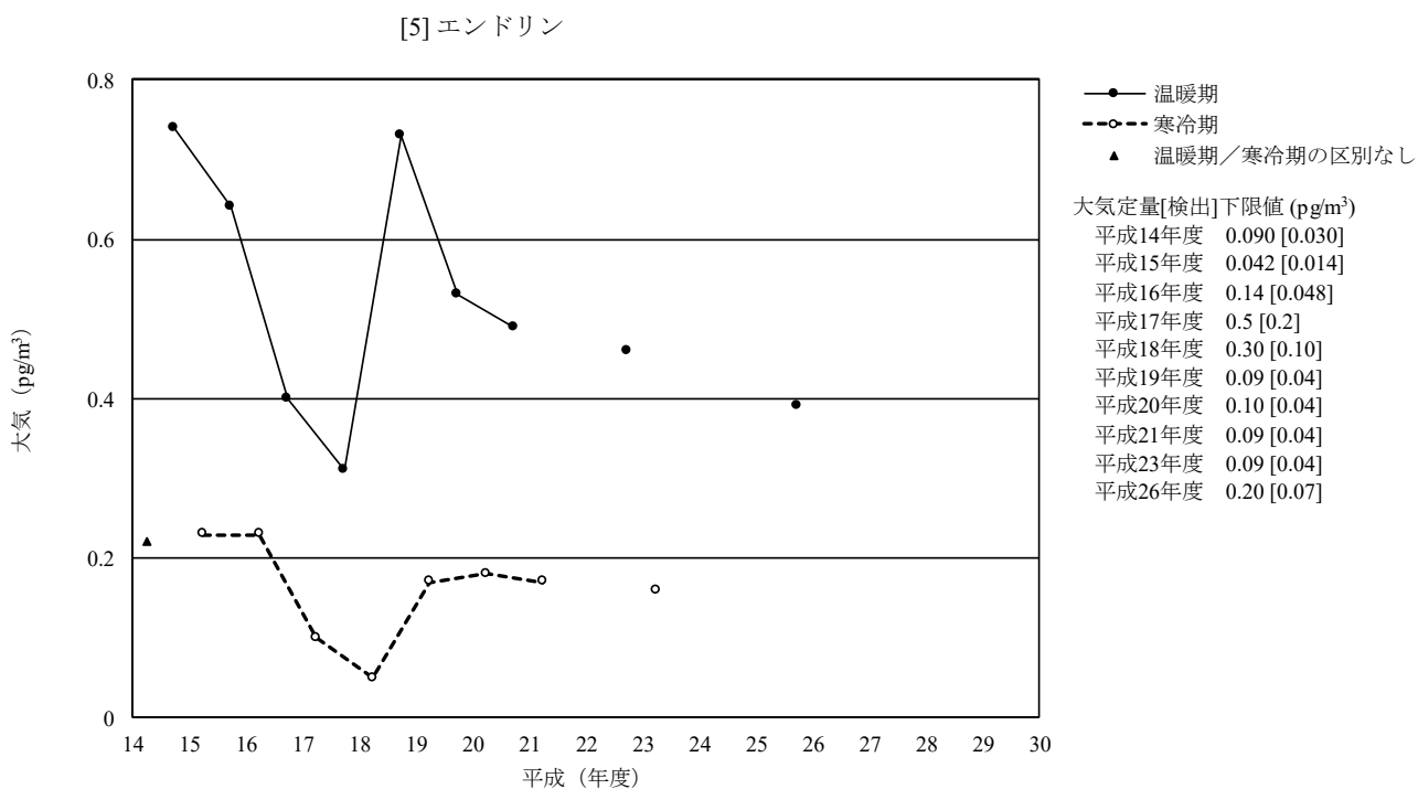
図 3-5-3 エンドリンの生物の経年変化 (幾何平均値)
