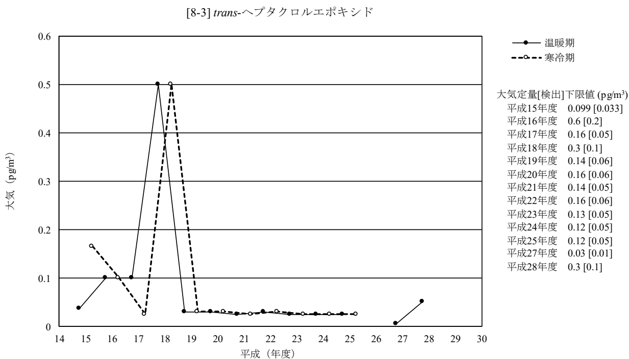
図 3-8-3-4 trans -ヘプタクロルエポキシドの大気の経年変化 (幾何平均値)
