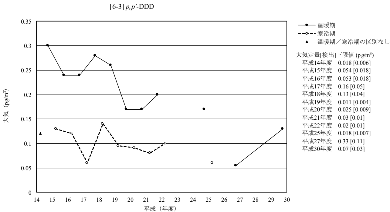
図 3-6-3-2 p,p' -DDD の大気の経年変化 (幾何平均値)
