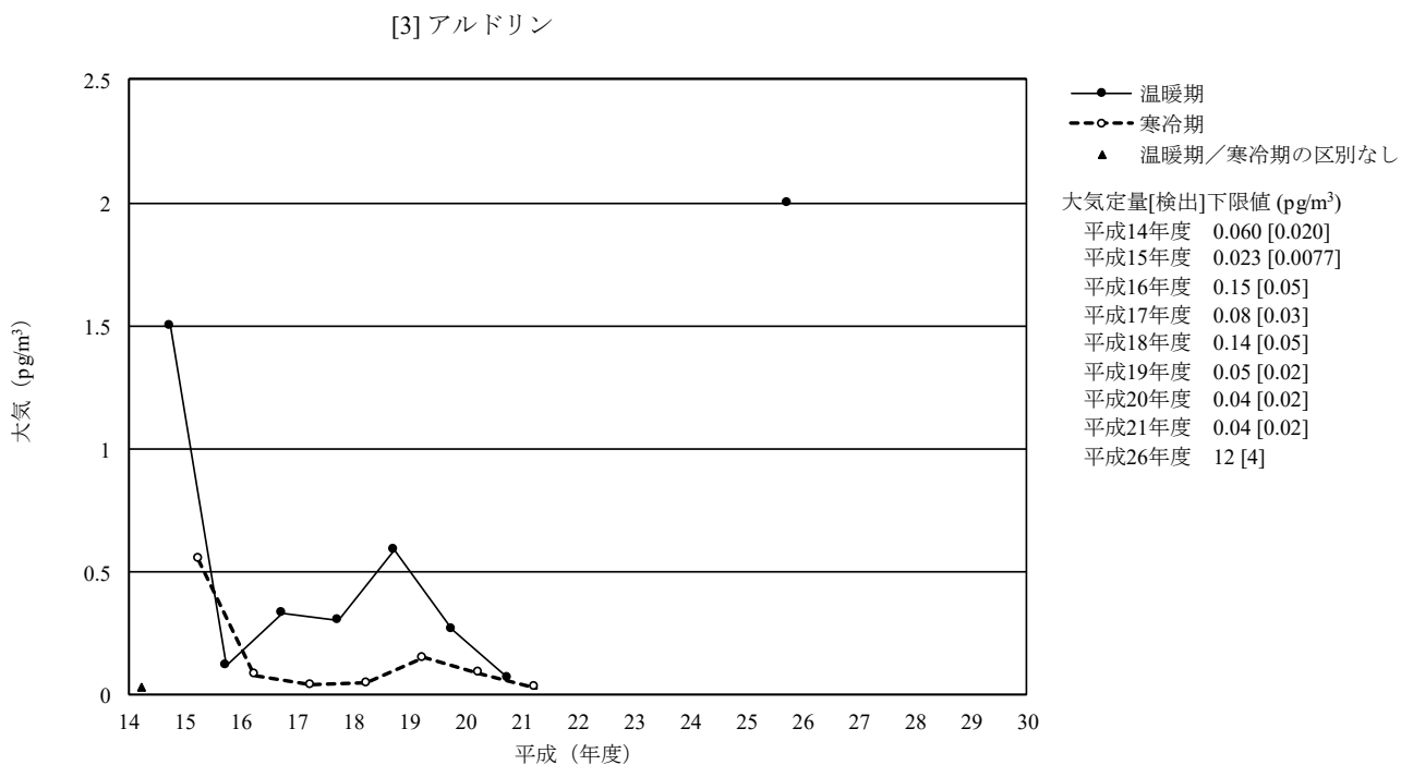
図 3-3-3 アルドリンの生物の経年変化（幾何平均値）（参考）
