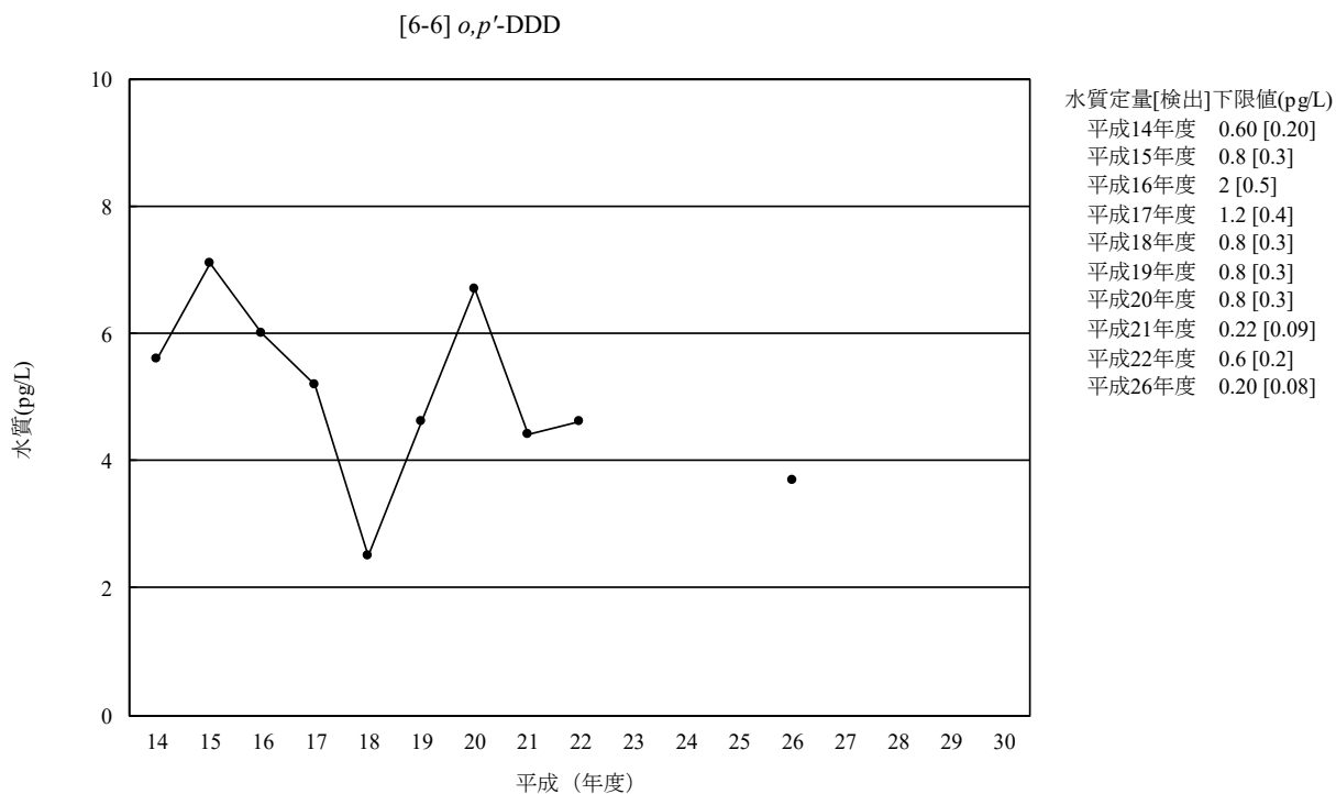
図 3-6-6-3 o,p' -DDD の水質の経年変化 (幾何平均値)
