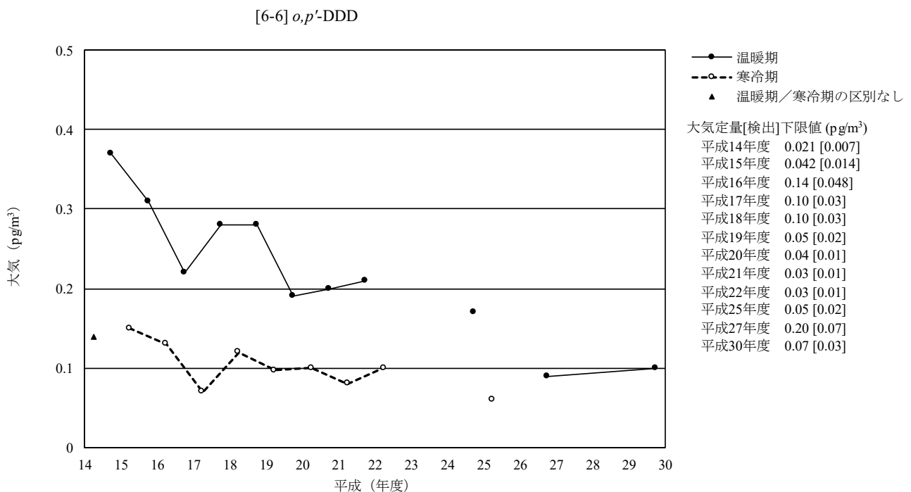
図 3-6-6-2 o,p' -DDD の大気の経年変化 (幾何平均値)
