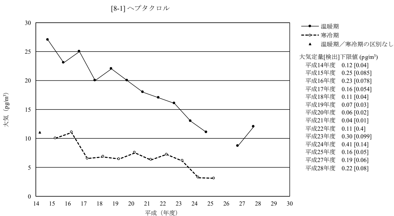
図 3-8-1-4 ヘプタクロルの大気の経年変化 (幾何平均値)
