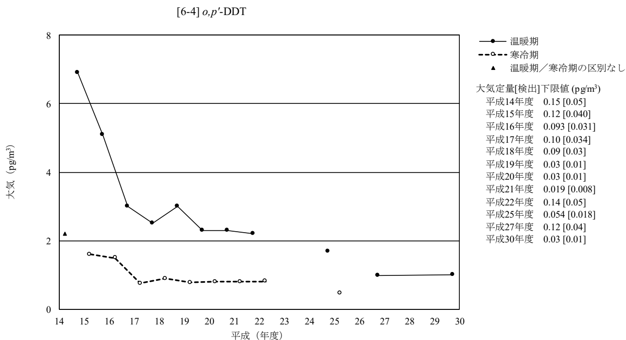
図 3-6-4-2 o,p' -DDT の大気の経年変化 (幾何平均値)
