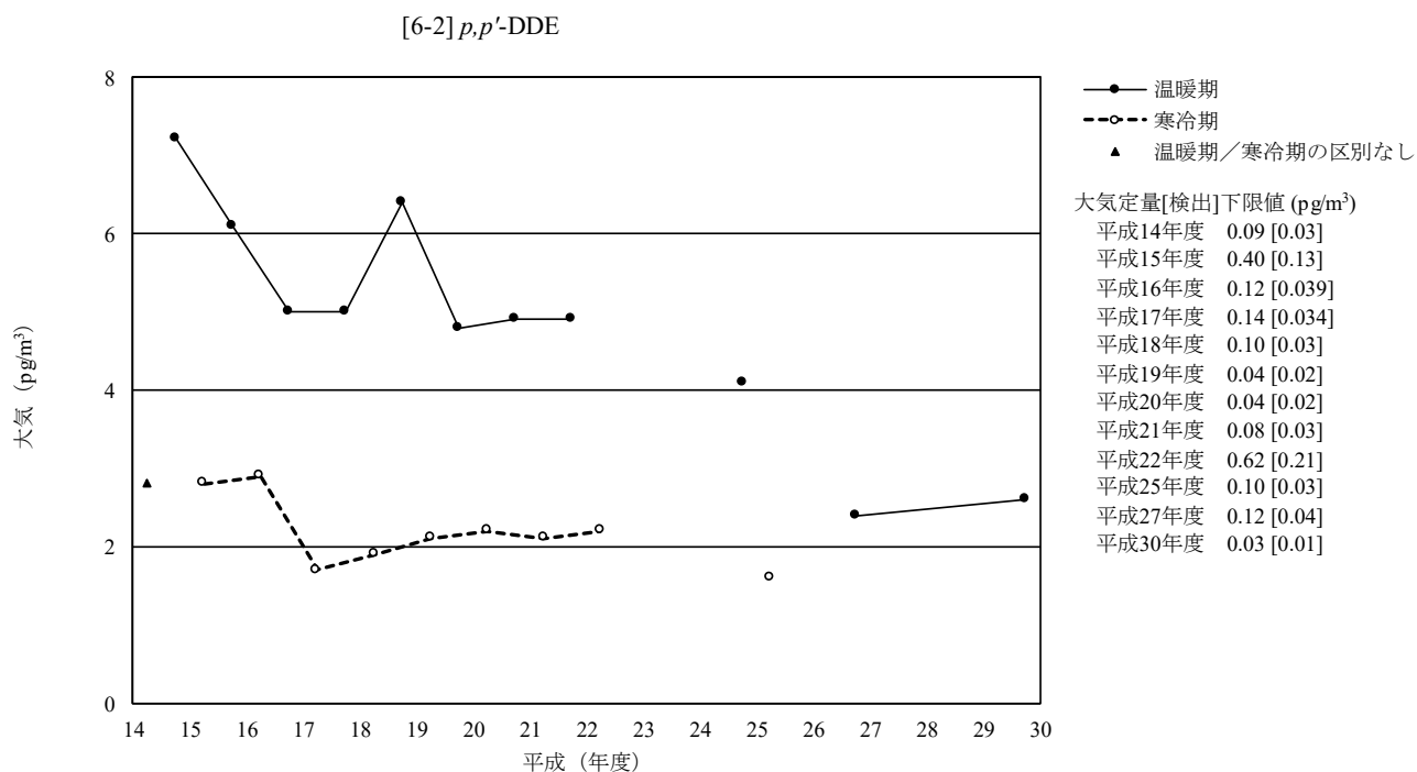
図 3-6-2-2 p,p' -DDE の大気の経年変化 (幾何平均値)
