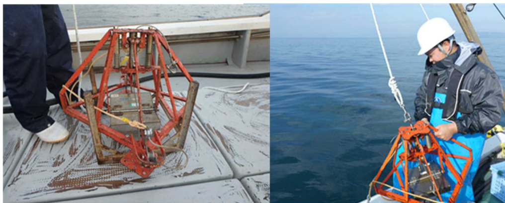
(1) スミスマッキンタイヤ型採泥器
