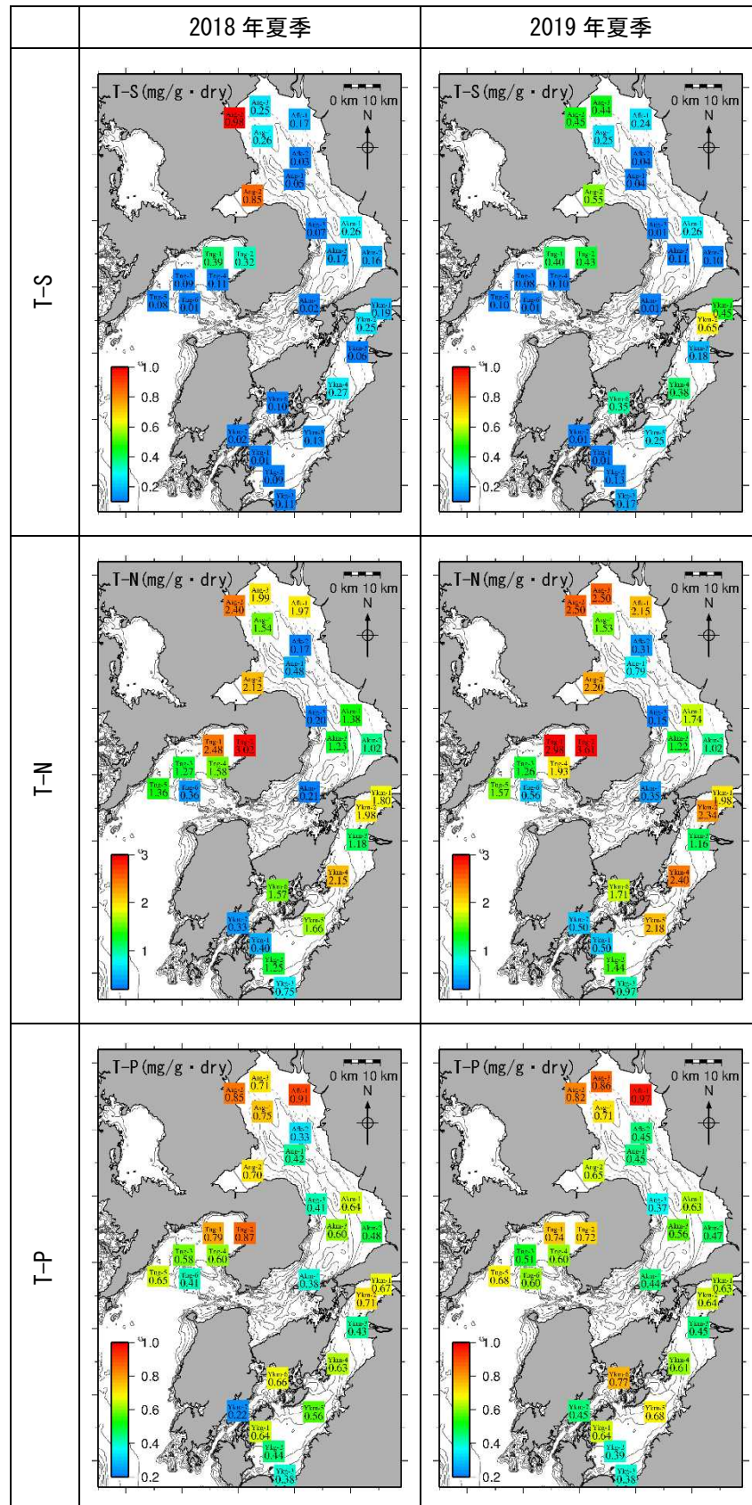
図 7 (3) 平面分布の変化(T-S、T-N、T-P)
