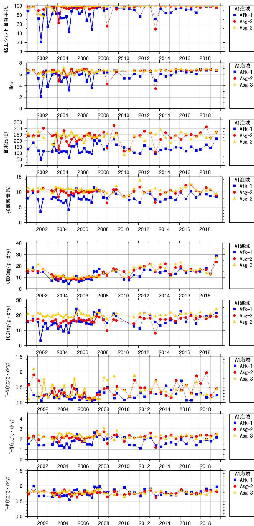
図 8 (1) 底質の変動(経年変化)(Afk-1、Asg-2、Asg-3)
