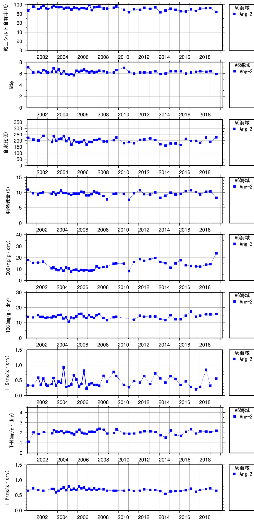
図 8 (6) 底質の変動(経年変化)(Ang-2)
