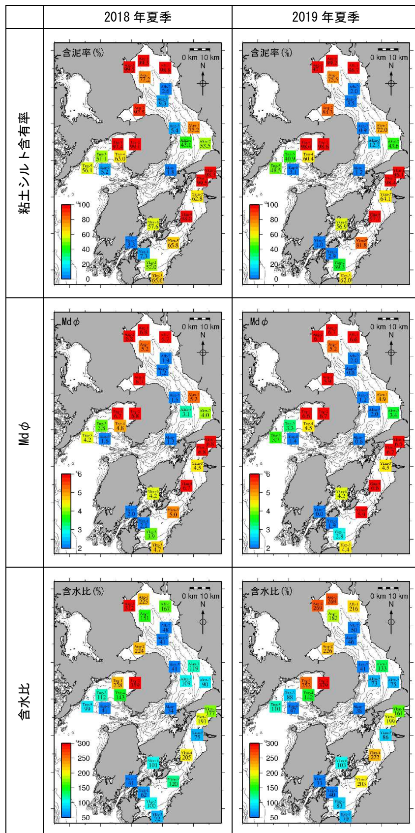
図 7 (1) 平面分布の変化(粘土シルト含有率、Md \phi 、含水比)
