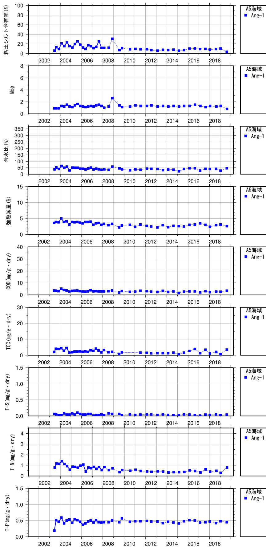
図 8 (5) 底質の変動(経年変化)(Ang-1)
