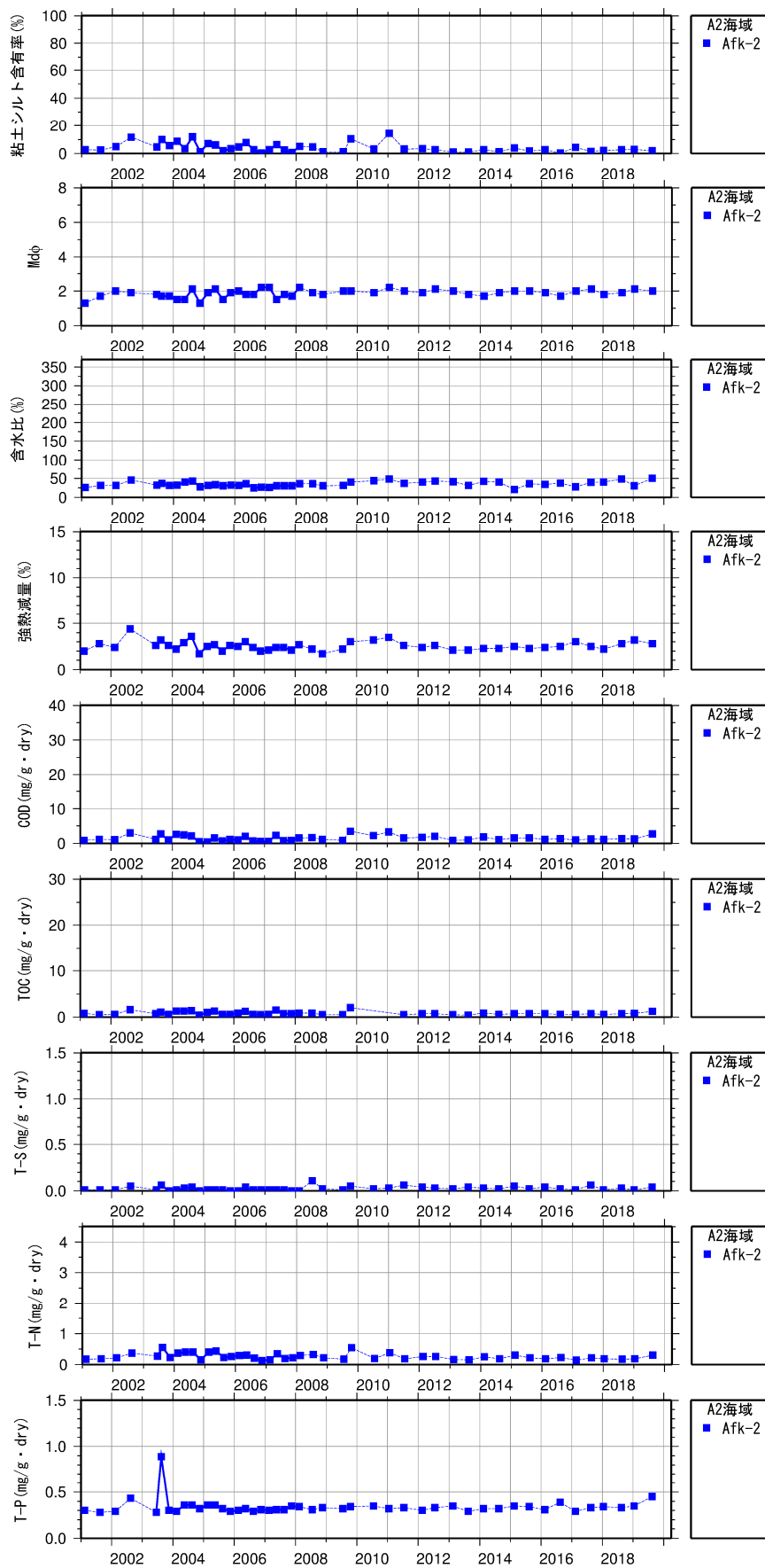
図 8 (2) 底質の変動(経年変化)(Afk-2)
