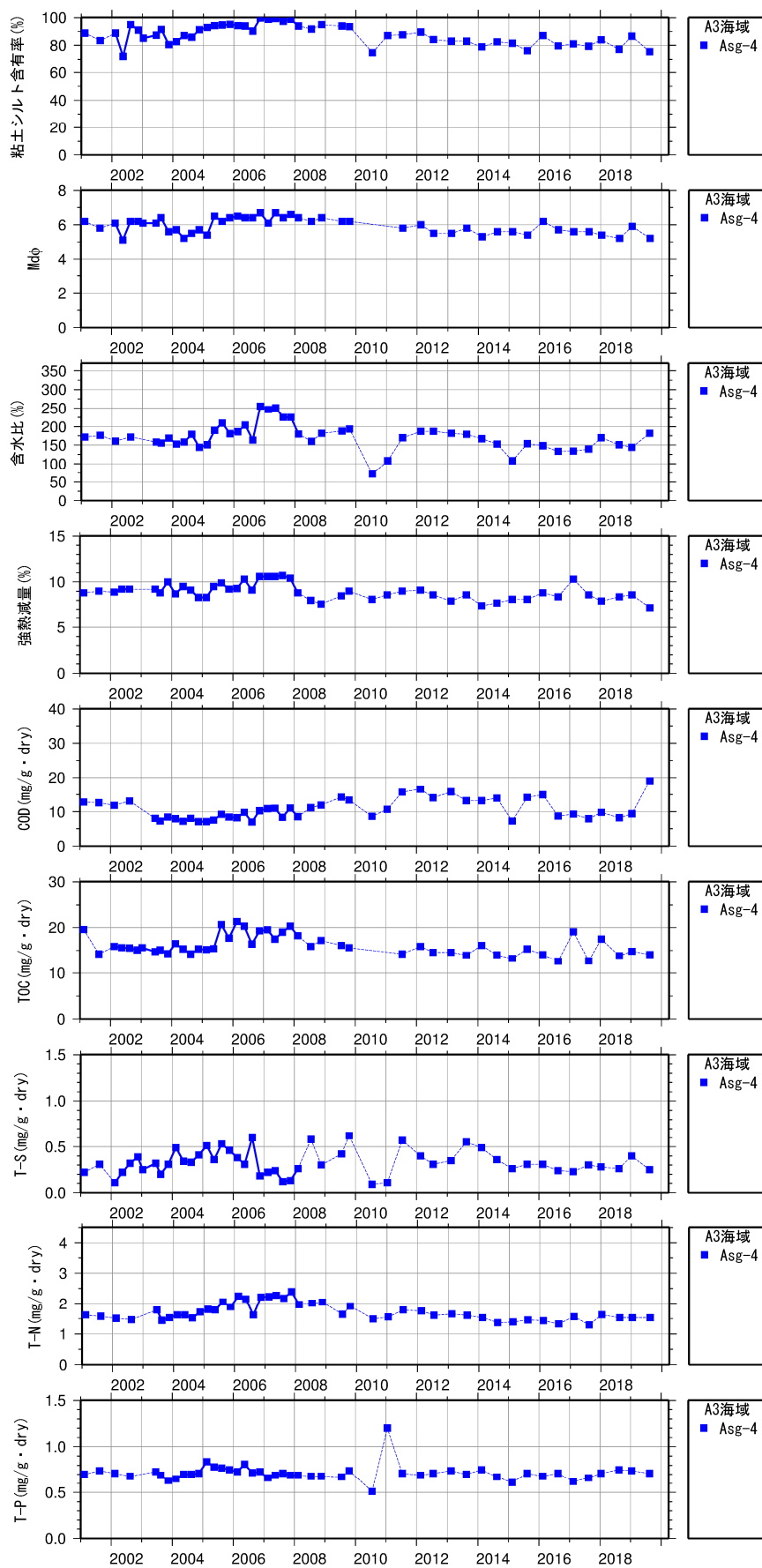
図 8 (3) 底質の変動(経年変化)(A3g-4)
