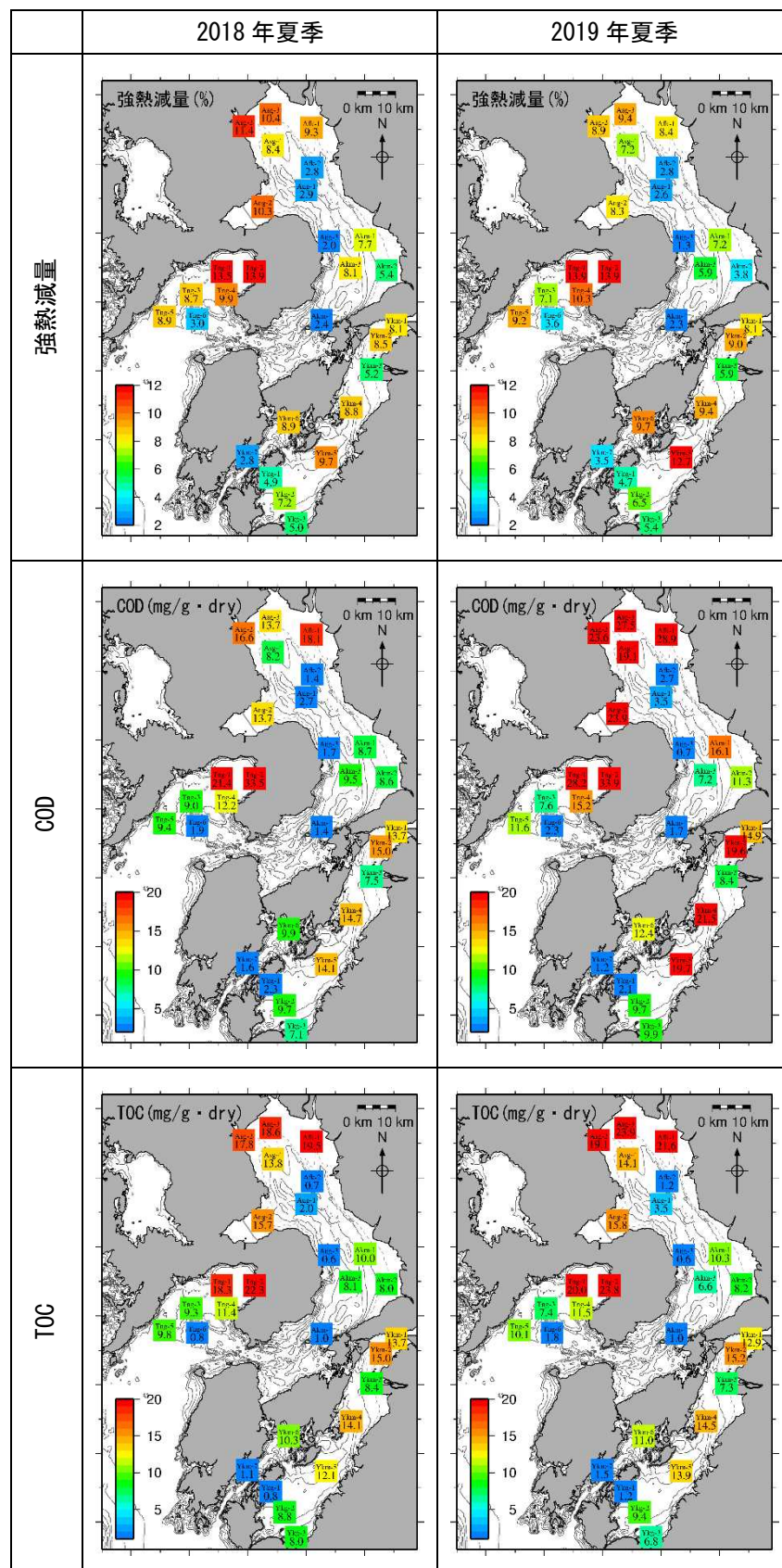
図 7 (2) 平面分布の変化(強熱減量、COD、TOC)
