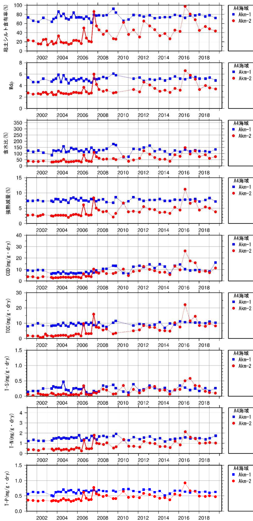
図 8 (4) 底質の変動(経年変化)(Akm-1、Akm-2)
