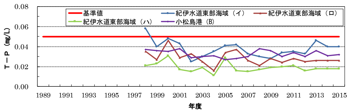
図 2-17 紀伊水道における TP の年度平均値の推移
