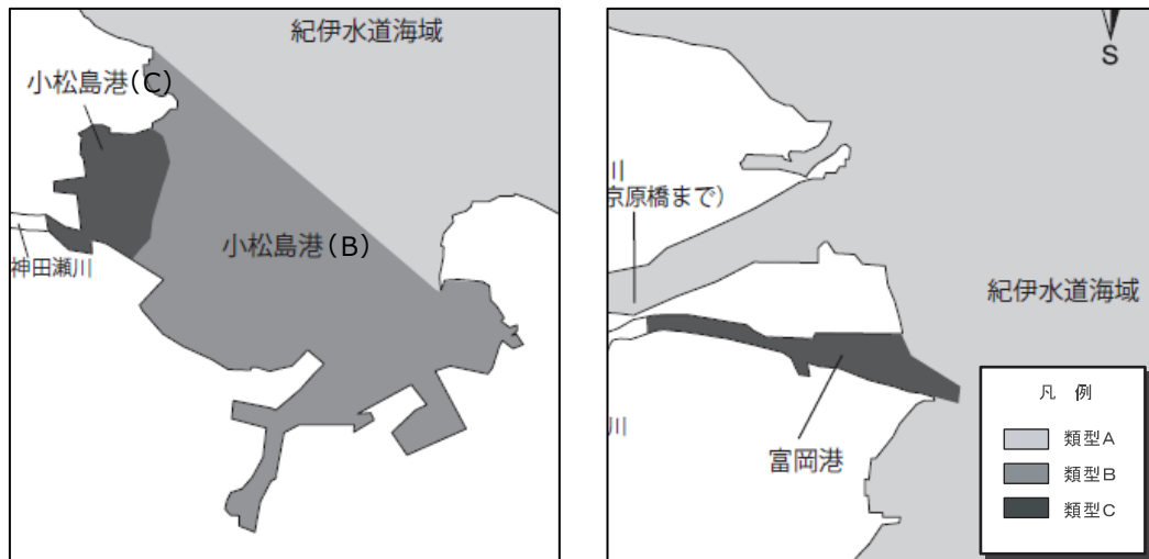
図 2-13(3) 紀伊水道における COD の類型指定(徳島県)
