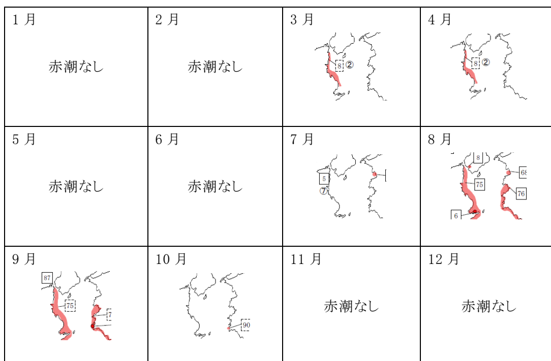
図 2-28 2013 年の紀伊水道における赤潮発生状況
