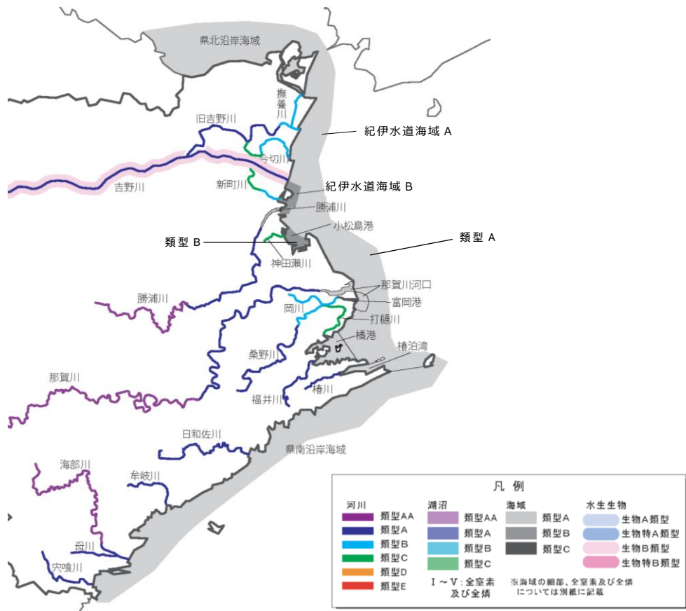
図 2-13(2) 紀伊水道における COD の類型指定(徳島県)
