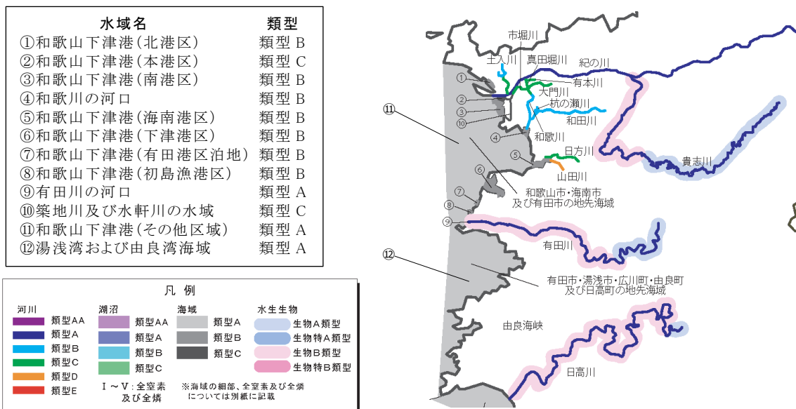
図 2-13(1) 紀伊水道における COD の類型指定(和歌山県)
