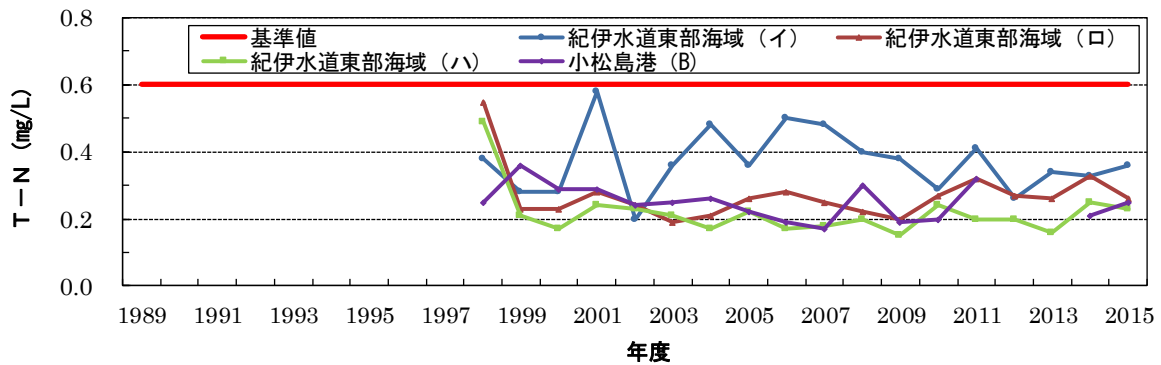
図 2-16 紀伊水道における TN の年度平均値の推移
