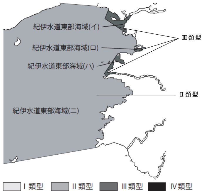
図 2-14(1) 紀伊水道における TN、TP の類型指定(和歌山県)
