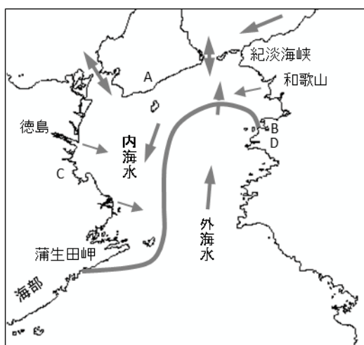
図 2-5 紀伊水道の水塊構造と流れ
