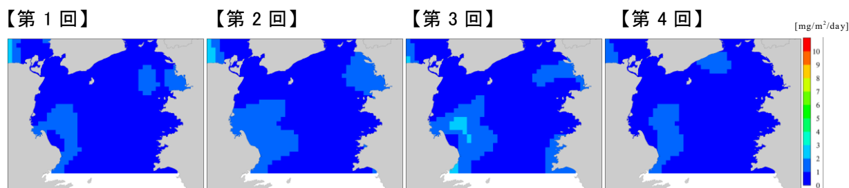
出典) 広域総合水質調査結果(環境省)、瀬戸内海環境情報基本調査結果(環境省)により算定 図 2-35 紀伊水道におけるりん溶出量(年平均値)の状況
