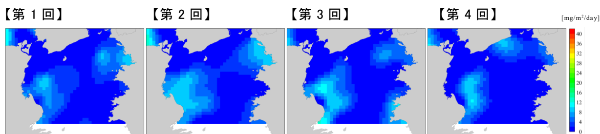
出典) 広域総合水質調査結果(環境省)、瀬戸内海環境情報基本調査結果(環境省)により算定 図 2-34 紀伊水道における窒素溶出量(年平均値)の状況
