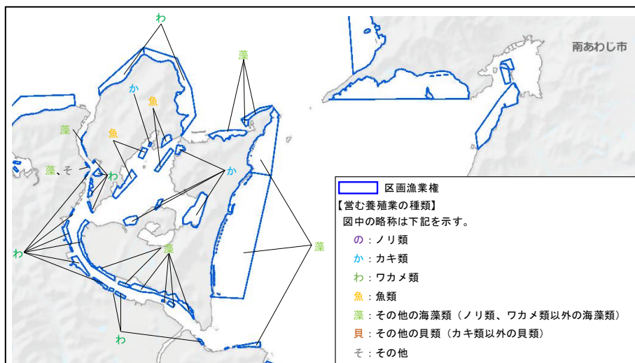
図 2-38 紀伊水道における区画漁業権の設定状況
