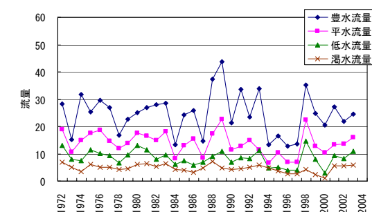
寄居流量観測地点の流況
