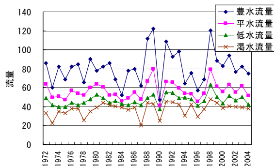
秋ヶ瀬取水堰の流況
