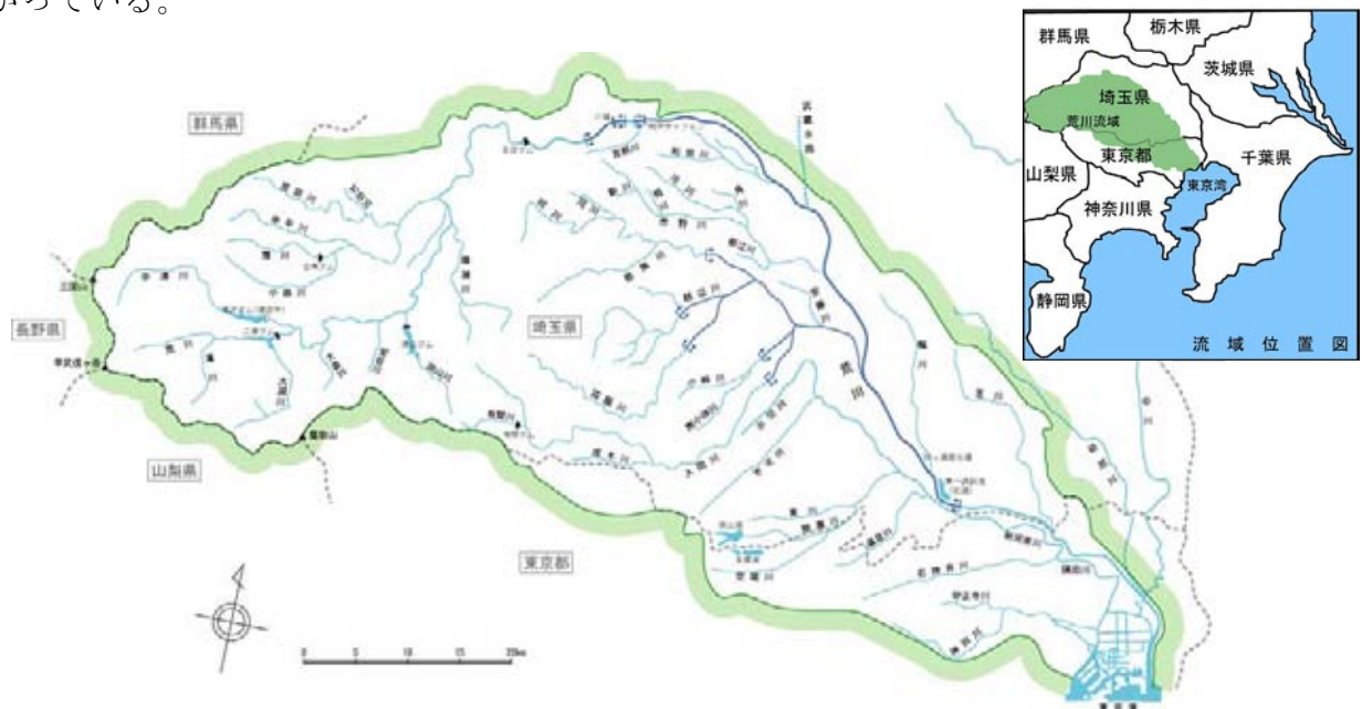
図 1-1 荒川流域図
