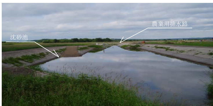
沈砂池写真（シロンド排水路）
