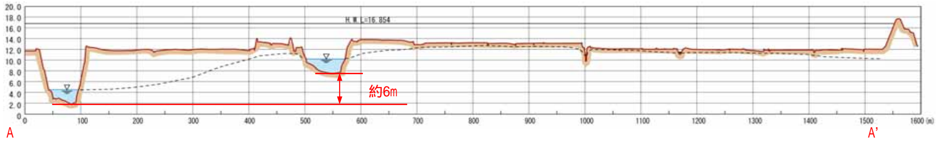
図2-6 横断面図 (52.0k)
