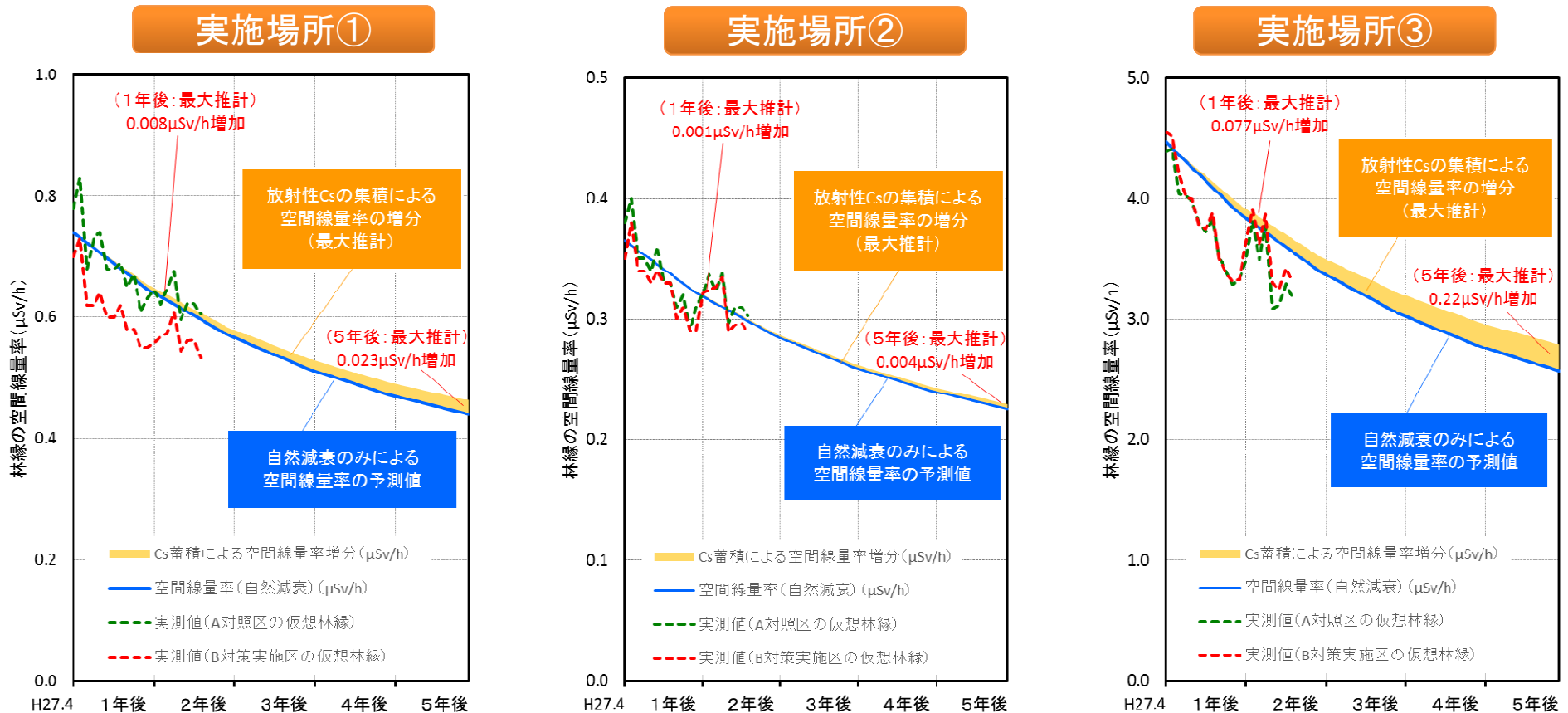
放射性Csの集積が林縁の空間線量率に及ぼす影響の推計 (降水量が非常に多かったH27年度と同じ状況が5年間継続した場合)
