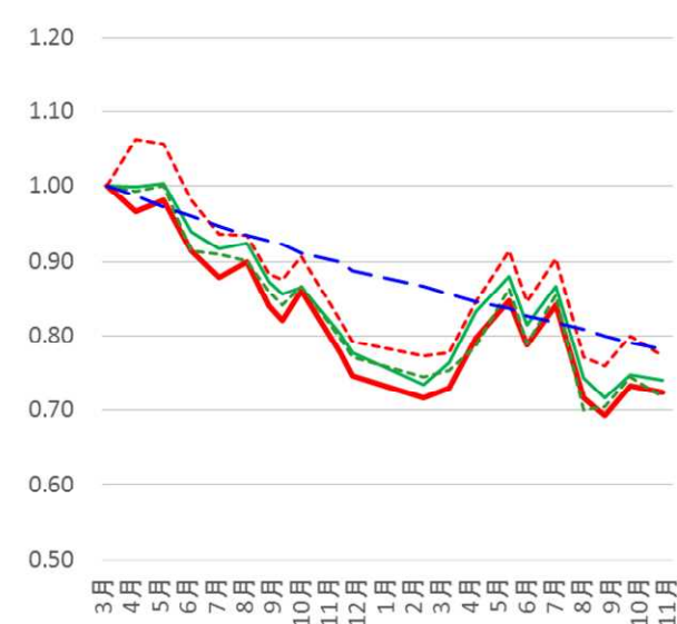
空間線量率推移の傾向 実施場所③ (計測開始月を1とする)
