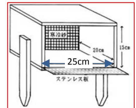
図2 土砂受け箱
