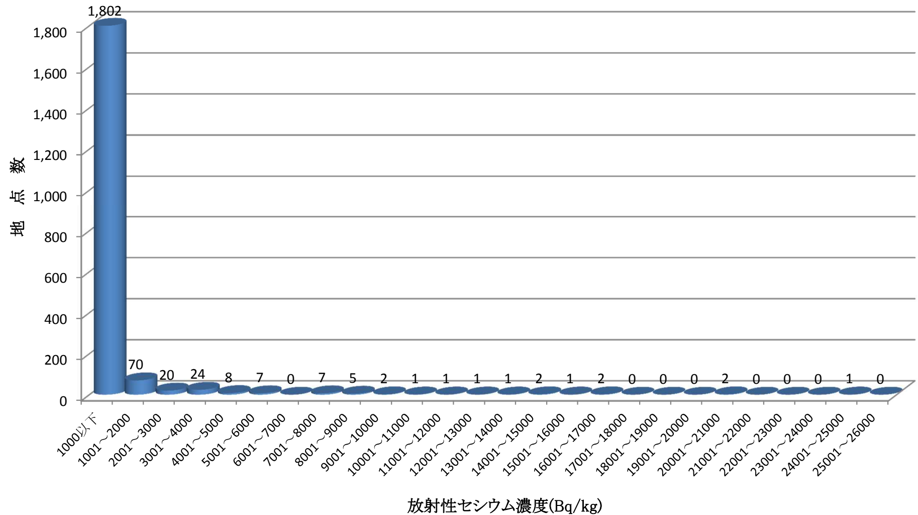
河川(底質)の放射性セシウム濃度ごと(1,000Bq/kg)の頻度(H26年度)
