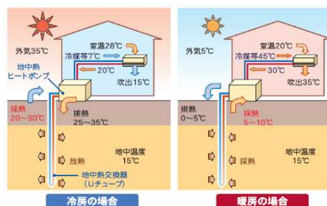
地中熱の冷暖房利用イメージ
