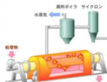
炭素繊維強化プラリサイクル設備
