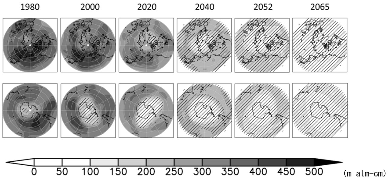
図 4-17 北半球中高緯度（上）および南半球中高緯度（下）のオゾン全量分布の経年変化
