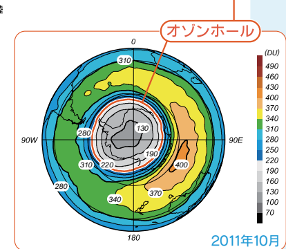
オゾンホールの年最大面積の経年変化（中央折れ線グラフ）と南半球の10月の月平均オゾン量の分布（左右図） データ提供：気象庁
