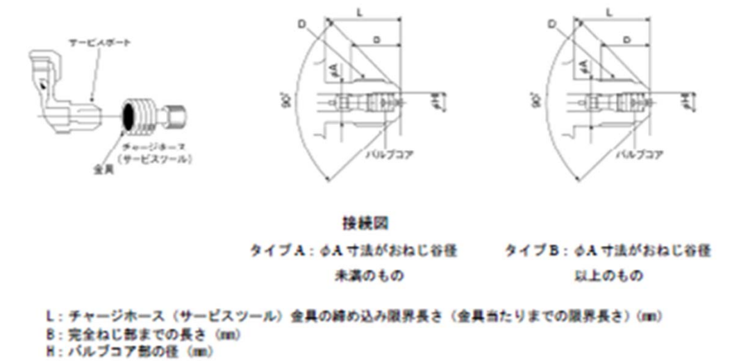
図 1-サービスポートのねじ部寸法
