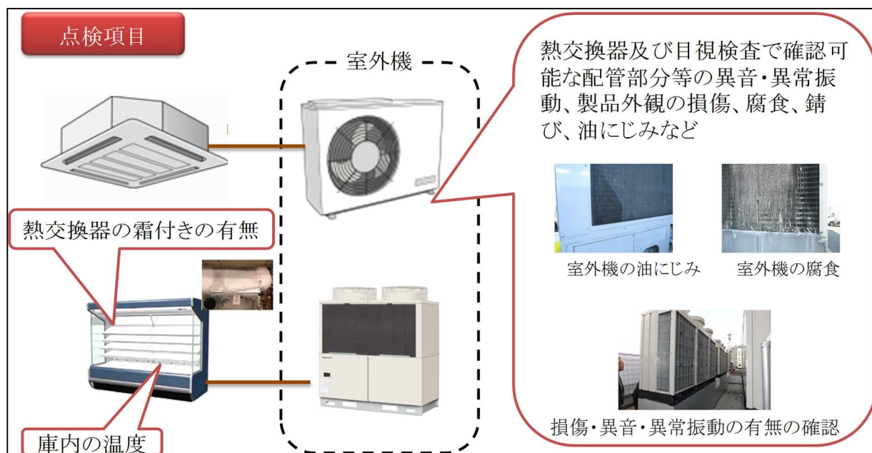
図 4 簡易点検時の点検箇所为例
