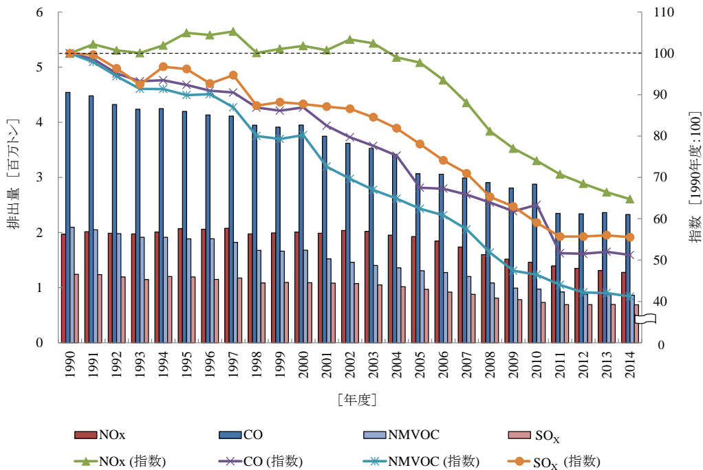
図 3 前駆物質及び硫黄酸化物の排出量の推移
