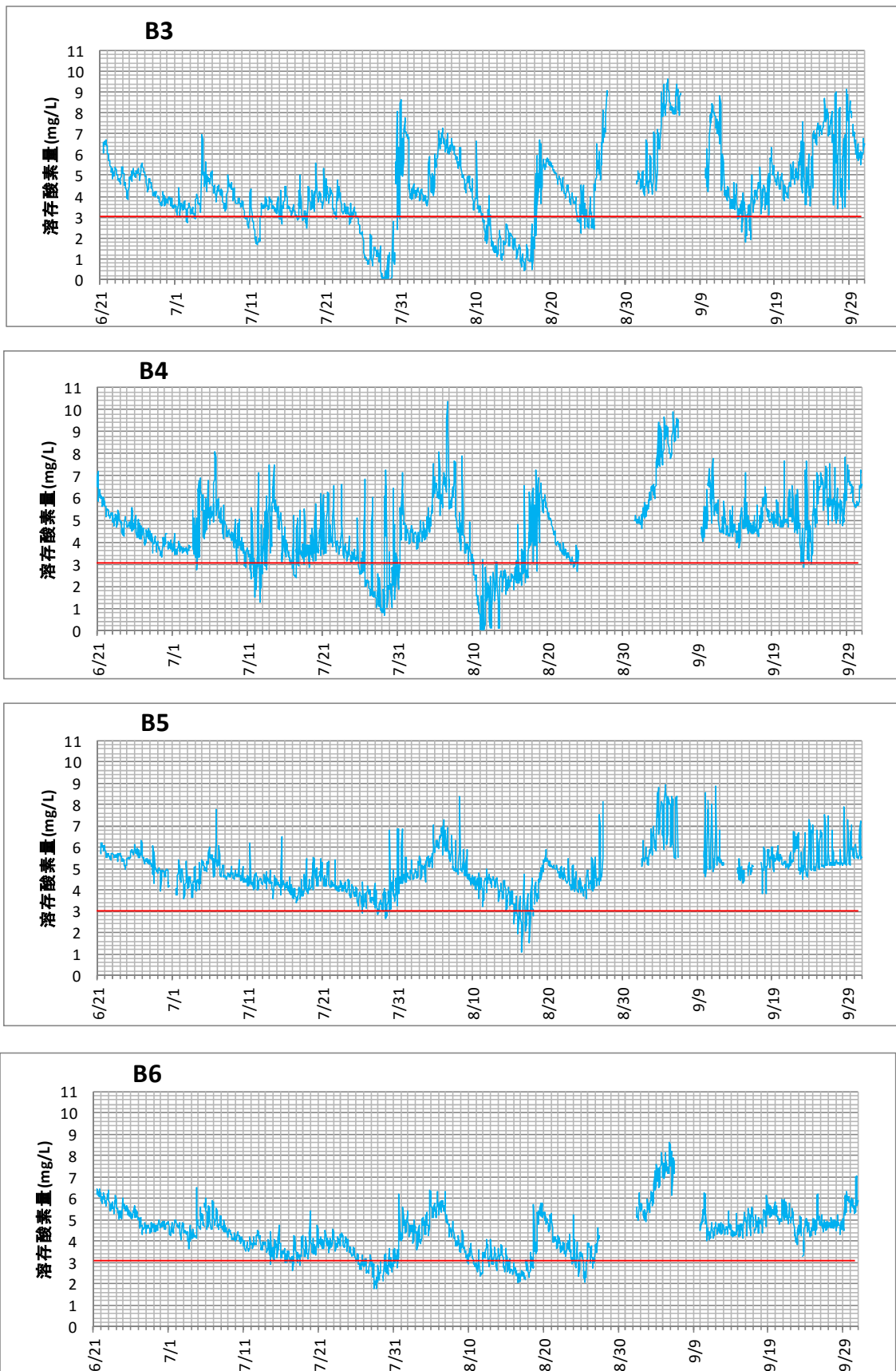
図 19(2) 底層DOの連続測定結果（その1）（2004 年、海底上1m）
