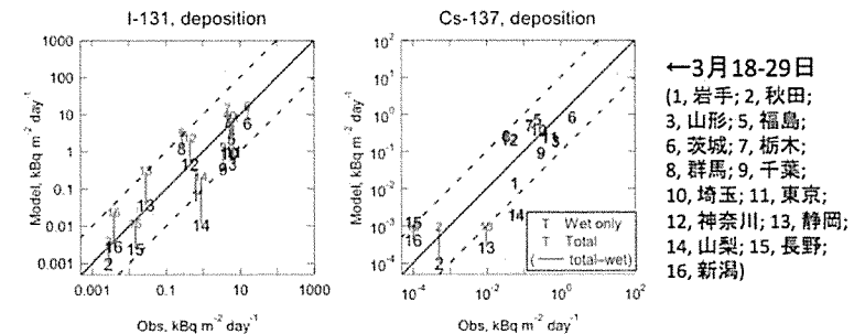
図 A3-2. 沈着量に対するモデルと観測 (文部科学省・定時降下物のモニタリング) の比較結果 (Morino et al., 2011)。
