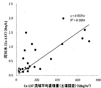
図 A3-4. 流域平均沈着量と河川水のセシウム 137 濃度の関係
