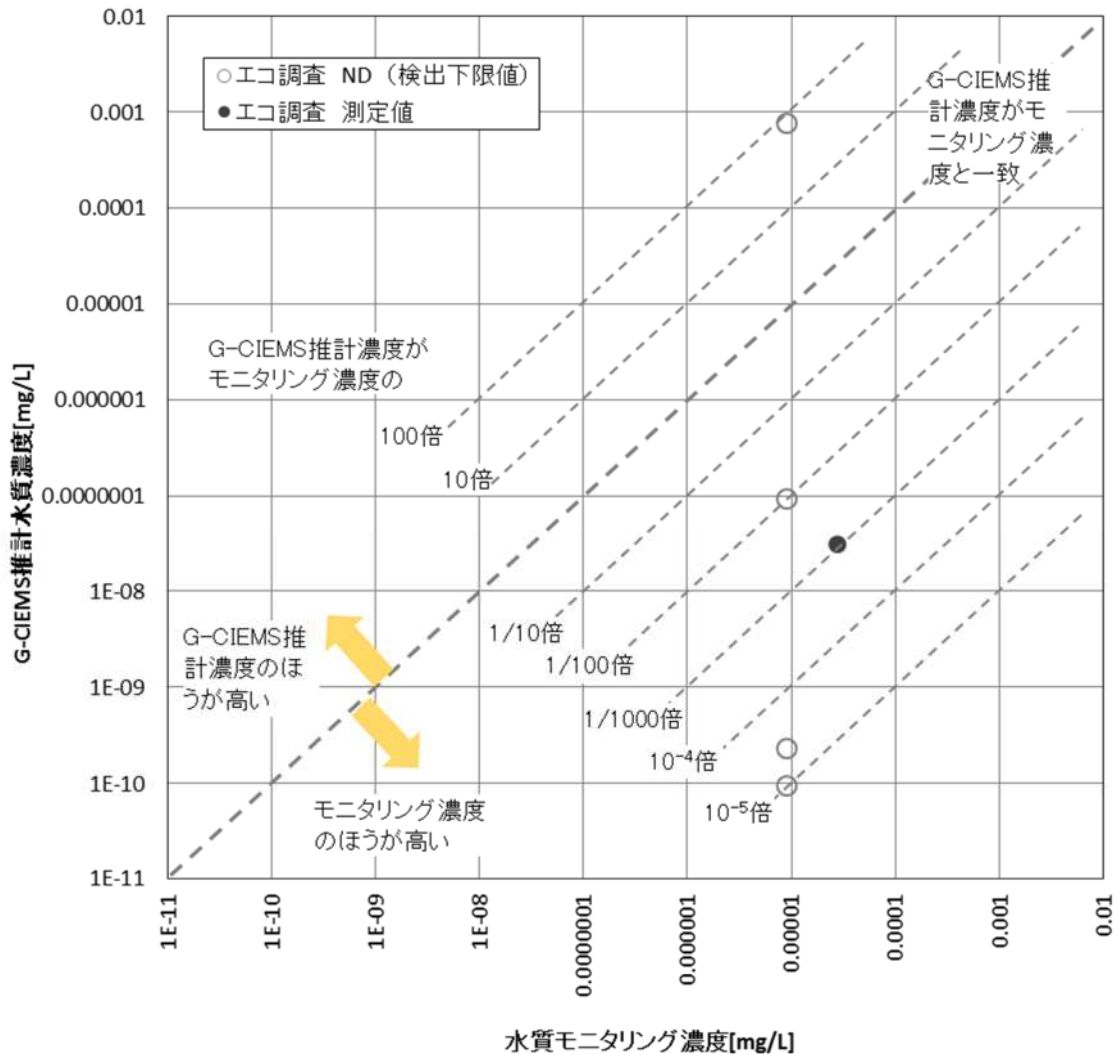
10 図 7-1 評価対象地点における G-CIEMS 推計水質濃度とモニタリング水質濃度の比較 11 (エコ調査(平成 24 年度))
