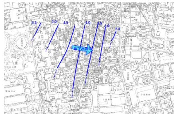
地下水コンター図 (平成 20 年 8 月:夏季)
