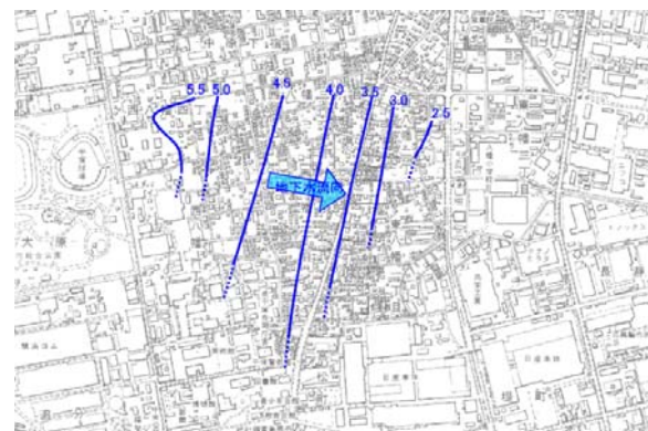
地下水コンター図 (平成 20 年 11 月:秋季)
