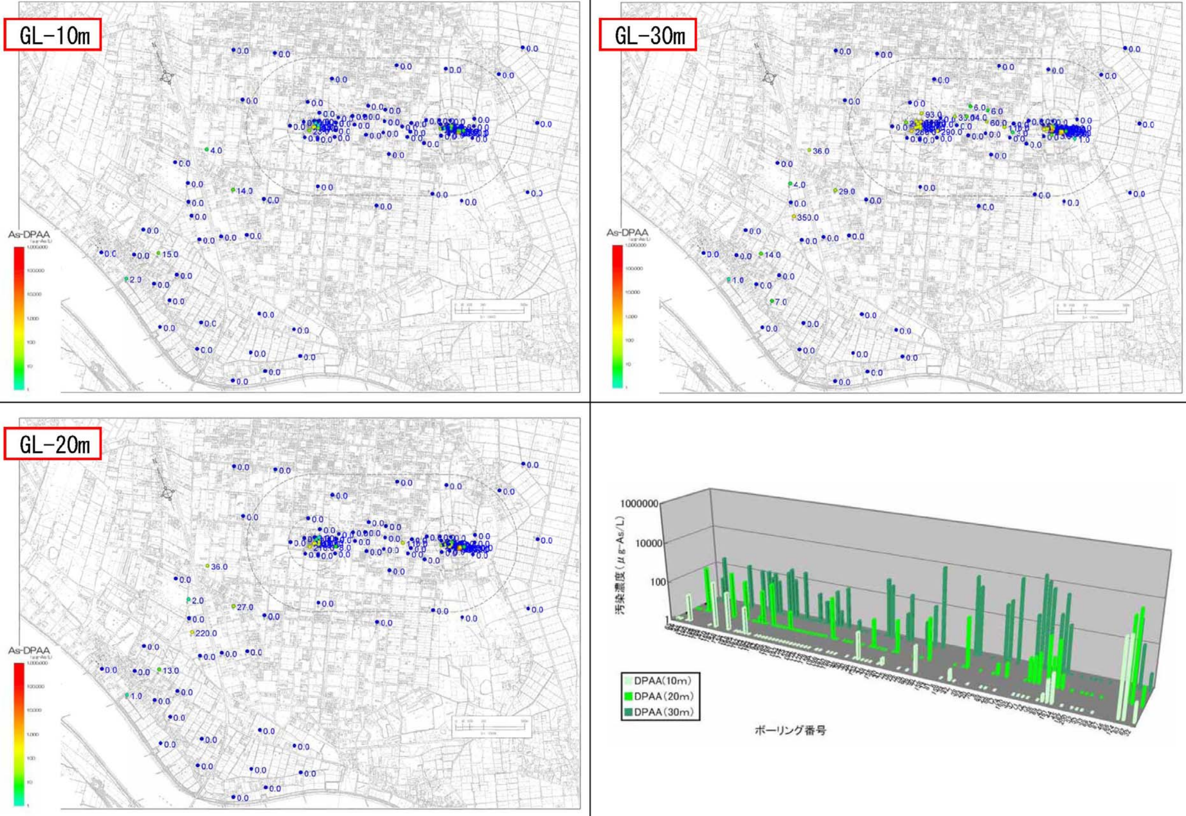
図 19 2008年春季(4月)ABトラック地下水DPAA汚染状況図
