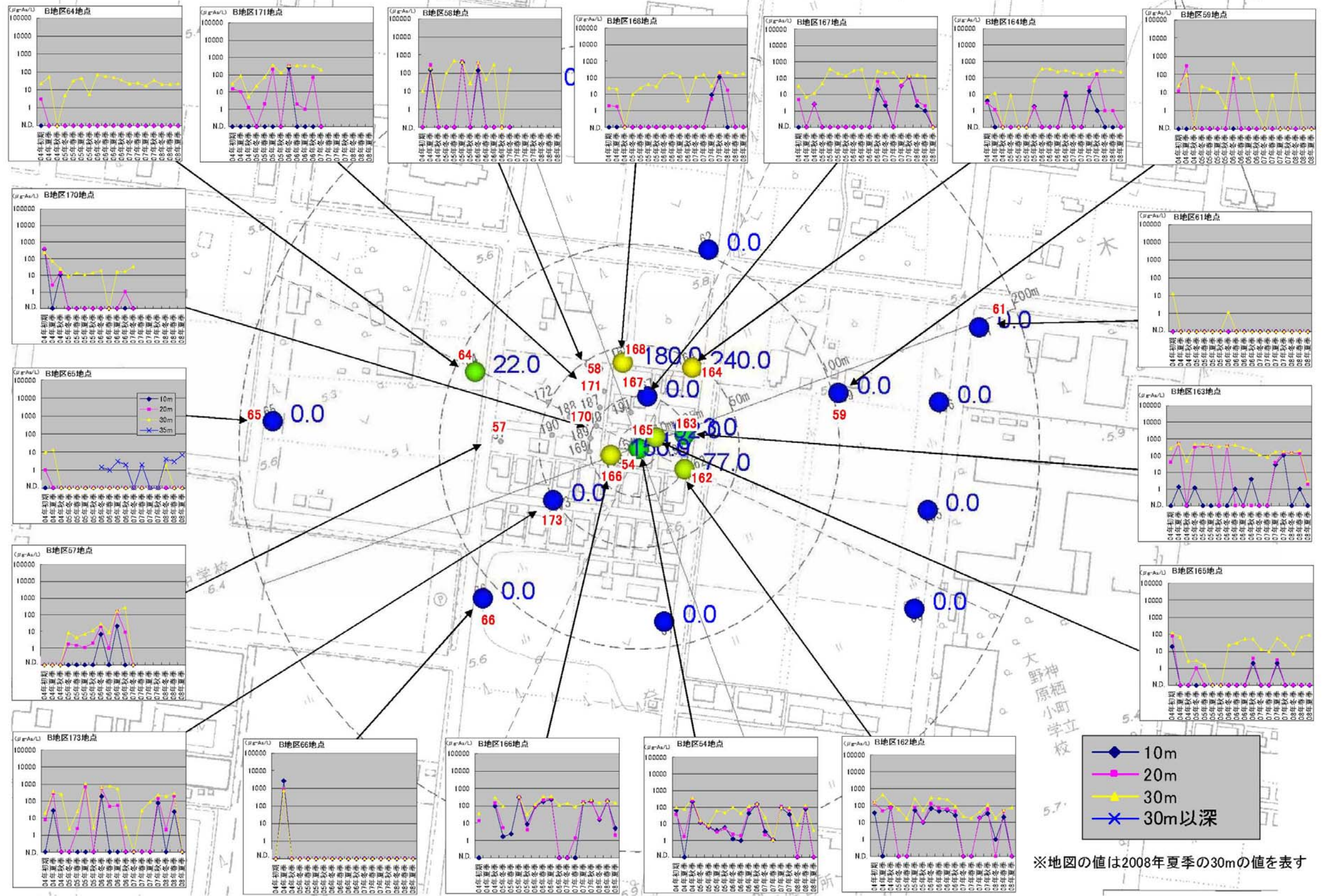
図 18 DPAA濃度変化 B地区 単位： \mu\text{g-As/L}
