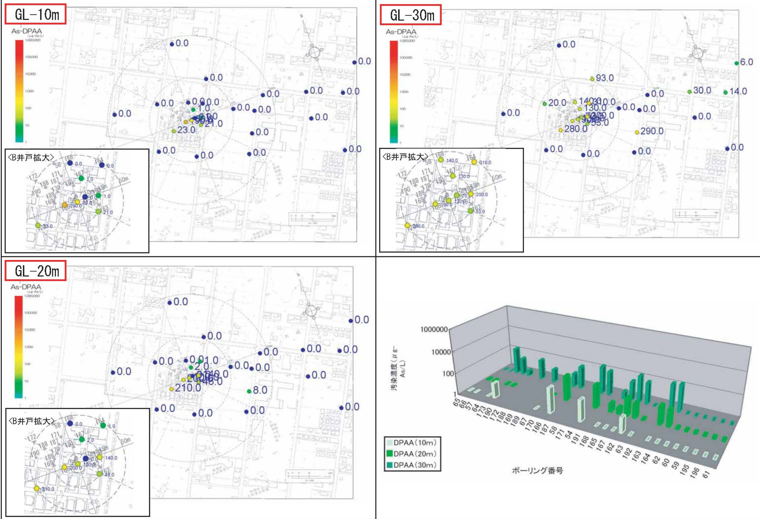
図 16 2008年春季(4月)B地区地下水DPAA汚染状況図
