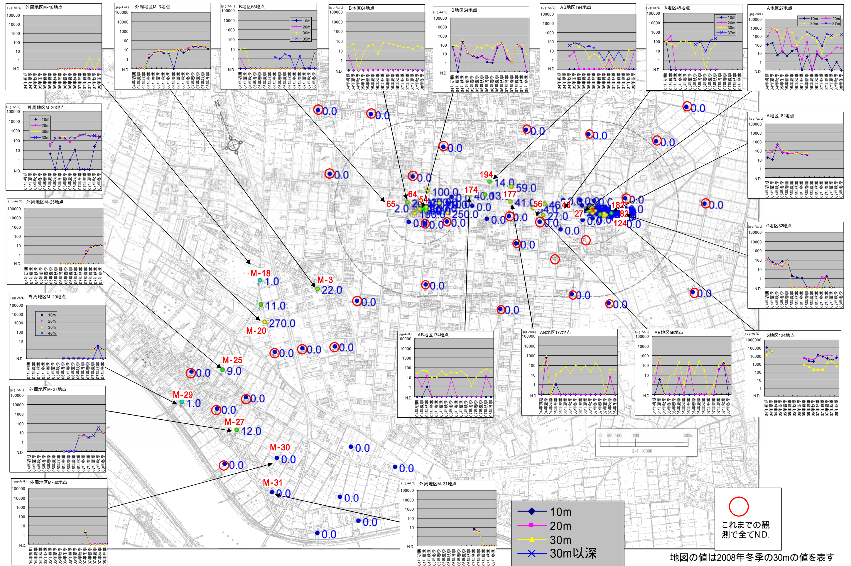
図 11 DPAA濃度変化 単位：μg-As/L
