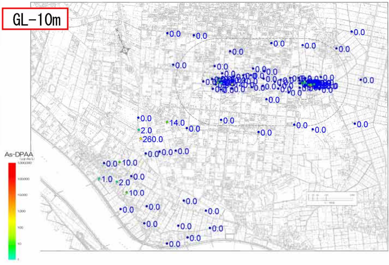
図 10 2008年冬季(1~2月)ABトラック地下水DPAA汚染状況図
