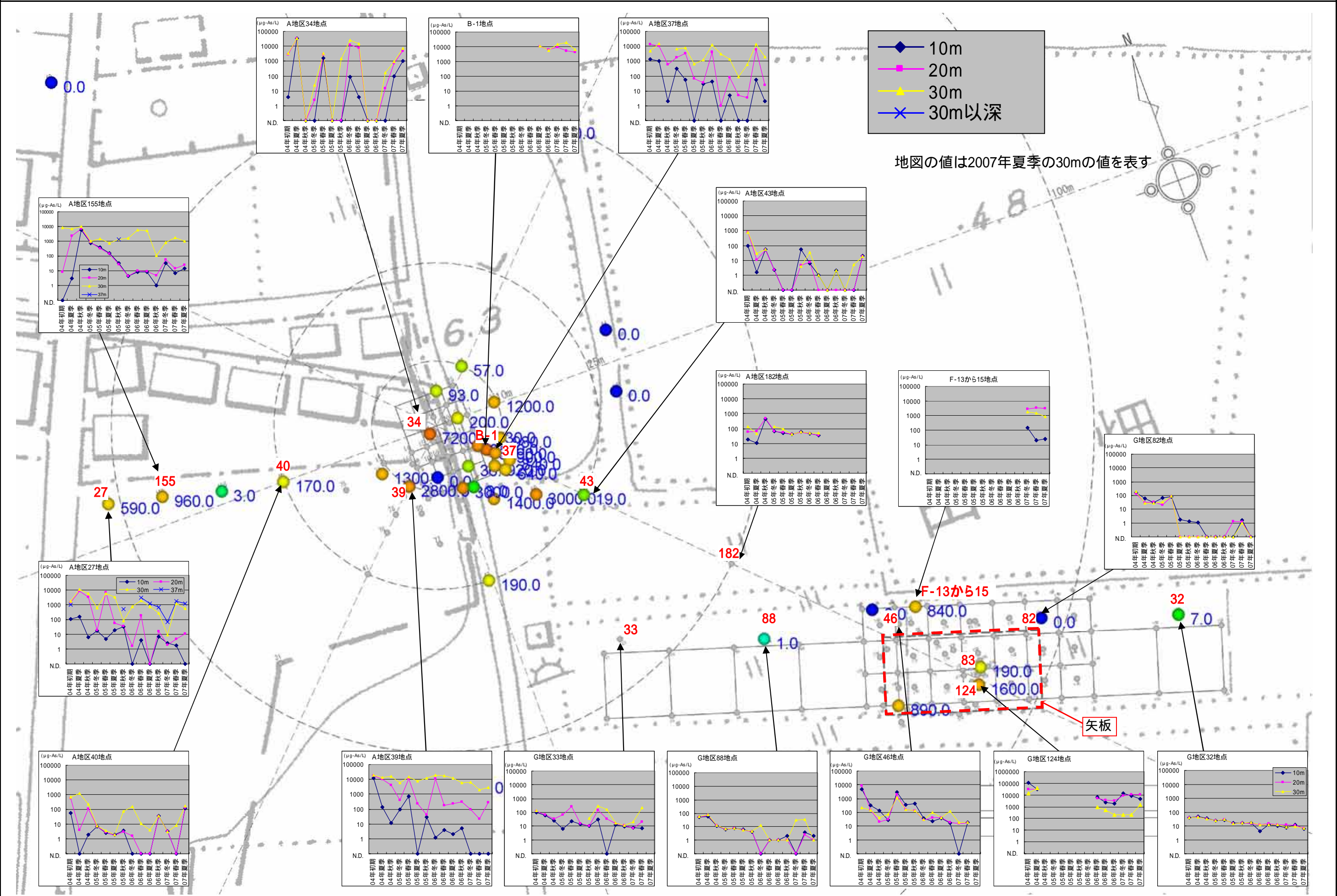
図11 DPAA濃度変化 A井戸周辺 単位：μg-As/L
