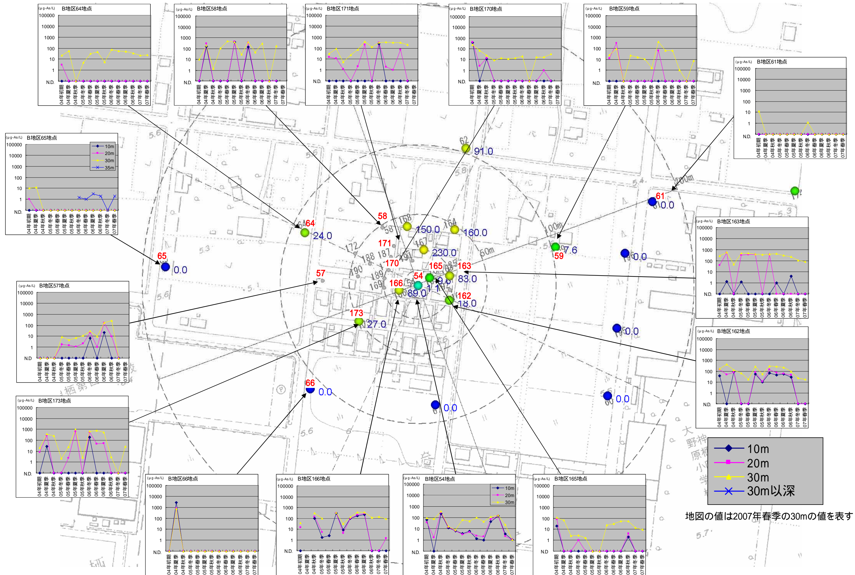
図8 B地区のDPAA濃の推移 (単位: \mu\text{g-As/L} )
