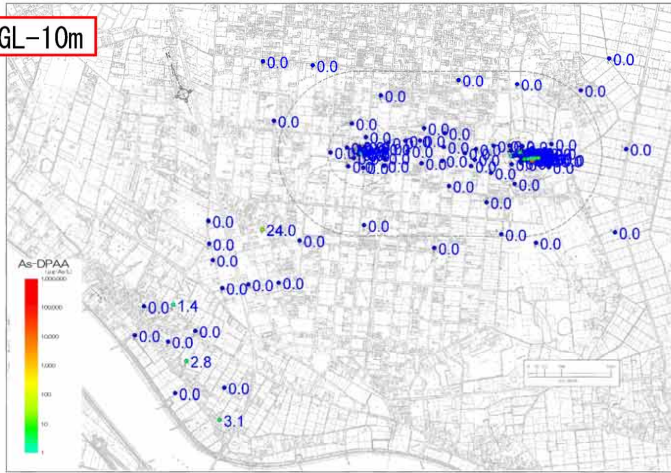
図9 2007年春季(4月)ABトラック地下水DPAA汚染状況図
