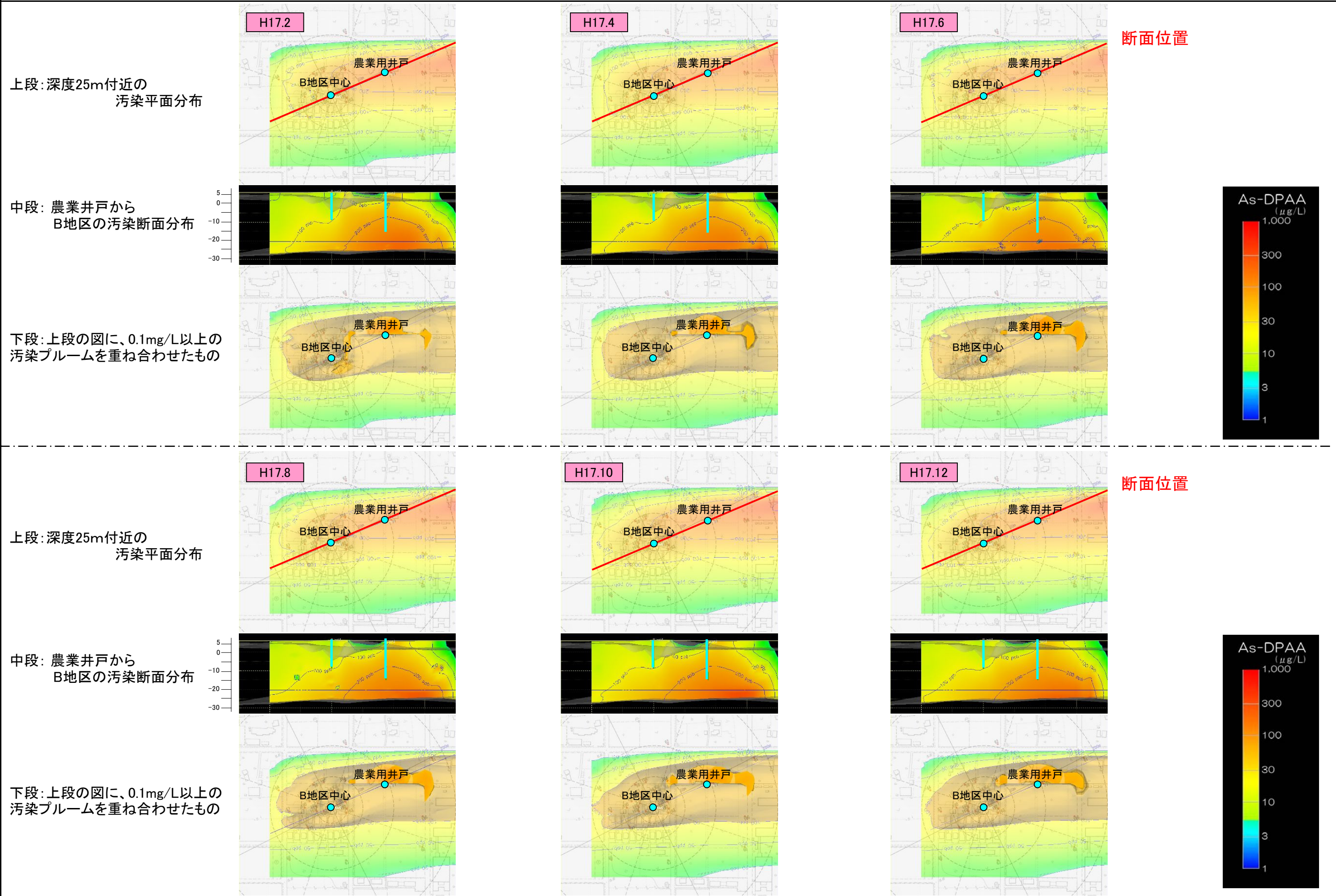
図6.1.4 B地区詳細地下水汚染シミュレーション結果 ⑧
