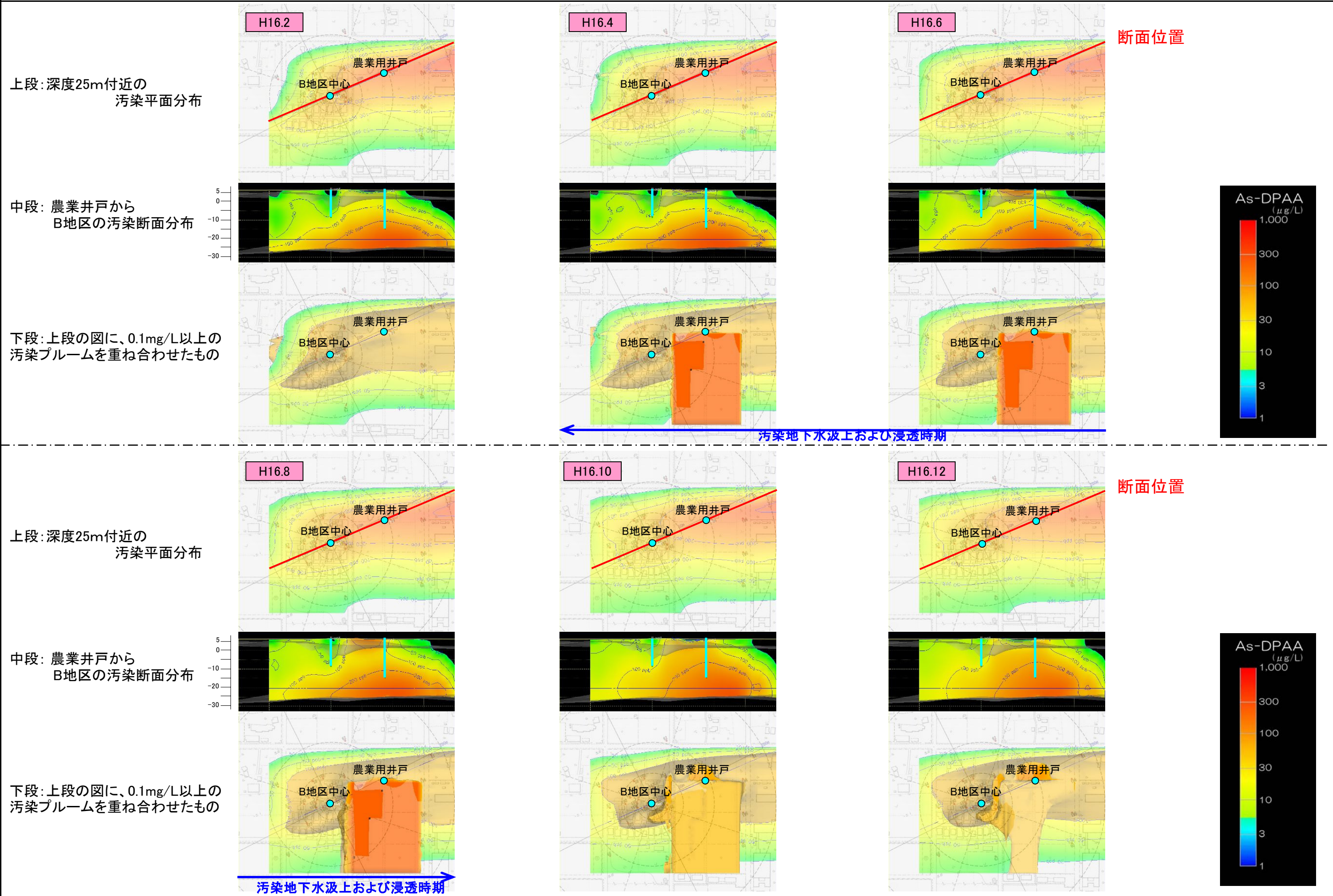
図6.1.4 B地区詳細地下水汚染シミュレーション結果 ⑦
