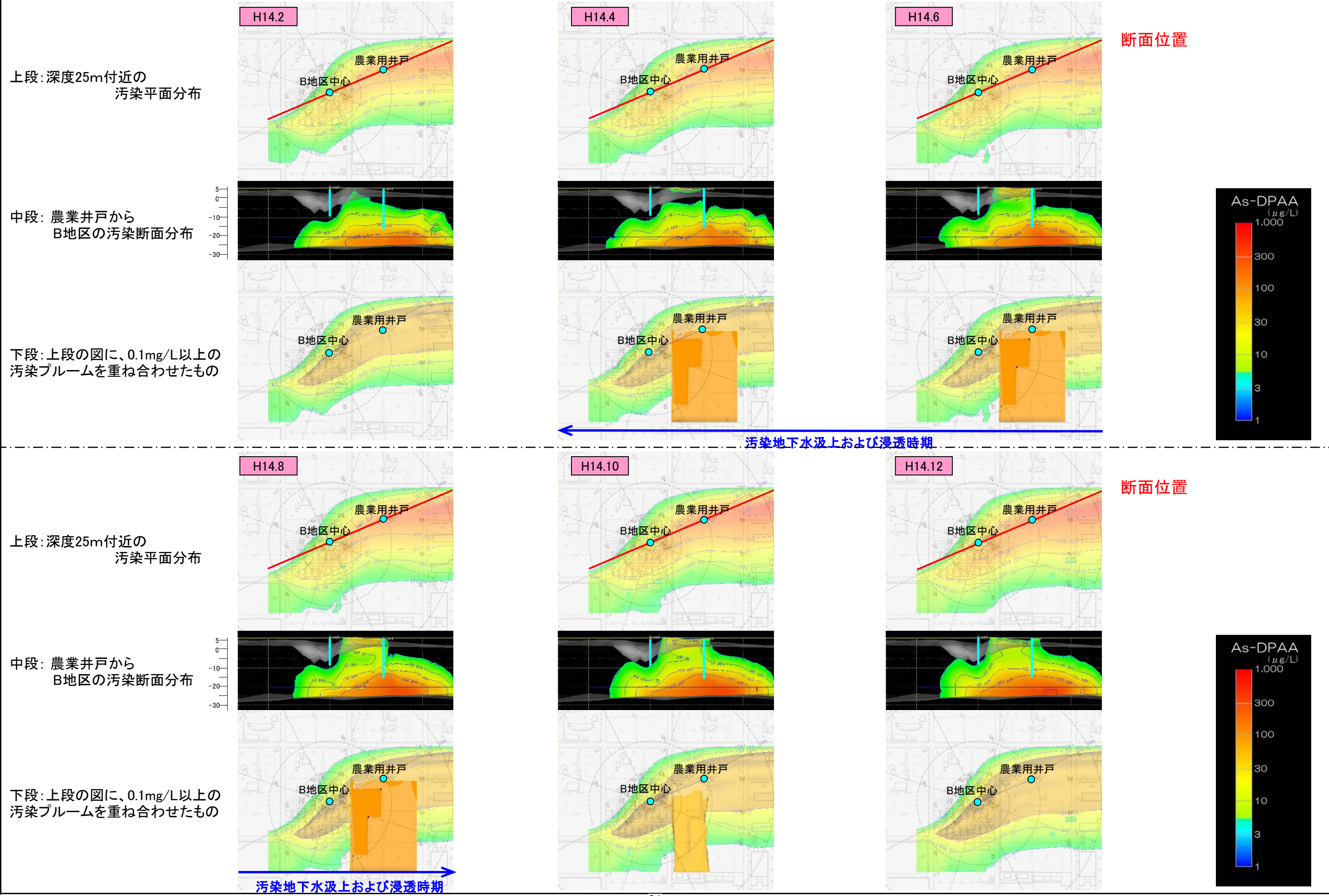
図6.1.4 B地区詳細地下水汚染シミュレーション結果 ⑤
