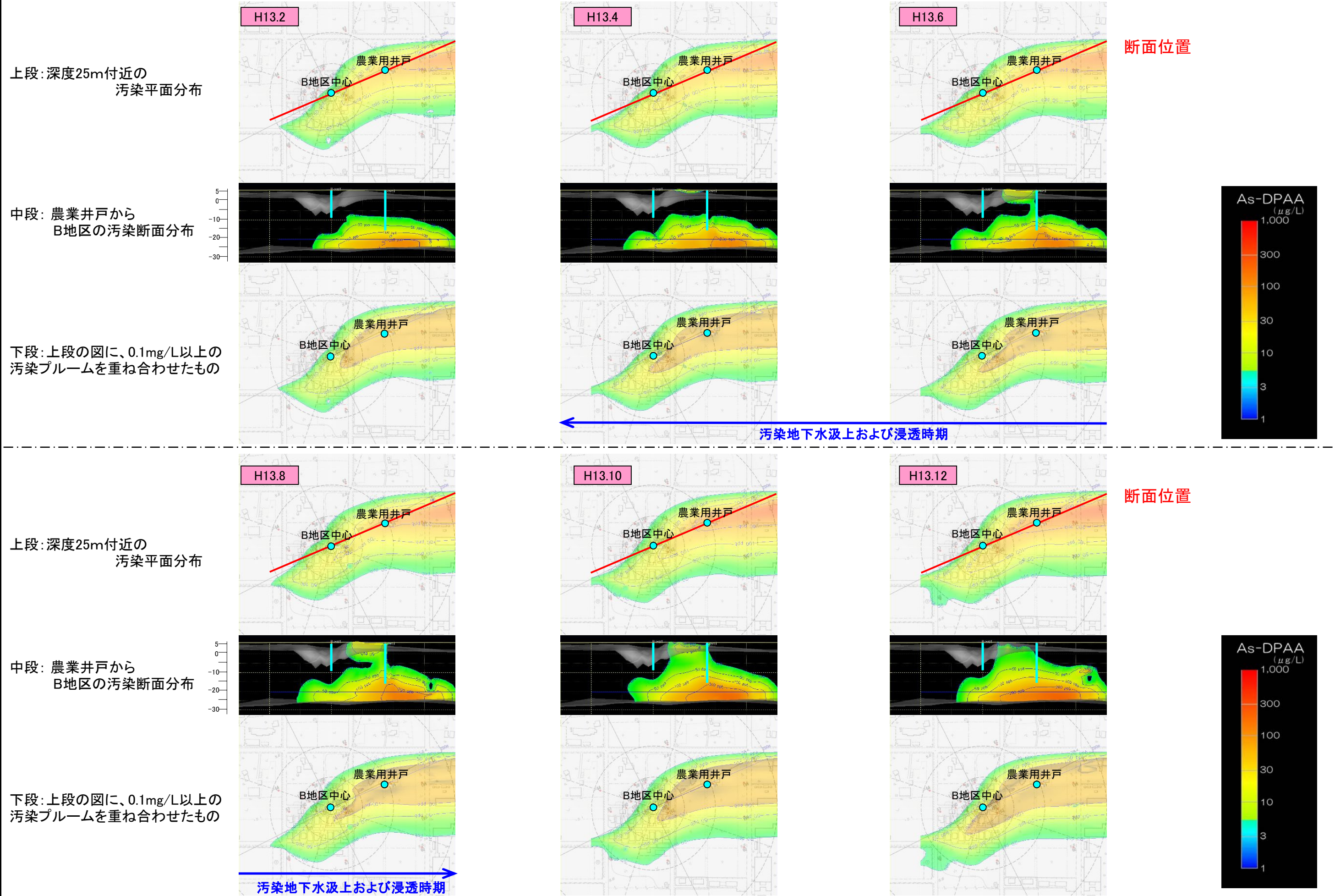
図6.1.4 B地区詳細地下水汚染シミュレーション結果 ④
