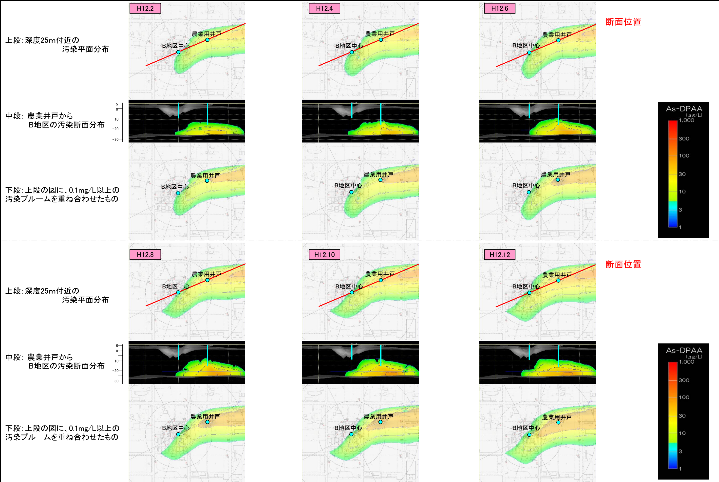
図6.1.4 B地区詳細地下水汚染シミュレーション結果 ③
