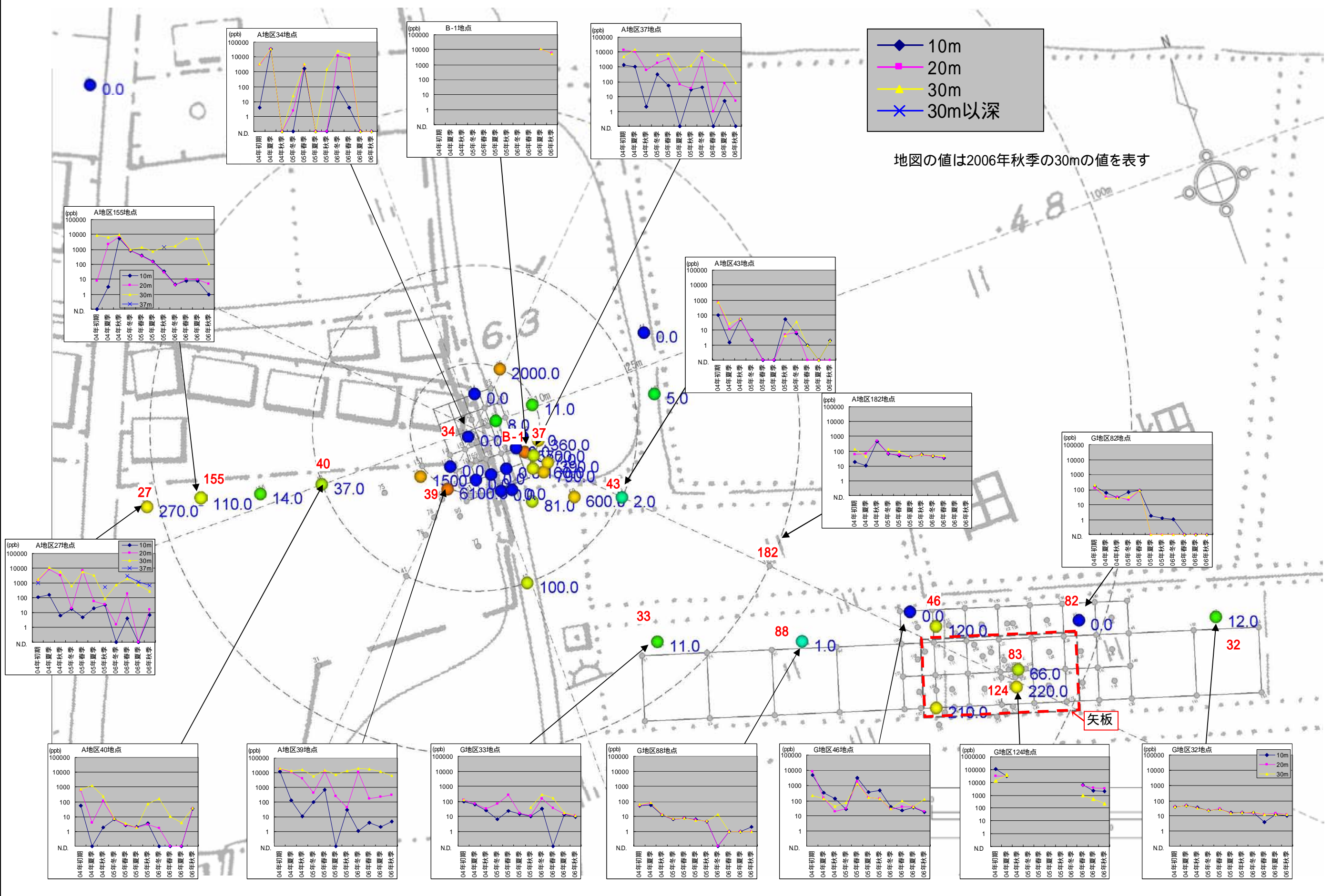
図6 DPAA濃度変化 A井戸周辺 (単位: ppb ヒ素換算値)
