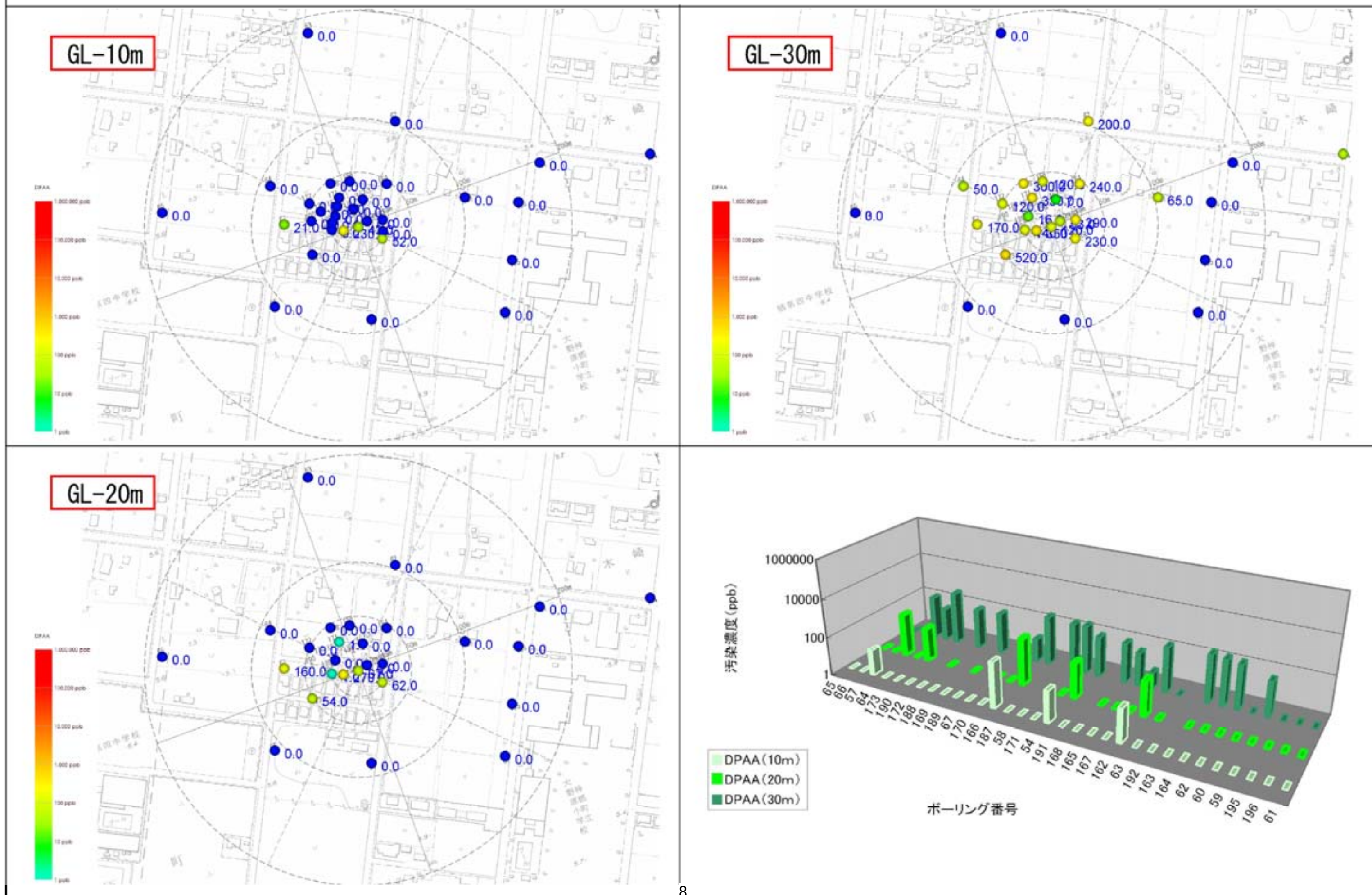
図6 2006年夏季(7~8月)B地区地下水DPAA汚染状況図
