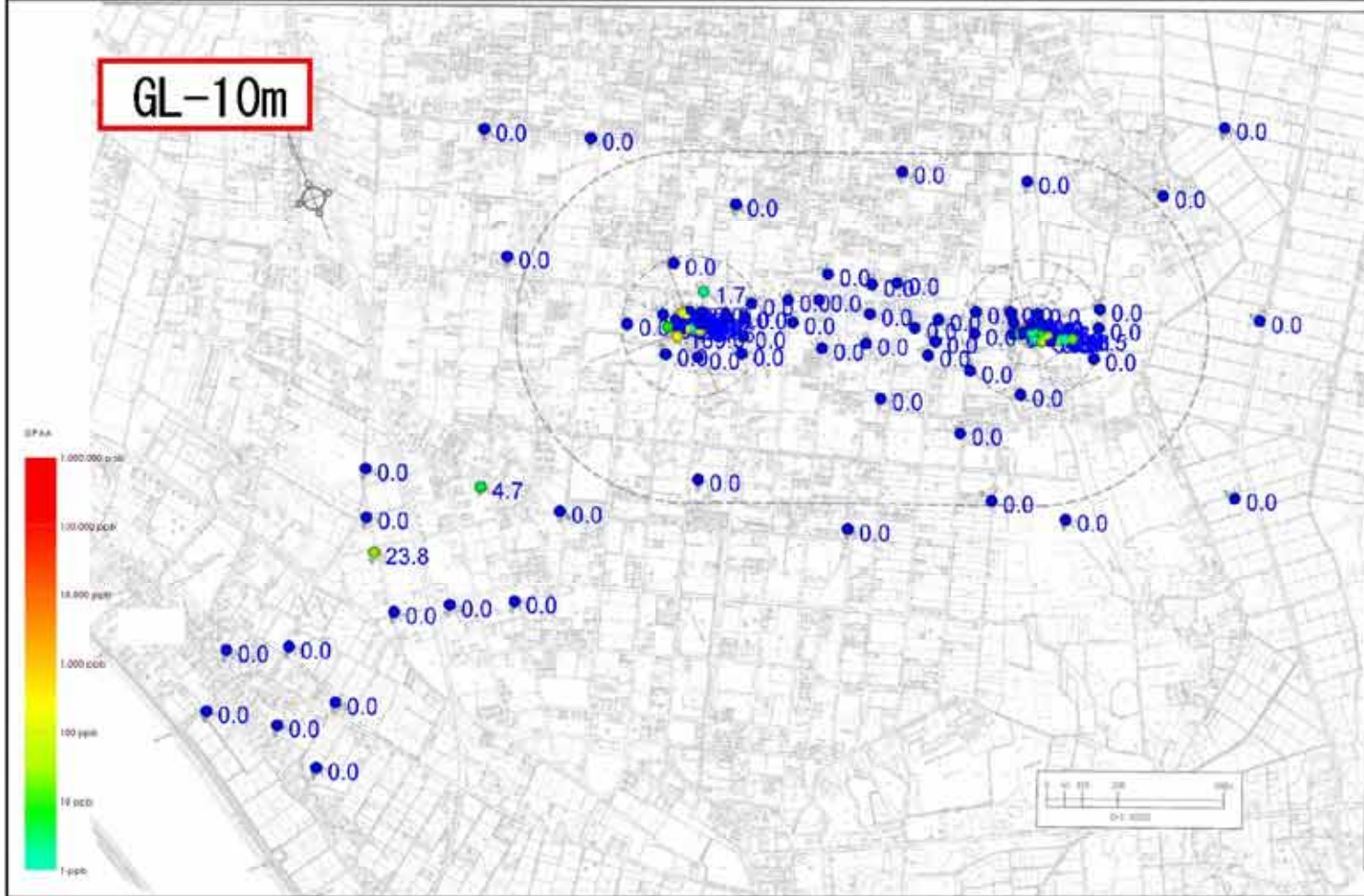
図8 2006年冬季(1~2月)ABトラック地下水DPAA汚染状況図
