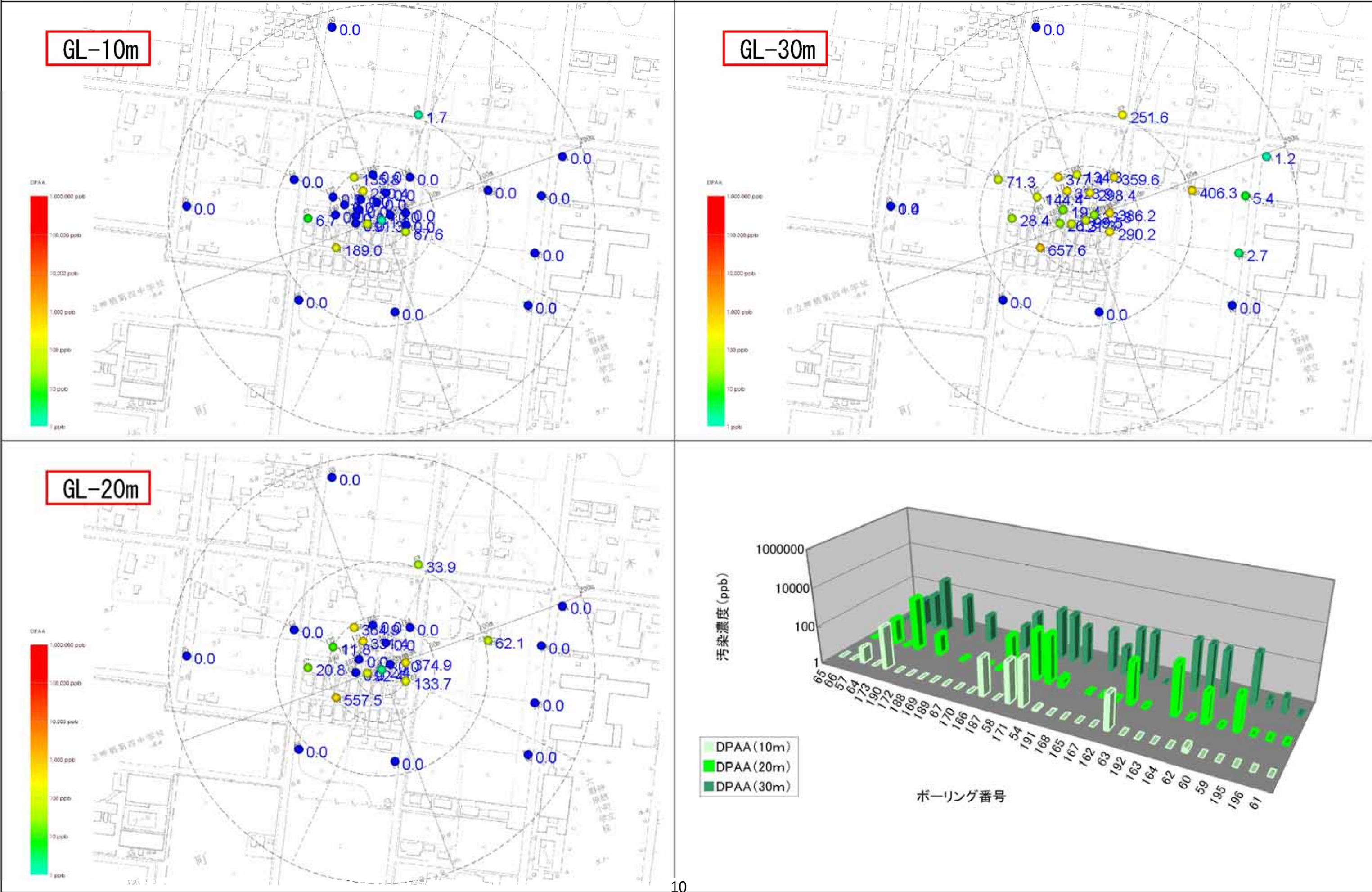
図7 2006年冬季(1～2月)B地区地下水DPAA汚染状況図
