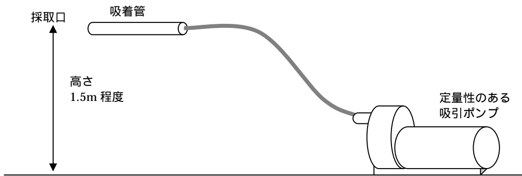
図 - 2 硫黄マスタードの大気試料採取装置の例
