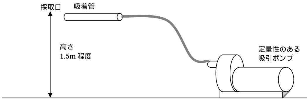
図 - 3 ルイサイトの大気試料採取装置の例
