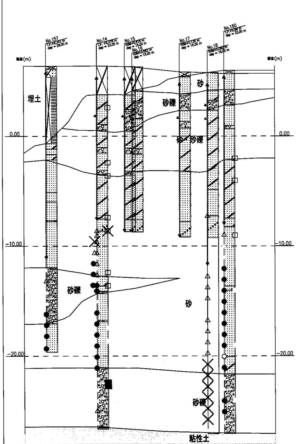
A地区直近東西断面図 (S=1:200) 西 東
