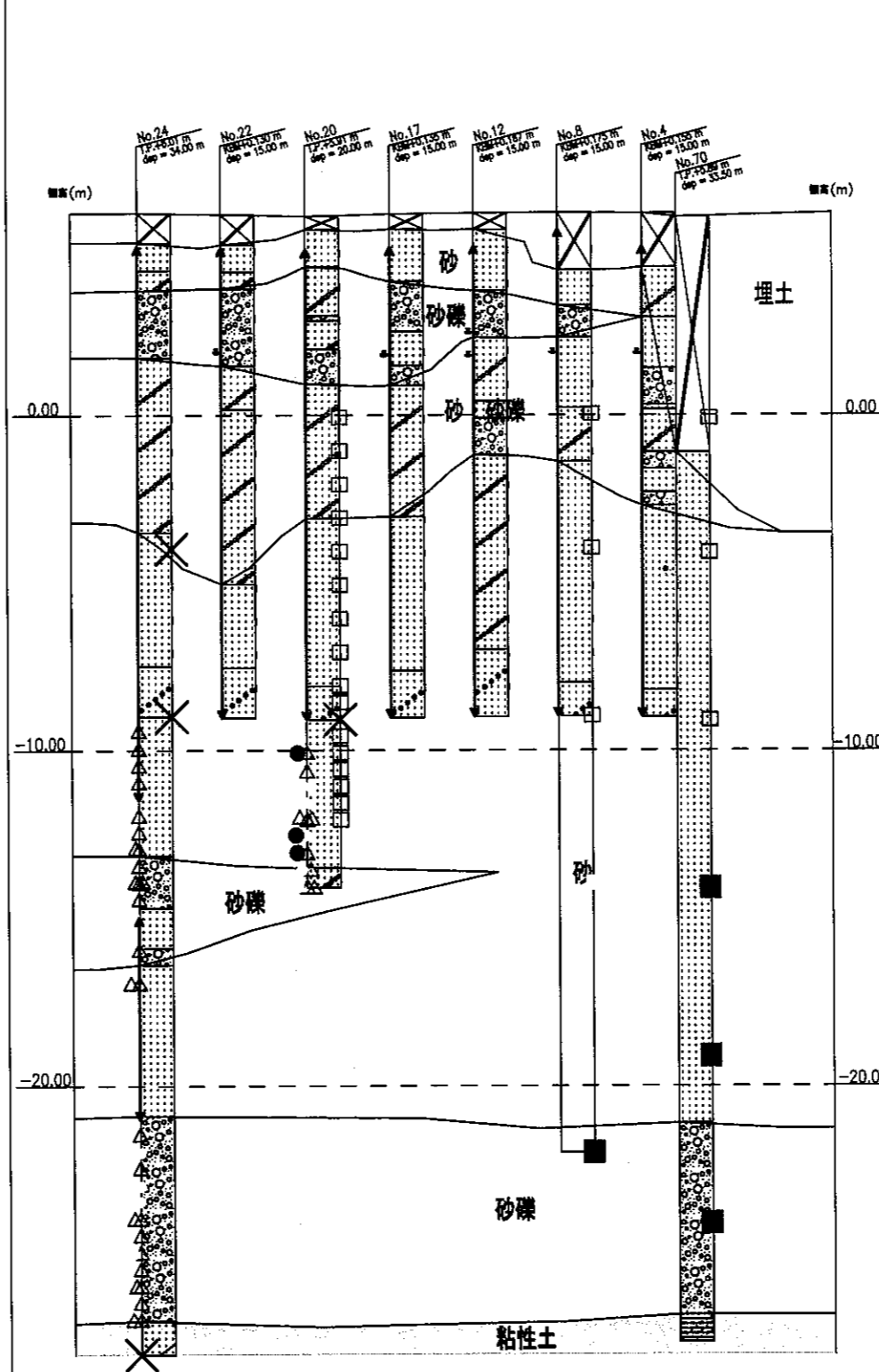
A地区直近南北断面図 (S=1:200) 北 南
