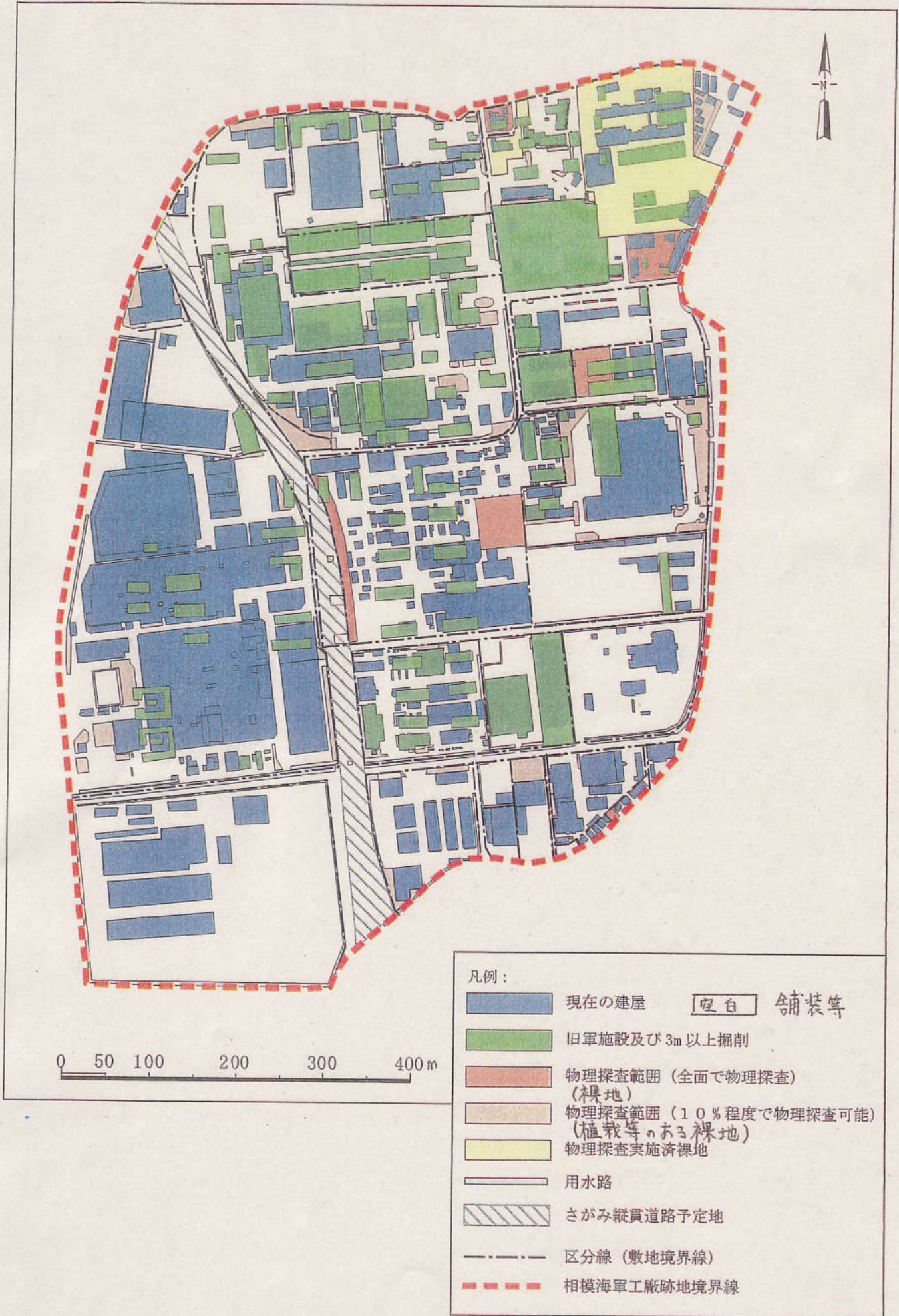
図 - 寒川町における物理探査調査地点（案）
