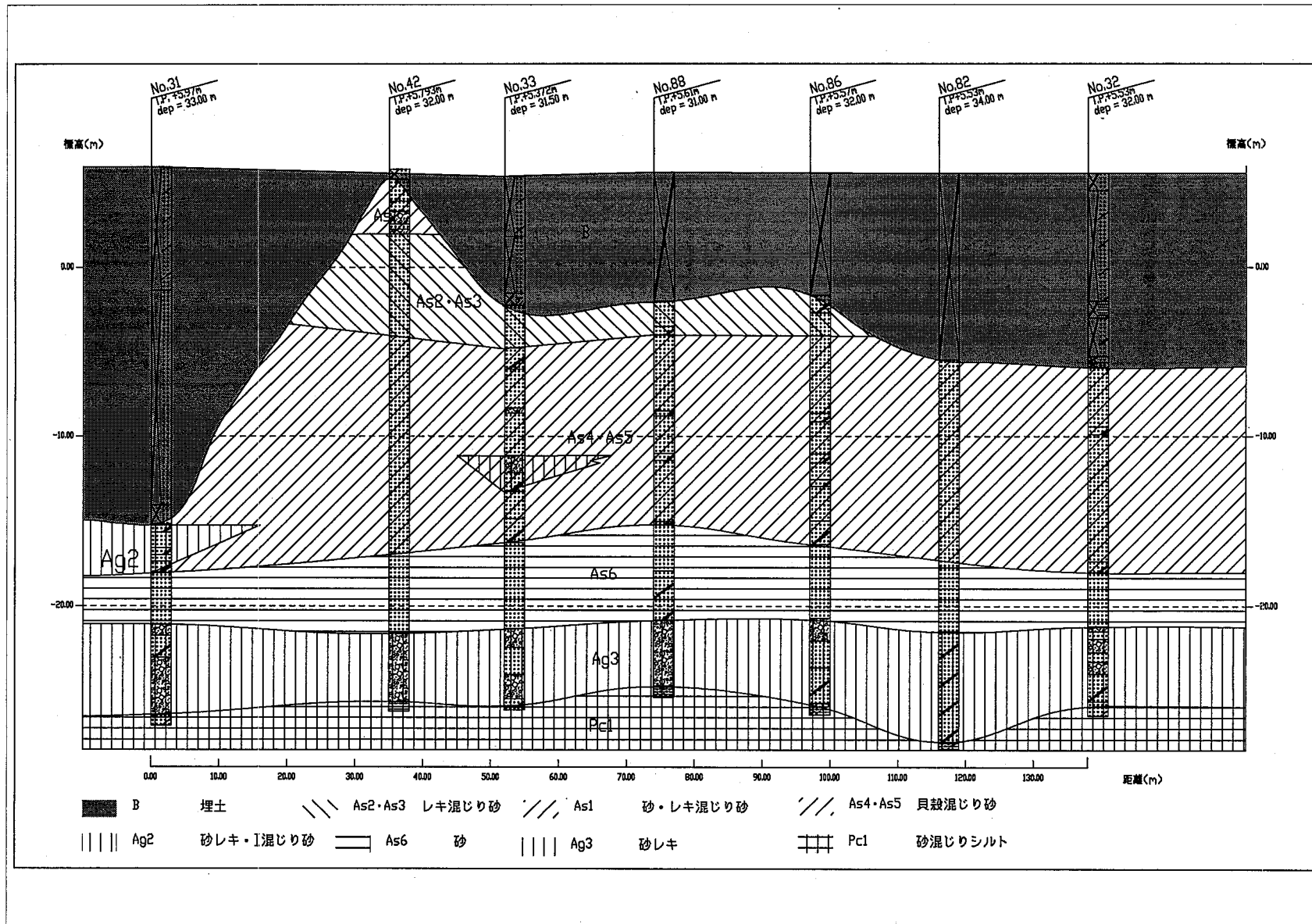
グラウンド東側空き地 東西方向の地質断面図
