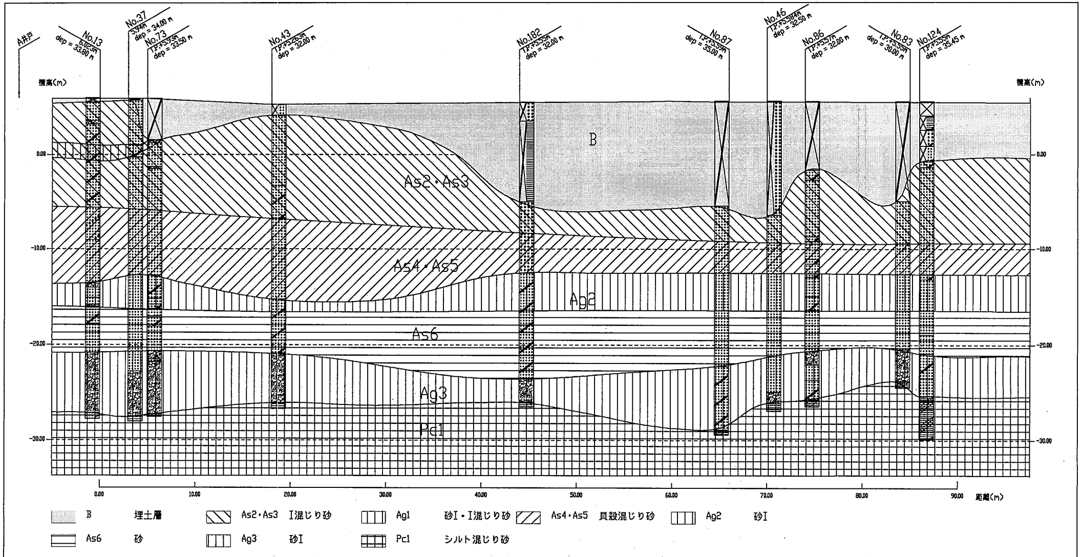
No.124~A井戸の地質断面図
