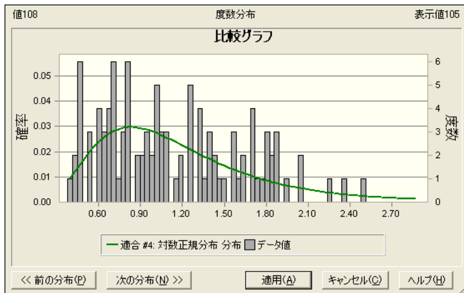
図 2-12 食事データへの対数正規分布の適合
