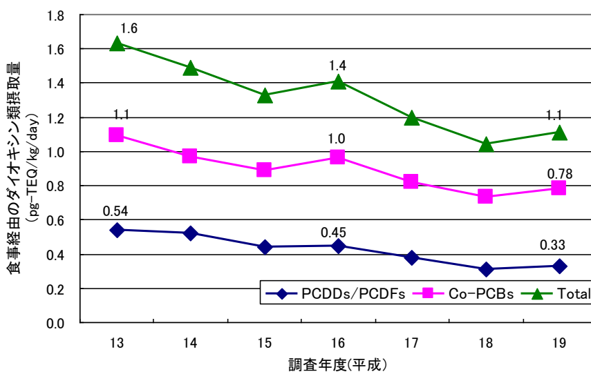
図 2-4 個人ばく露量（算術平均）
