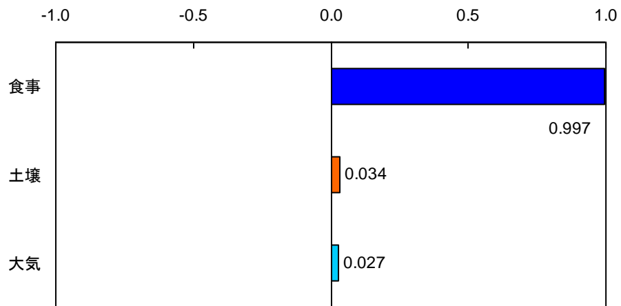
図 2-25 モデル 2 個人総ばく露量への各変数の寄与率 (順位相関による感度グラフ)
