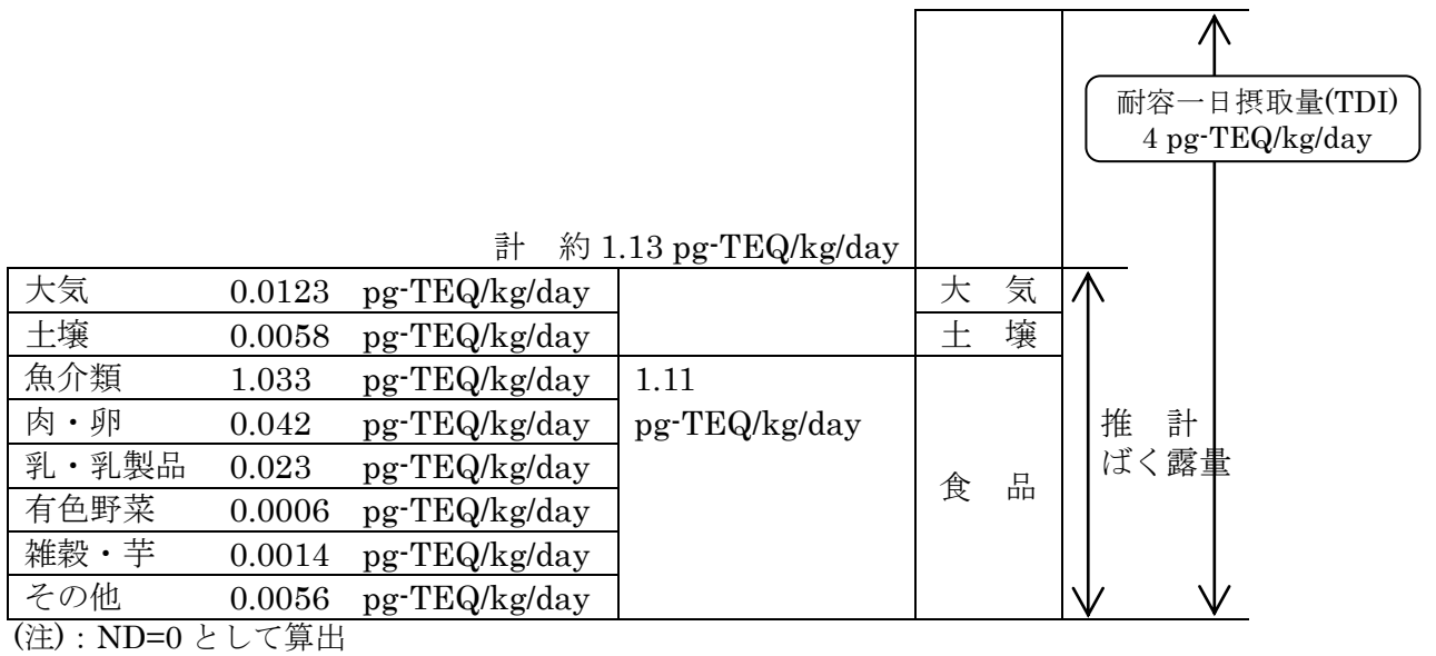
図 2-1 一般環境における個人総ばく露量の内訳 (平成 19 年度)
