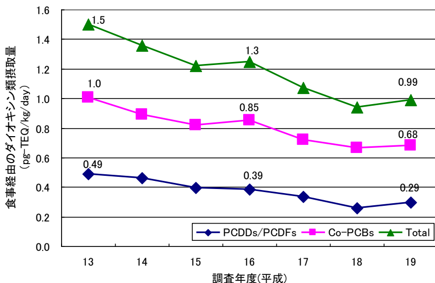
図 2-5 個人ばく露量（幾何平均）
