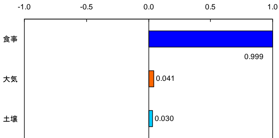
図 2-27 モデル 3 個人総ばく露量への各変数の寄与率 (順位相関による感度グラフ)
