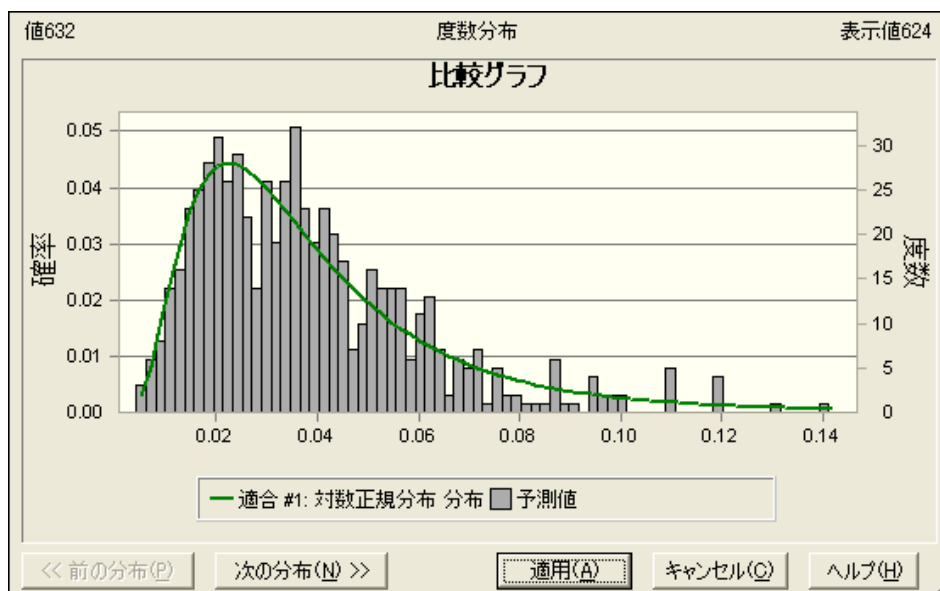
図 2-6 大気データ（一般環境+沿道）への対数正規分布の適合
