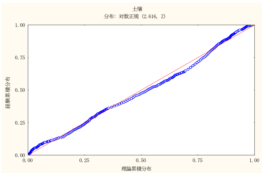
図 2-9 土壌中ダイオキシン類濃度の P-P プロット（対数正規分布）
