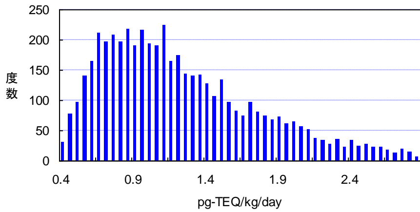
図 2-16 モデル1 個人総ばく露量推計結果 (度数分布)
