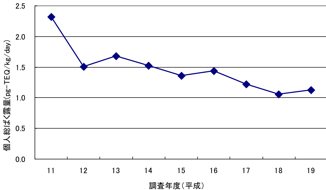
図 2-2 一般環境における個人総ばく露量の推移 (算術平均) (表 2-1 における推計結果②参照)
