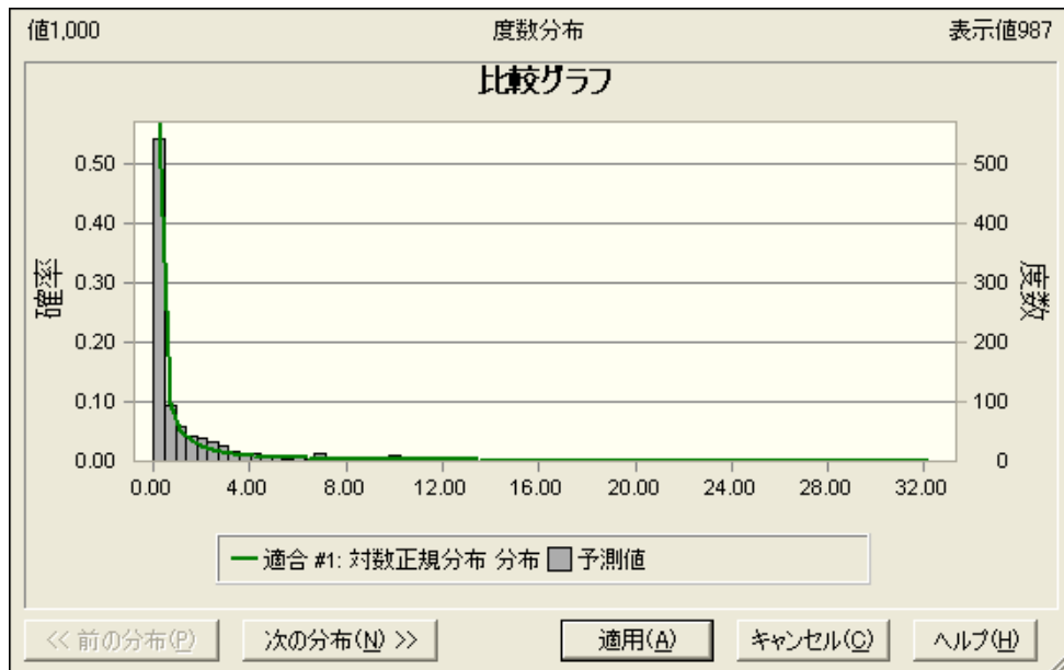
図 2-8 土壌データ（一般環境）への対数正規分布の適合
