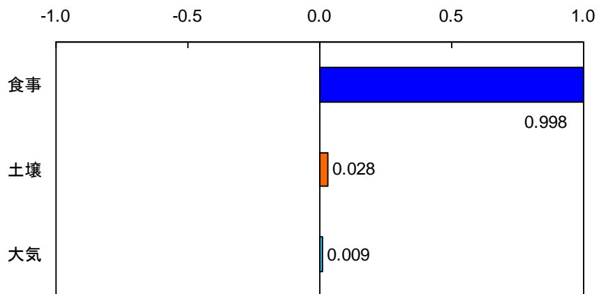
図 2-23 モデル 1 個人総ばく露量への各変数の寄与率 （順位相関による感度グラフ）
