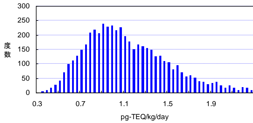
図 2-24 モデル 2 個人総ばく露量推計結果 (度数分布)
