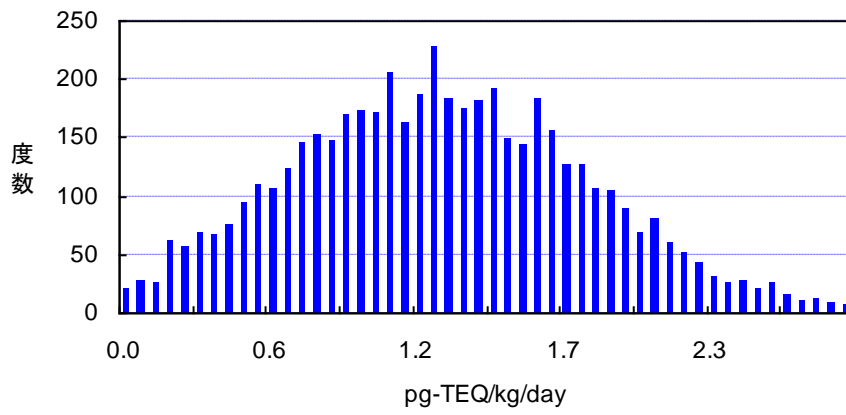
図 2-20 モデル 3 個人総ばく露量推計結果 (度数分布)
