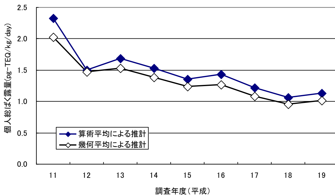
図 2-3 一般環境における個人総ばく露量の推移
