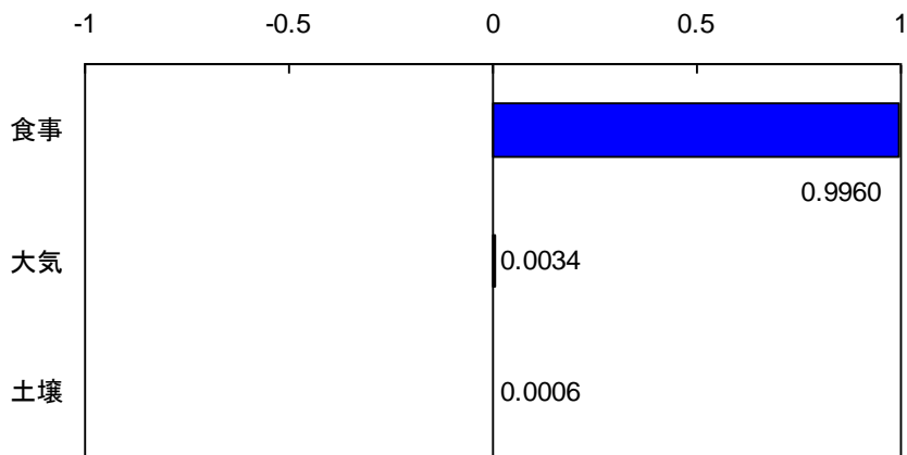
図 2-17 モデル1 個人総ばく露量への各変数の寄与率 (順位相関による感度グラフ)
