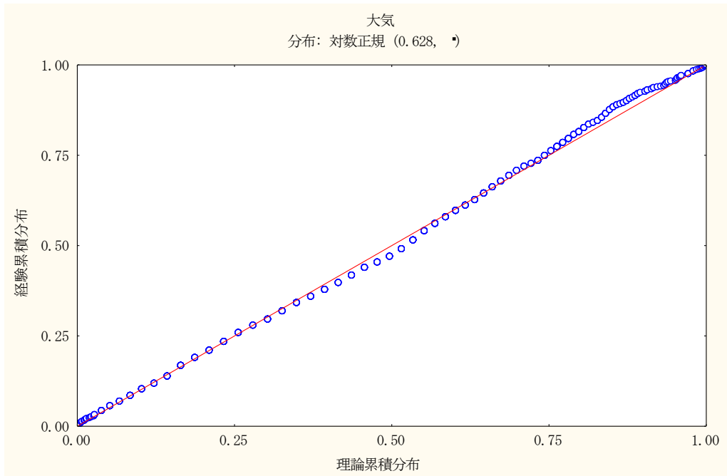
図 2-7 大気中ダイオキシン類濃度の P-P プロット (対数正規分布)
