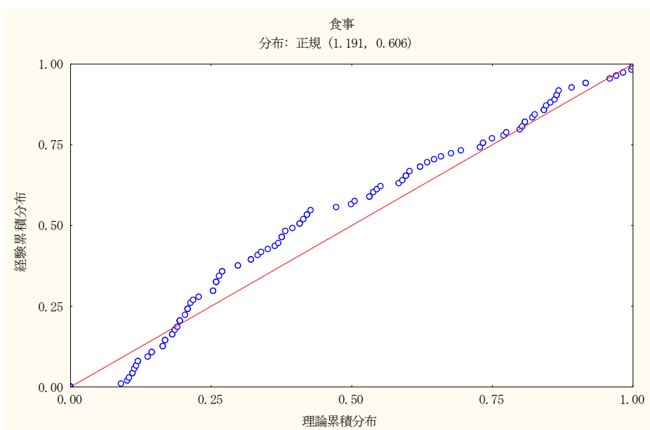
図 2-15 食事中ダイオキシン類の P-P プロット (正規分布)
