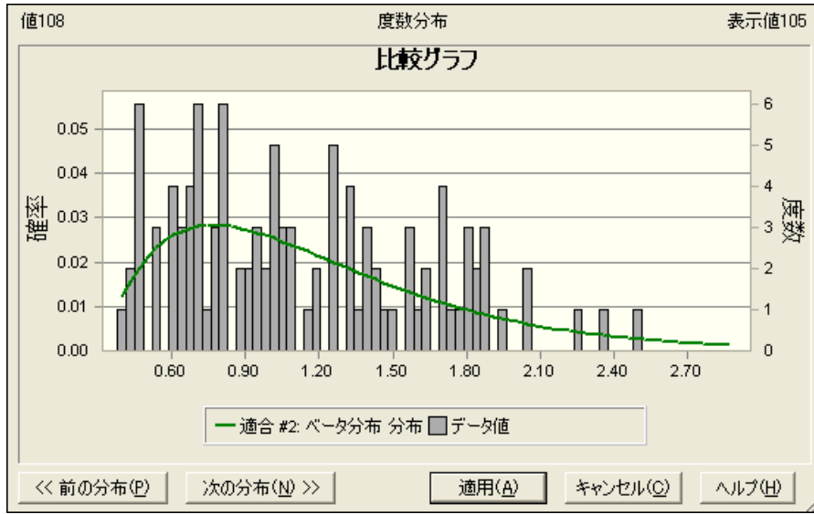
図 2-10 食事データへのベータ分布の適合
