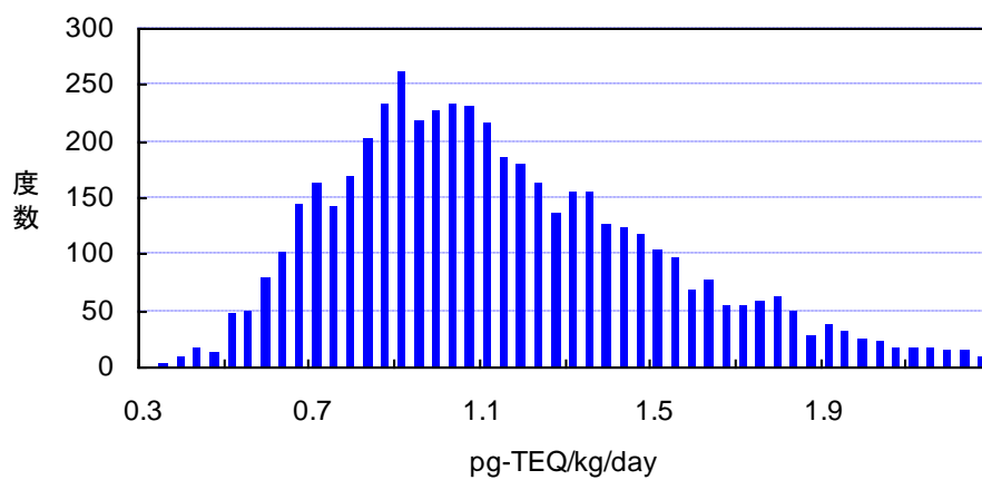
図 2-18 モデル 2 個人総ばく露量推計結果 (度数分布)
