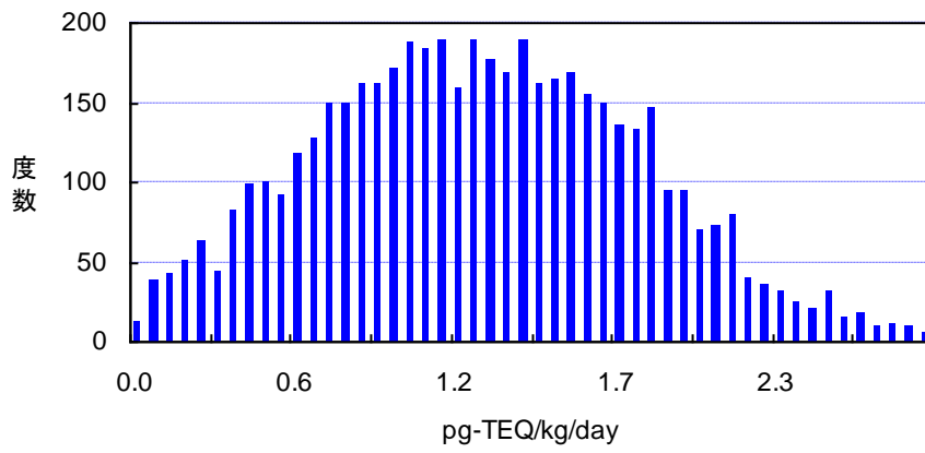
図 2-26 モデル 3 個人総ばく露量推計結果 (度数分布)
