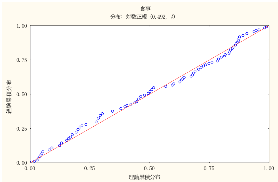
図 2-13 食事中ダイオキシン類の P-P プロット (対数正規分布)
