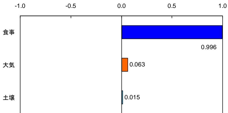
図 2-21 モデル 3 個人総ばく露量への各変数の寄与率 (順位相関による感度グラフ)
