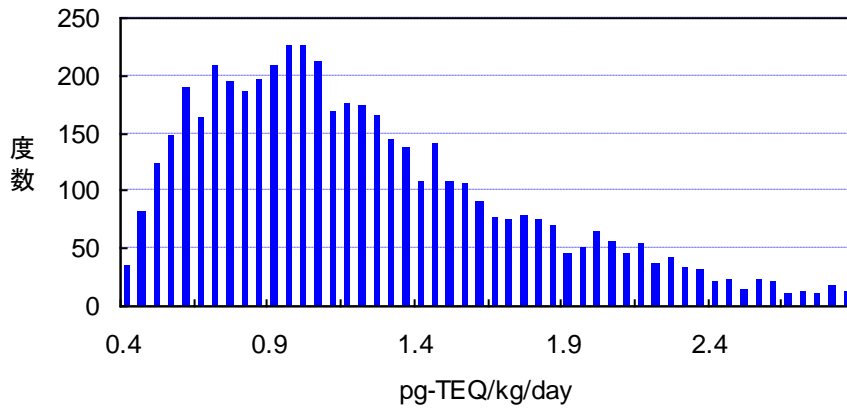
図 2-22 モデル 1 個人総ばく露量推計結果（度数分布）
