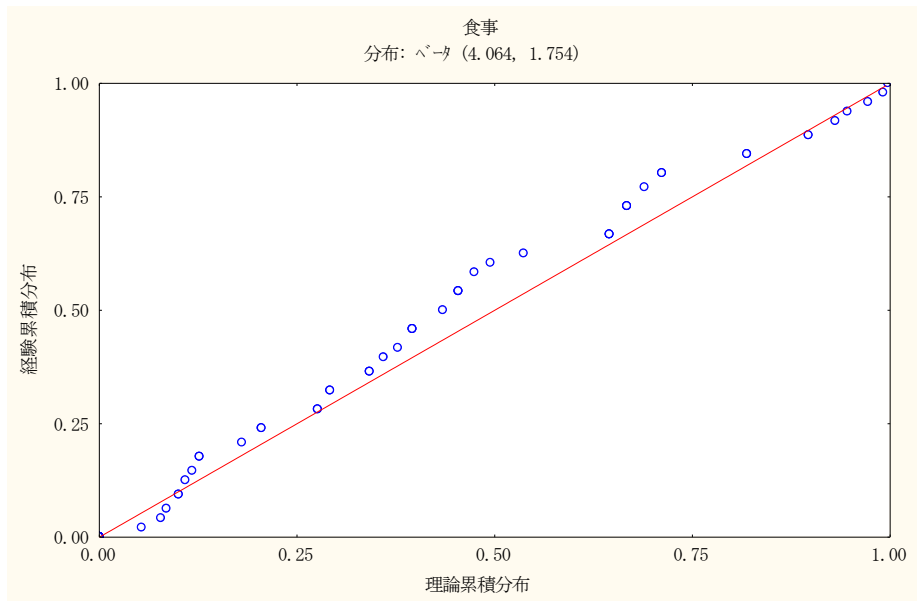
図 2-11 食事中ダイオキシン類の P-P プロット ( \beta 分布)
