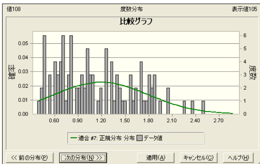
図 2-14 食事データへの正規分布の適合
