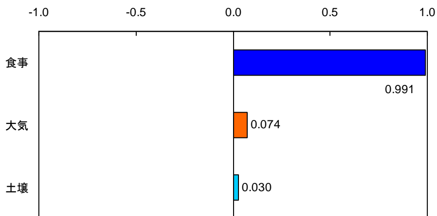
図 2-19 モデル 2 個人総ばく露量への各変数の寄与率 (順位相関による感度グラフ)
