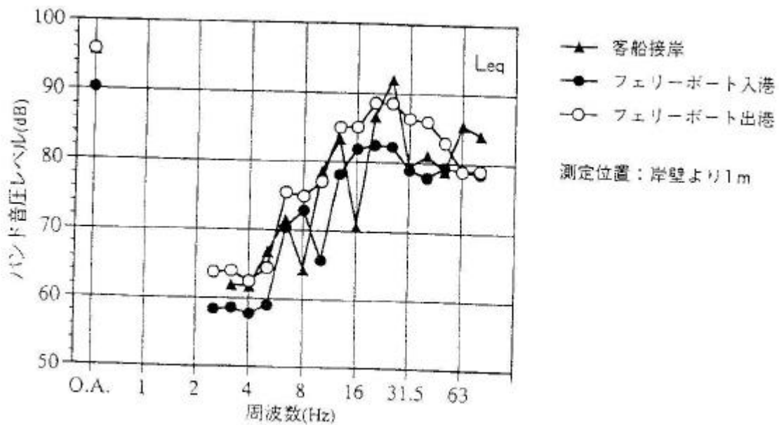
図-e.8 低周波音の周波数特性の例（港周辺）
