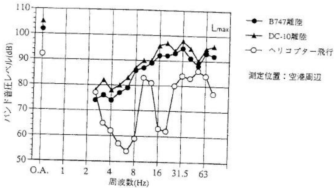
図-e.7 低周波音の周波数特性の例（航空機・ヘリコプター）
