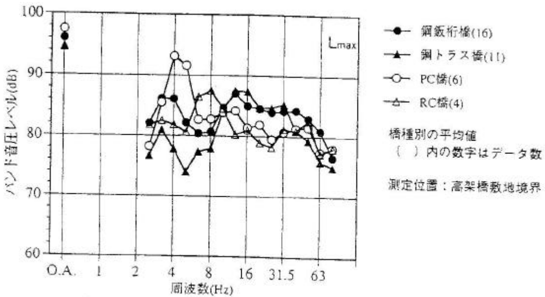
図-e.6 低周波音の周波数特性の例（道路高架橋）
