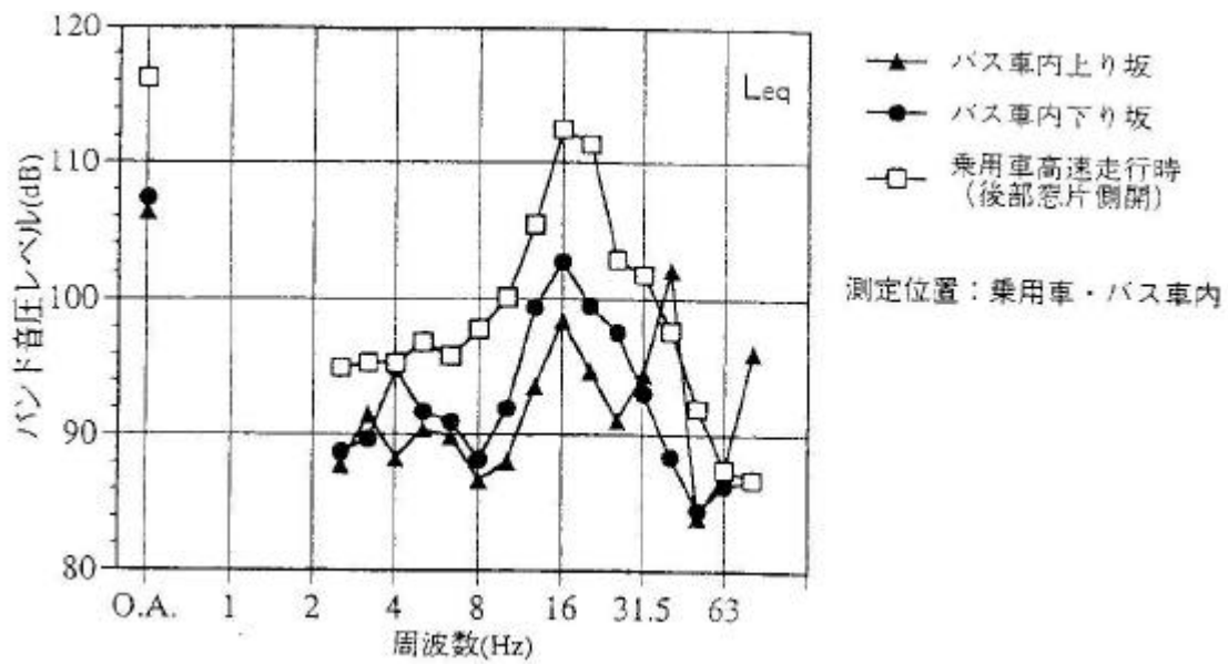
図-e.5 低周波音の周波数特性の例（乗り物車内）
