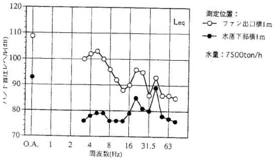
図-e.4 低周波音の周波数特性の例（クーリングタワー）
