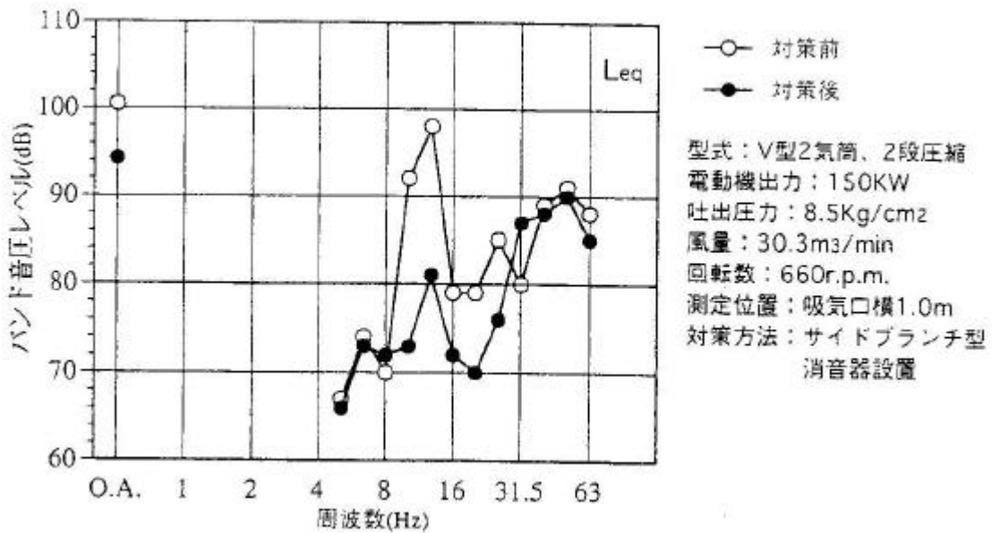
図-e.3 低周波音の周波数特性の例（圧縮機）
