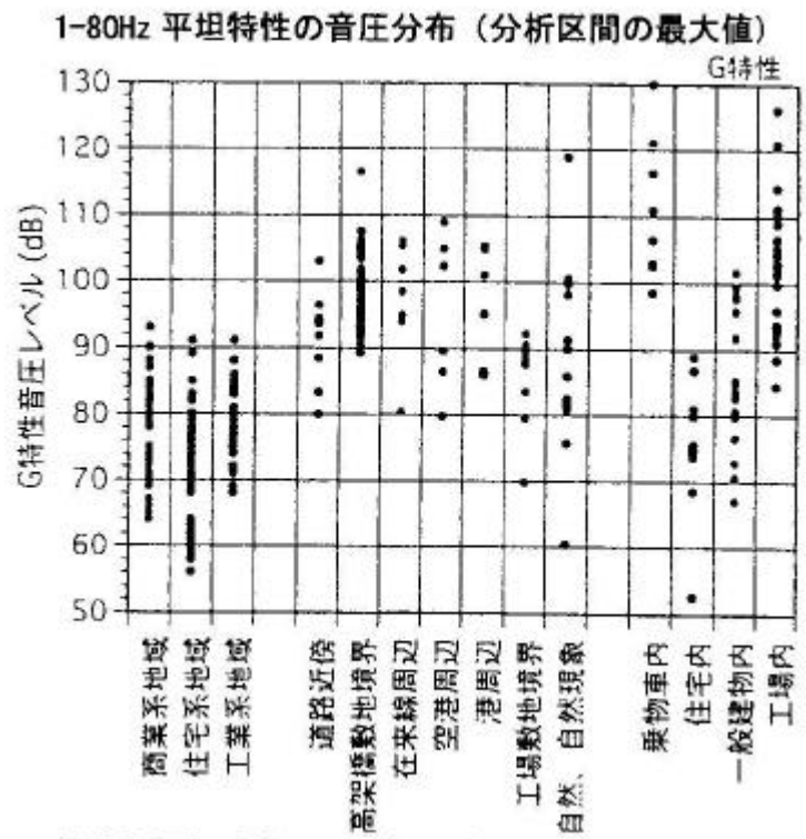
図-e.2 発生源周辺を含めた一般住宅空間における G 特性音圧レベル分布 (分析区間の最大値)
