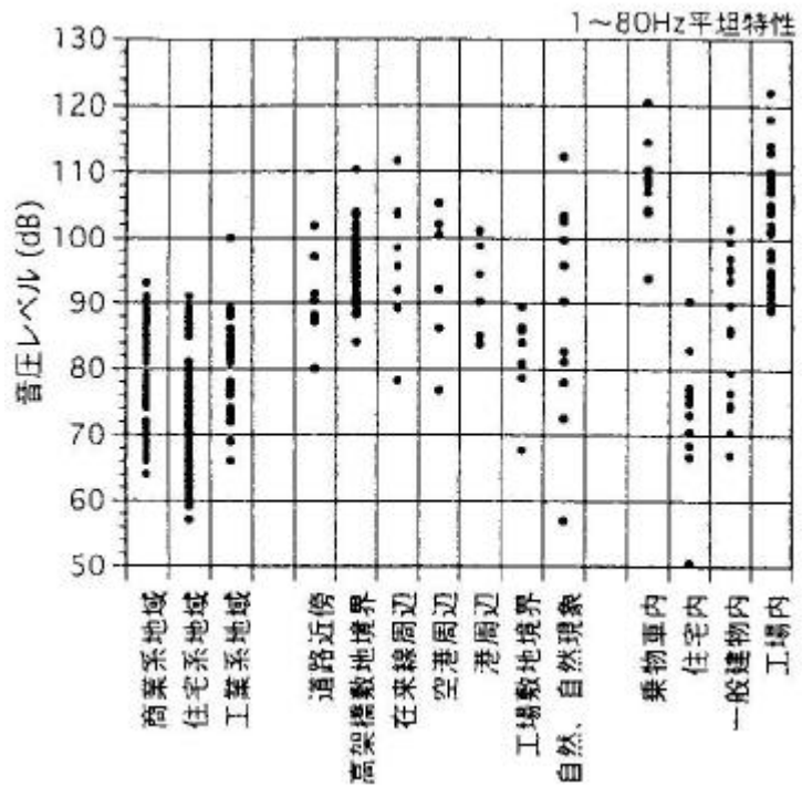
図-e.1 発生源周辺を含めた一般住宅空間における 1-80Hz 平坦特性の音圧分布 (分析区間の最大値)
