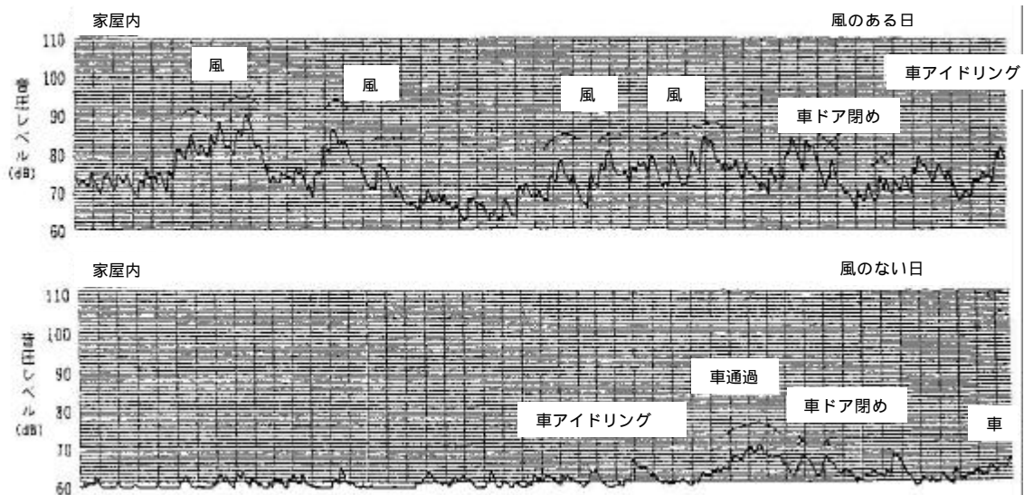
図-5.3.8 風のある日とない日における家屋内の低周波音測定例
