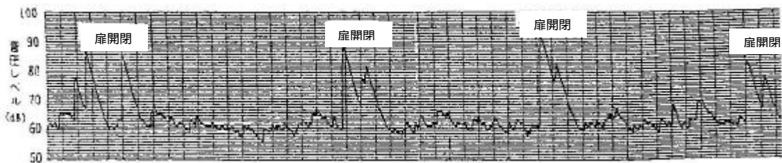
図-5.3.9 扉の開閉によるレベル変動の例
