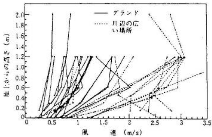
図-5.3.6 風速の垂直分布
