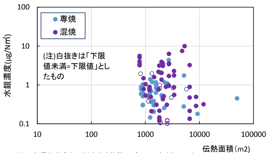
図 II-1-11 伝熱面積と全水銀濃度
