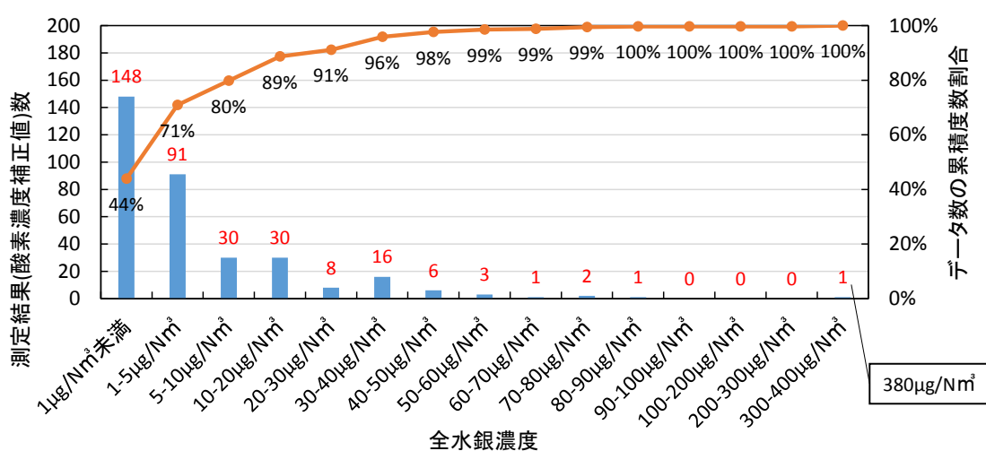
図 II-4-1-1 排ガス中全水銀濃度 ヒストグラム（産業廃棄物焼却炉）
