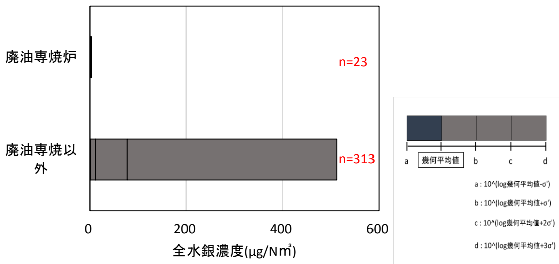
図 II-4-1-8 焼却対象物の種類（廃油）と全水銀濃度（対数標準偏差）
