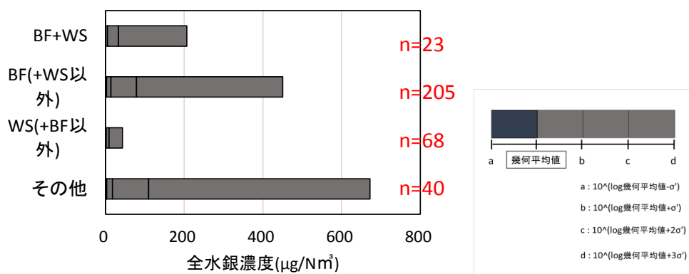
図 II-4-1-3 対数標準偏差による排ガス処理方式と全水銀濃度（産業廃棄物焼却炉）
