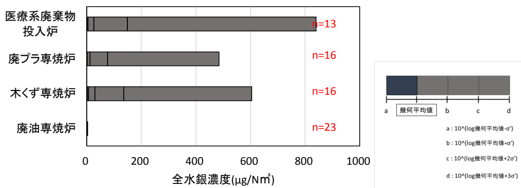
図 II-4-1-6 産業廃棄物焼却炉における焼却対象物の種類と全水銀濃度 (対数標準偏差)
