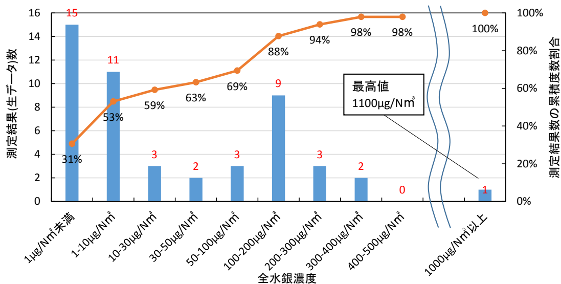
図 II-3-2 排ガス中全水銀濃度 ヒストグラム (非鉄二次施設 亜鉛)
