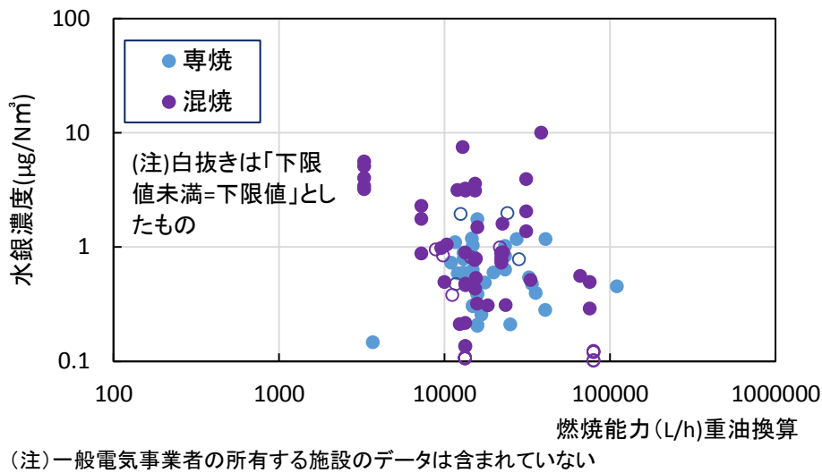
図Ⅱ-1-12 燃烧能力と全水銀濃度
