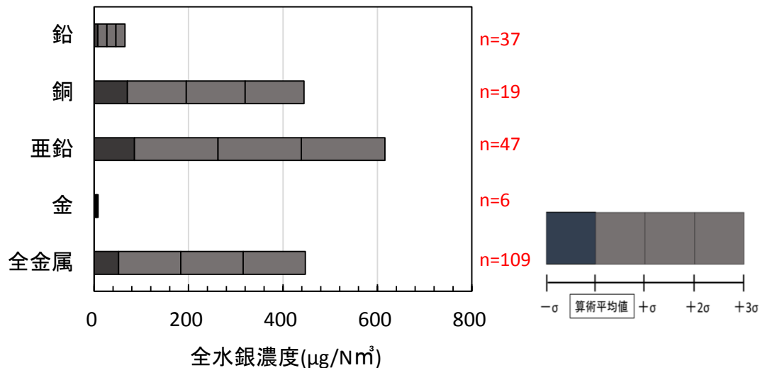
図 II-3-6 非鉄二次施設の金属種類と濃度分布
