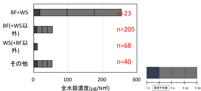
図 II-4-1-2 排ガス処理方式と全水銀濃度（産業廃棄物焼却炉）
