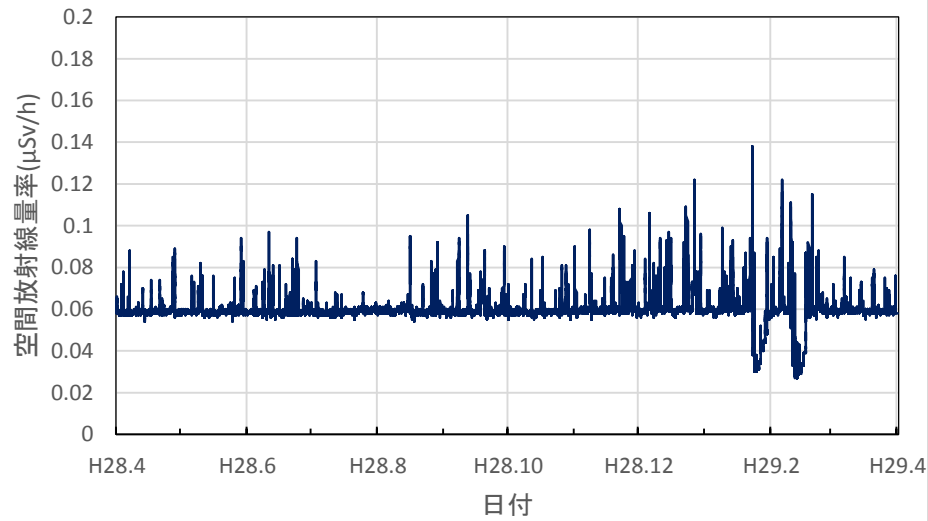
鳥取県琴浦町 きらりタウン赤碕の空間放射線量率(10分値使用)
