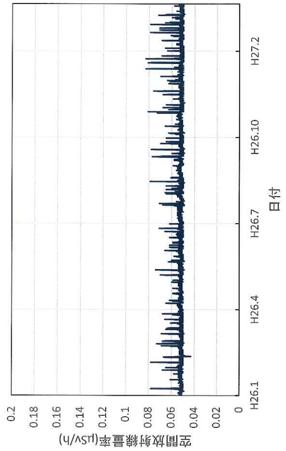
三重県伊勢市 伊勢庁舎の空間放射線量率(10分値使用)
