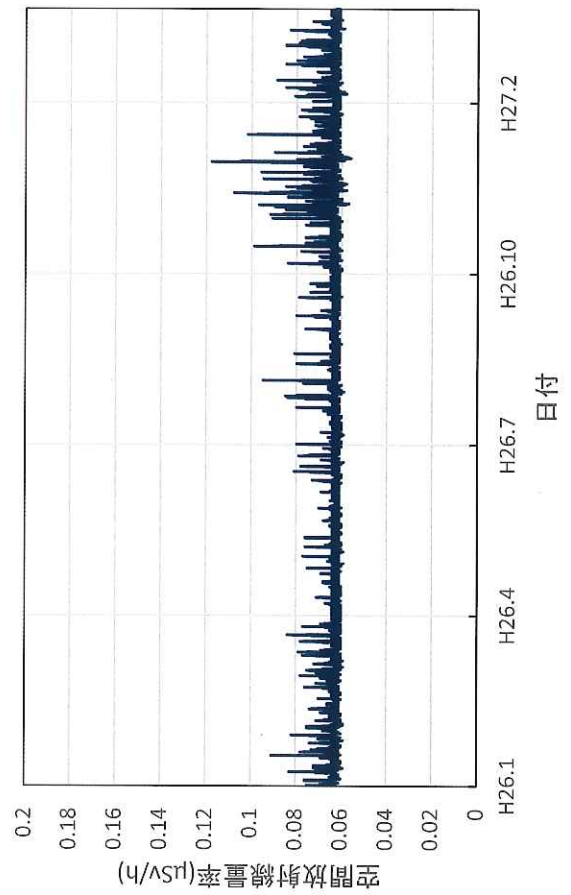
福井県あわら市 あわら市役所の空間放射線量率(10分値使用)
