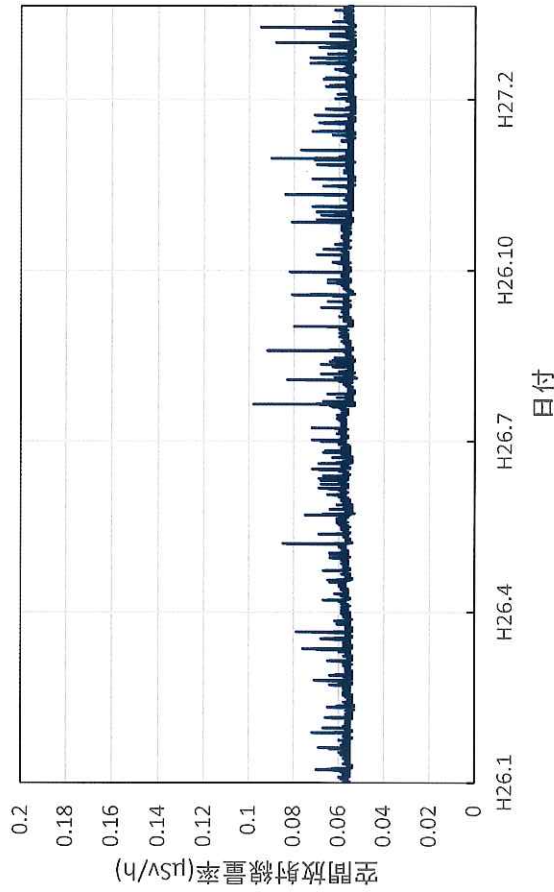
大阪府茨木市 茨木保健所の空間放射線量率(10分値使用)
