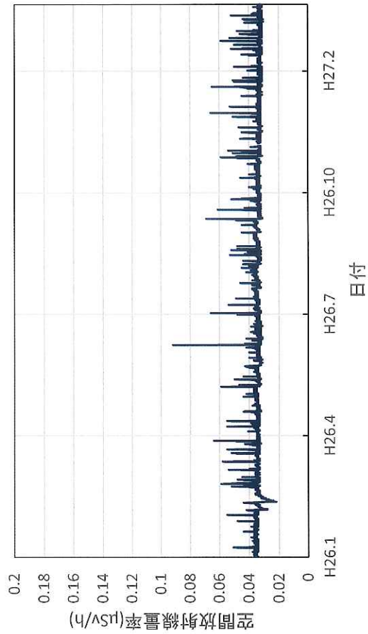
神奈川県海老名市 県産業技術センターの空間放射線量率(10分値使用)
