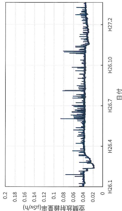
長野県軽井沢町 軽井沢町役場の空間放射線量率(10分値使用)
