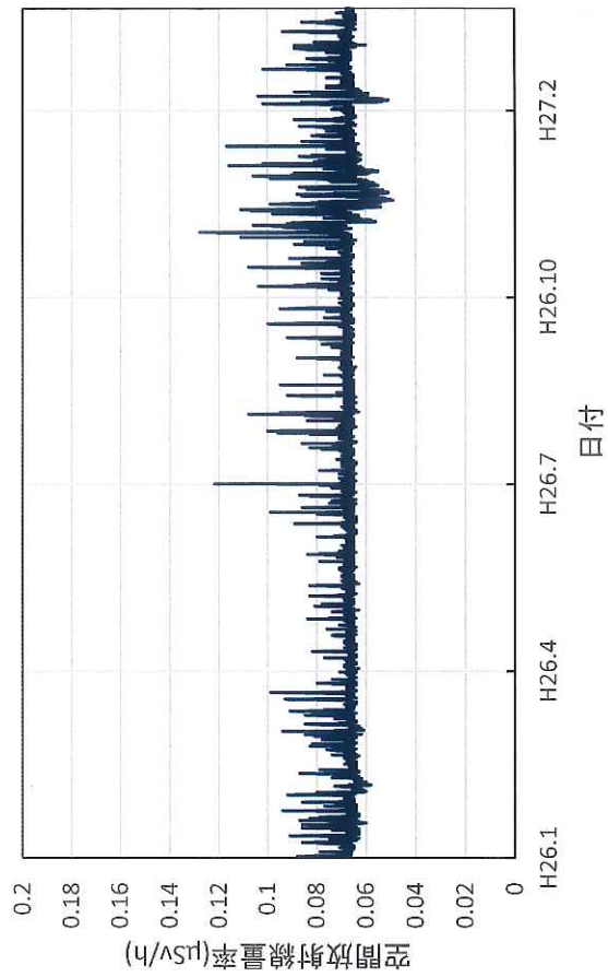
富山県砺波市 砺波総合庁舎の空間放射線量率(10分値使用)
