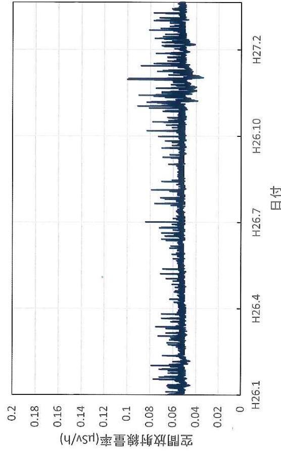
福井県鯖江市 鯖江市役所の空間放射線量率(10分値使用)
