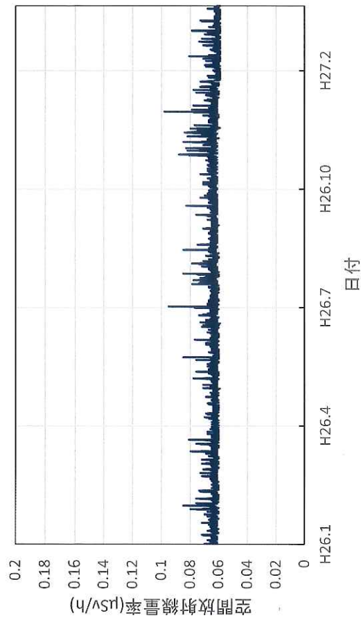
岐阜県各務原市 保健環境研究所の空間放射線量率(10分値使用)
