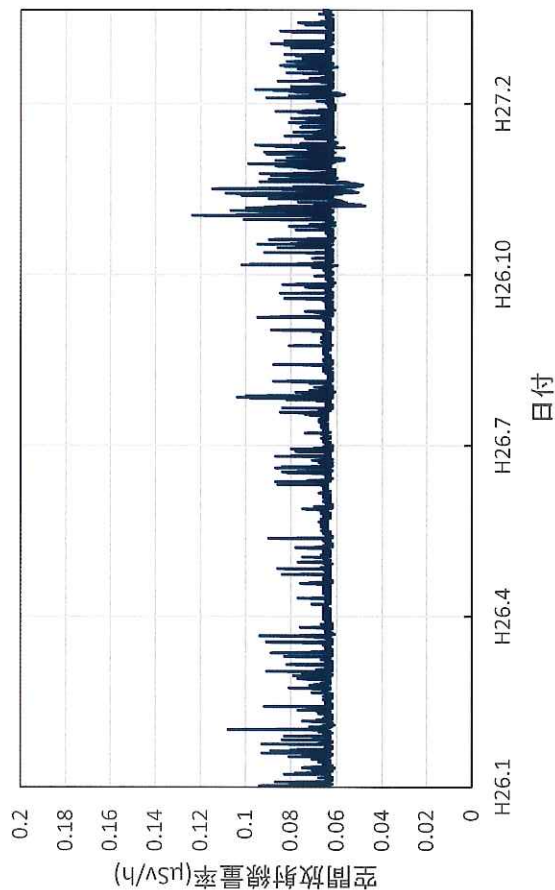
石川県羽咋市 余喜小学校の空間放射線量率(10分値使用)
