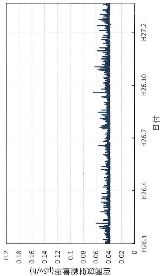
愛知県名古屋市長 環境調査センターの空間放射線量率(10分値 使用)
