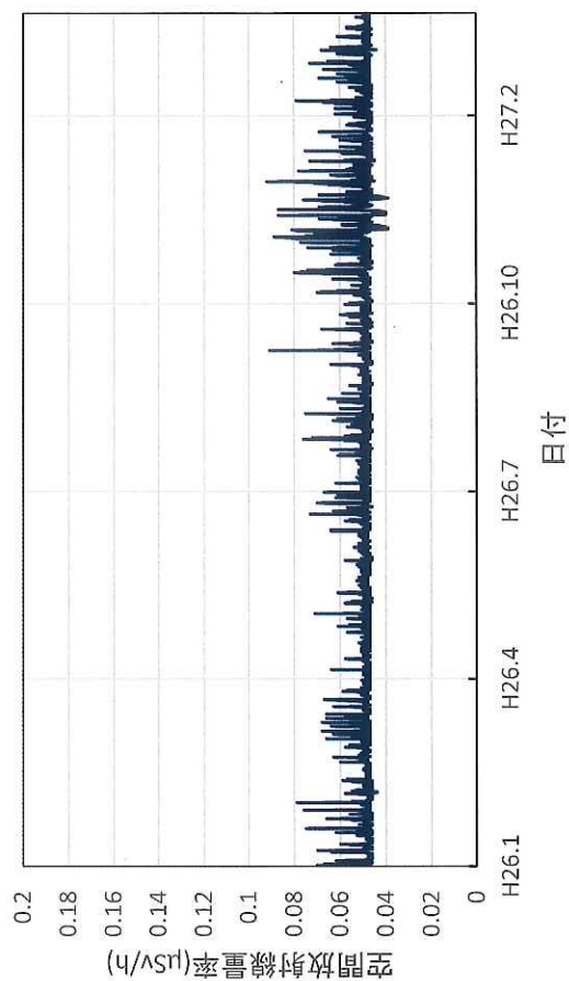
新潟県新潟市 放射線監視センター新潟分室の空間放射線量率 (10分値使用)
