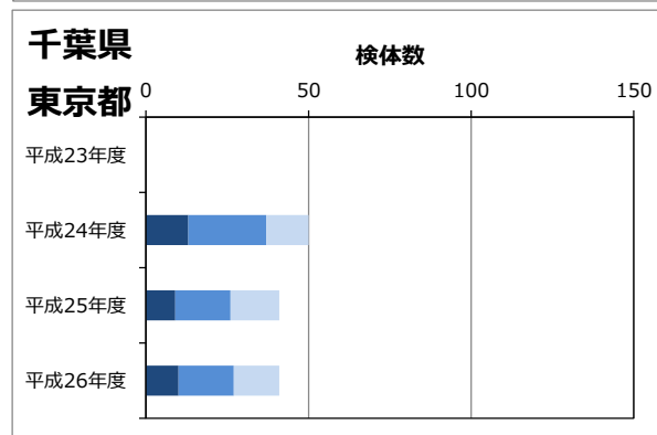
図 4.2-3 沿岸底質中の放射性セシウムを検出状況の推移（検体数が少ない自治体は割愛した）
