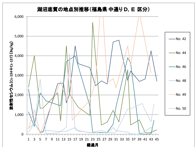
図 4.3-13 各地点の経年的な推移（福島県中通り：湖沼底質）
