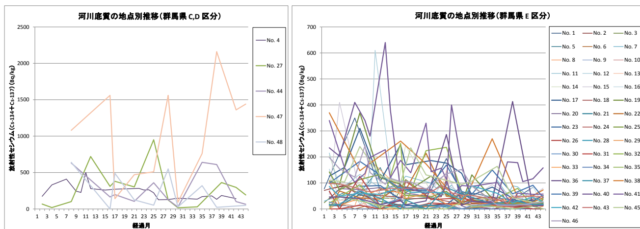
図 4.3-9 各地点の経年的な推移（群馬県：河川底質）
