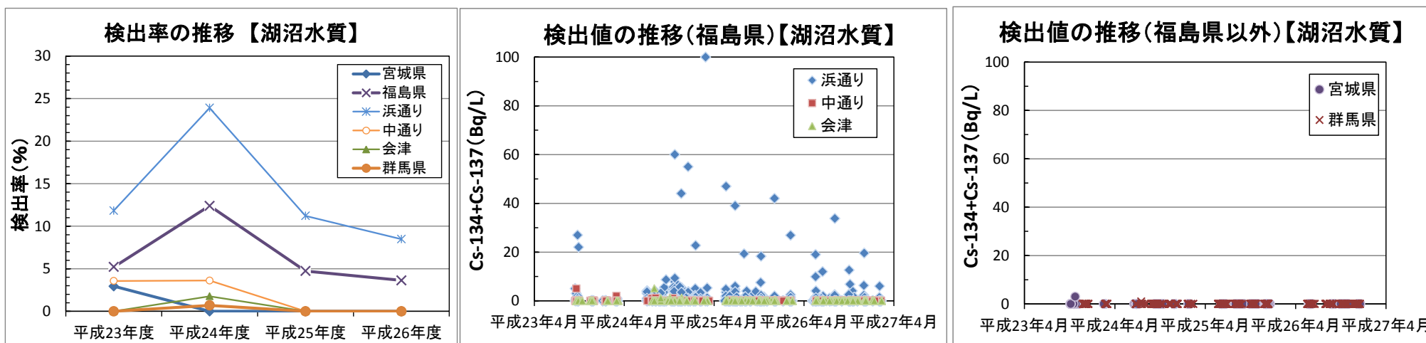
図 4.1-2 湖沼水質の放射性セシウムの「検出率 (左)」及び「検出値の推移 (中央及び右)」
