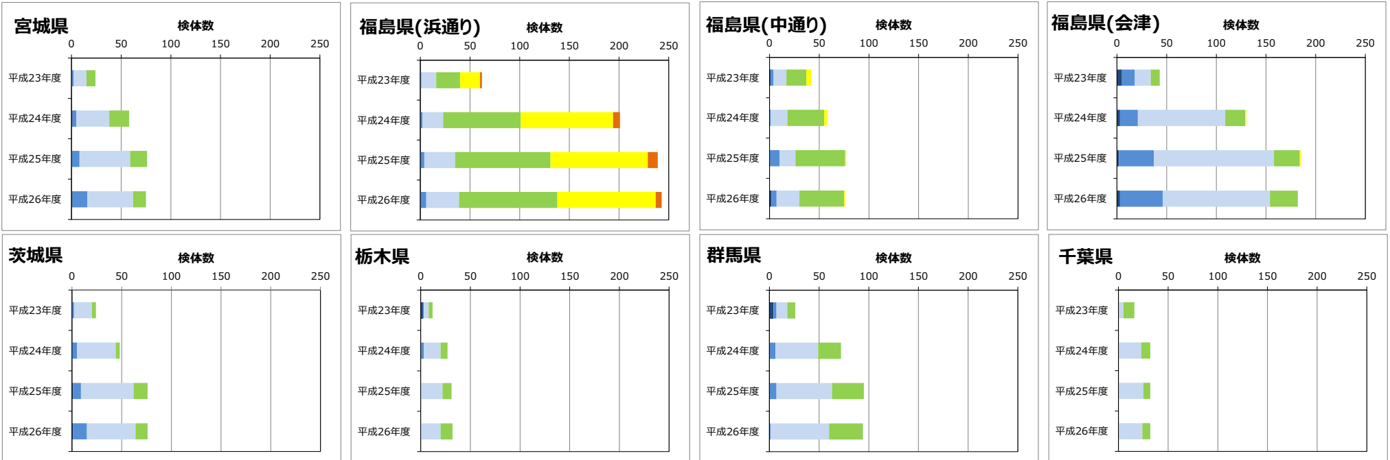
図 4.2-2 湖沼底質中の放射性セシウムの検出状況の推移（検体数が少ない自治体は割愛した）
