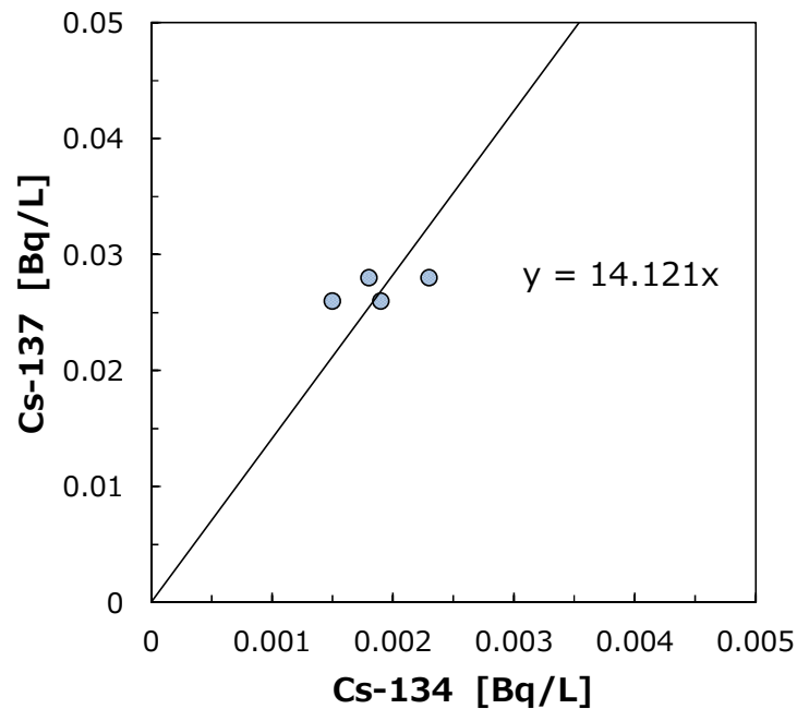
図 3.2-7 Cs-137/Cs-134 比の状況【水質 (公共用水域)】
