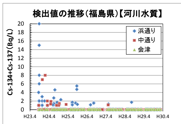
図 4. 1. 1-1 河川水質の放射性セシウムの「検出率の推移 (上)」及び「検出値の推移 (左下及び右下)」
