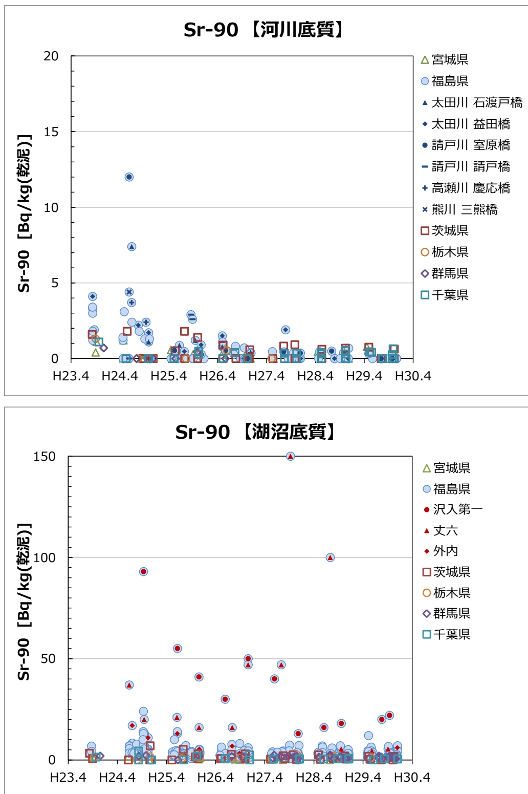
図 4. 2-1 公共用水域における底質中の Sr-90 の検出状況（上：河川、下：湖沼）
