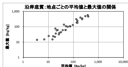
図 4.1.2-7 地点平均値の順位による区分の設定状況 (左: 設定のイメージ、右上: 区分整理結果 9 、右下: 地点平均値と最大値の関係)
